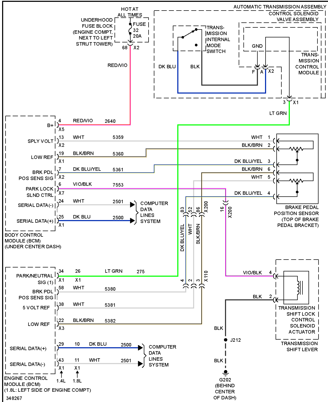
Fig. 67: Shift Interlock Circuit
