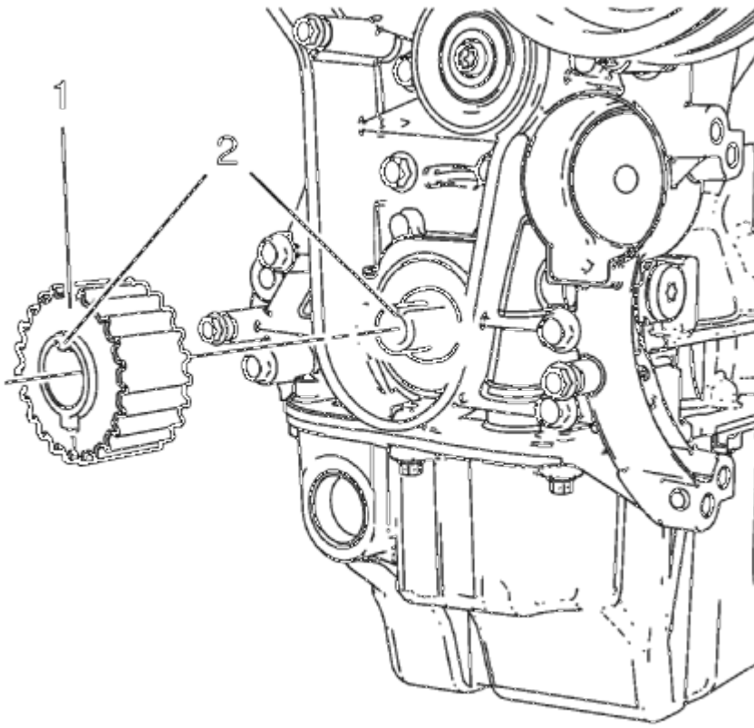
Fig. 365: Crankshaft Sprocket
