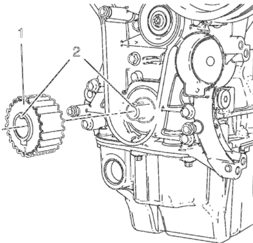
Fig. 176: Crankshaft Sprocket
