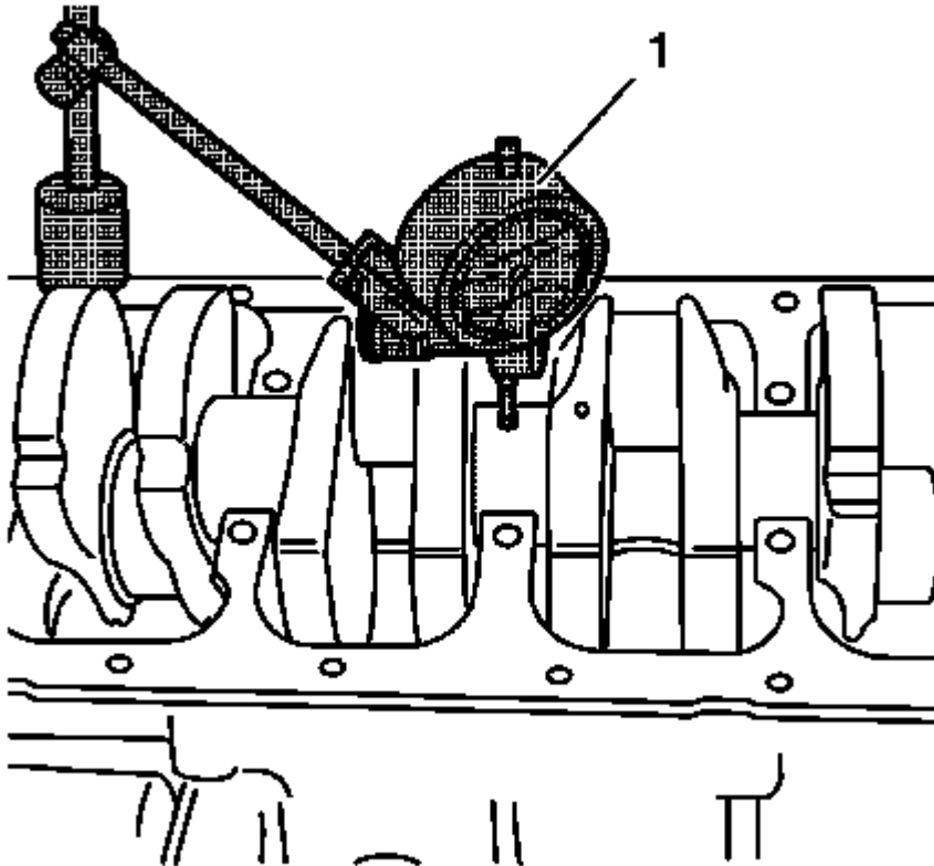
Fig. 440: Gauge Tool
