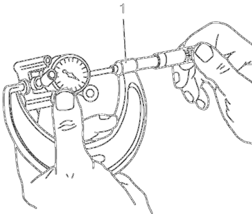
Fig. 443: Micrometer Gauge
