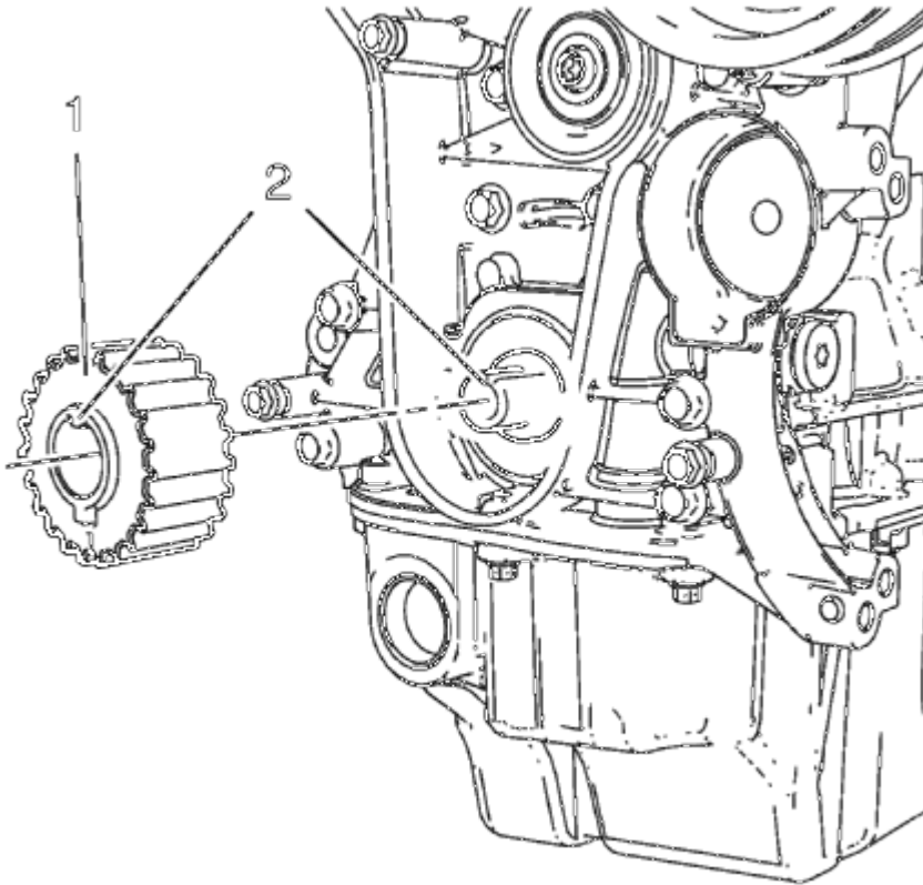
Fig. 511: Crankshaft Sprocket
