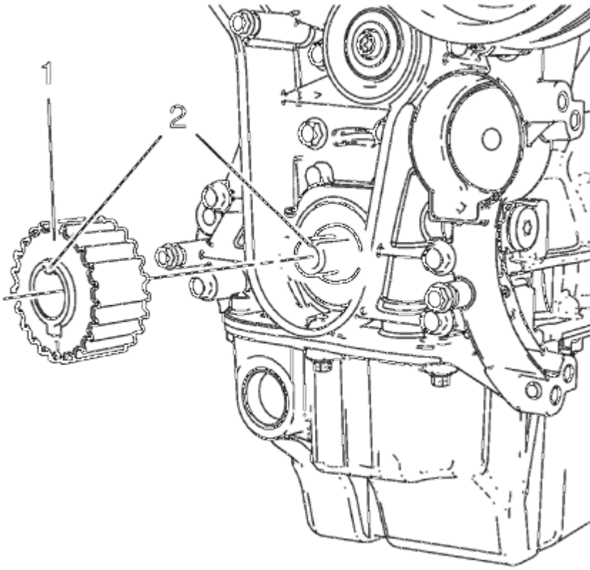
Fig. 180: Crankshaft Sprocket
