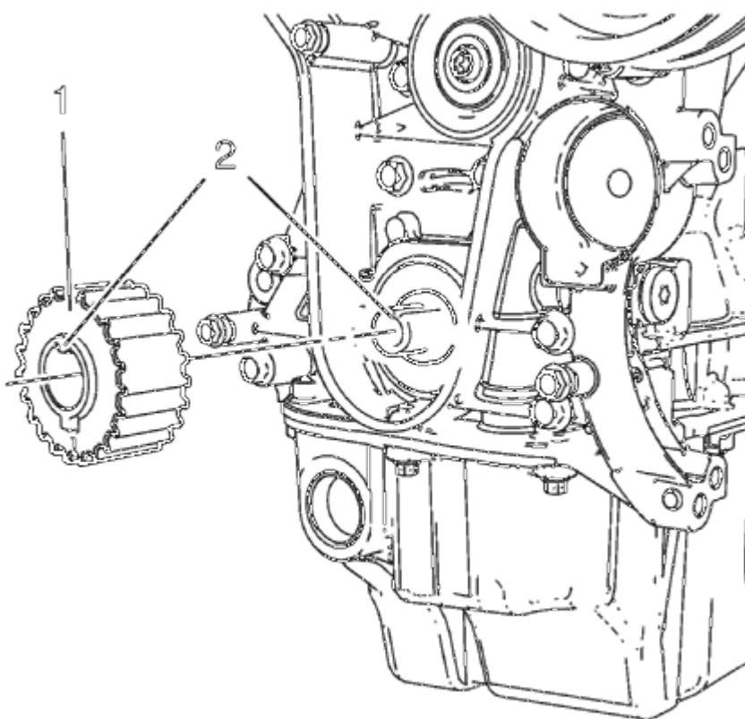
Fig. 275: Crankshaft Sprocket
