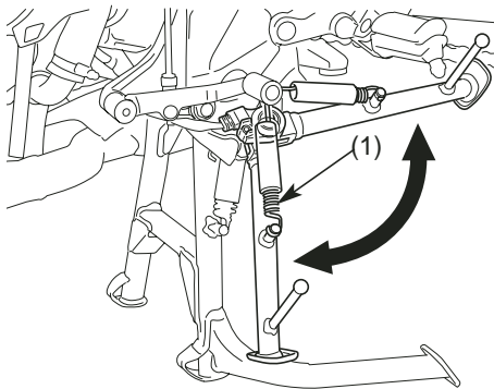
(1) Resorte
