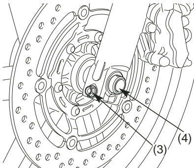
(3) Pernos de retención del eje (4) Eje delantero
