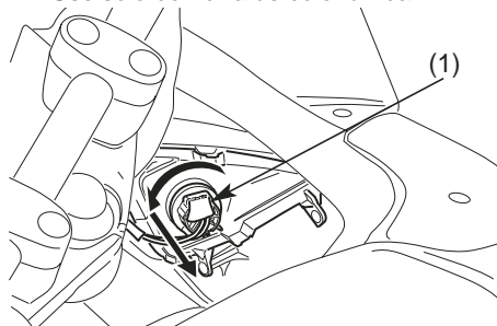
(1) Portalámparas
