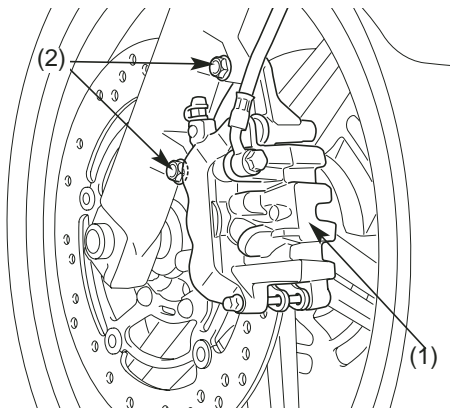
(1) Conjunto pinza de freno (2) Pernos de fijación
