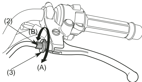
(2) Ajustador del cable del embrague
