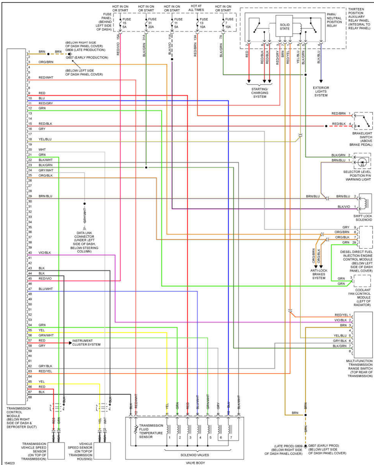
Fig. 71: 1.9L Turbo Diesel, A/T Circuit
