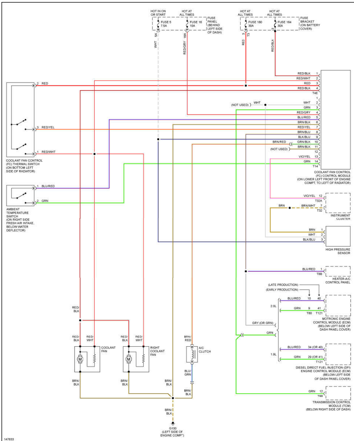
Fig. 14: 1.9L Turbo Diesel, Cooling Fan Circuit
