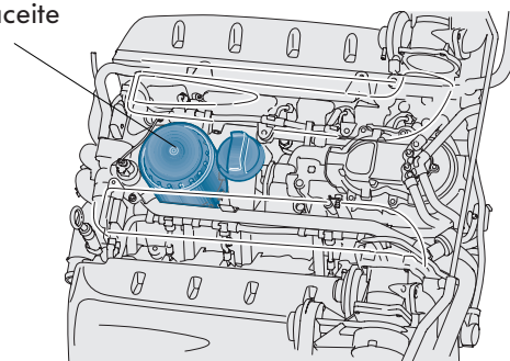
Módulo del filtro de aceite
