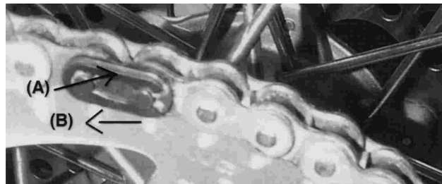
(A). Clip. (B). Dirección de la rotación de la cadena.
