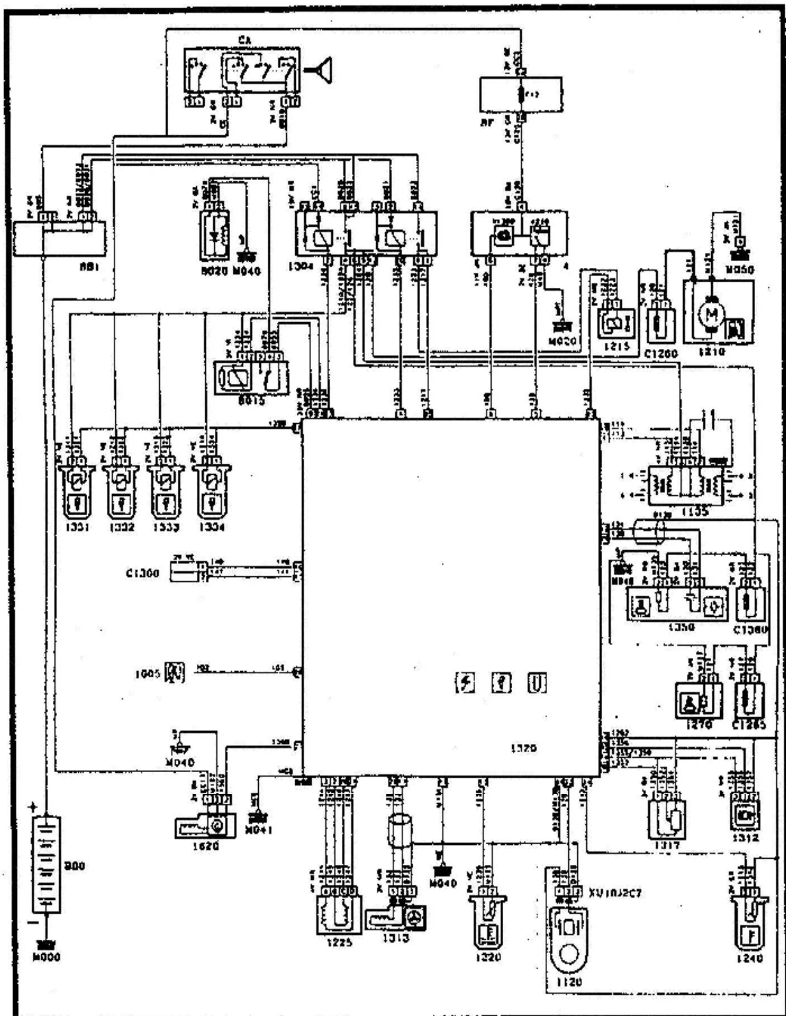
Fig. IV.16 Esquema de principio
