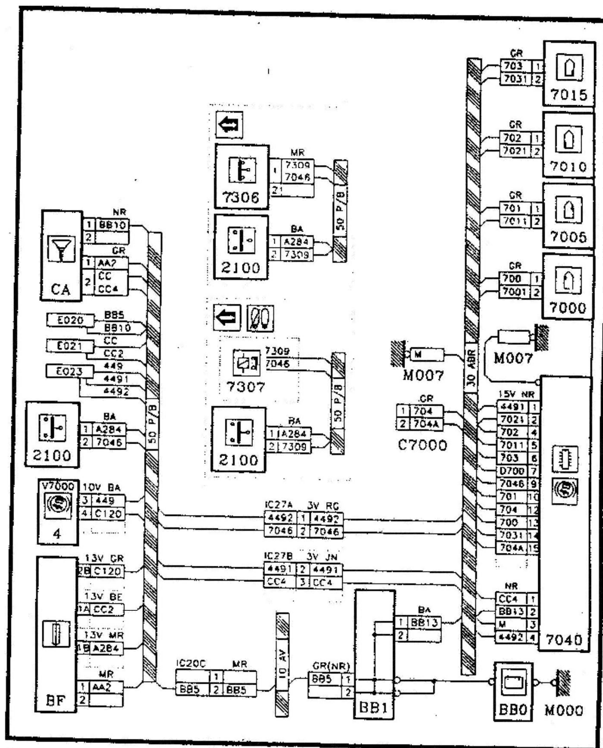
Fig. V.36 Esquema de cableado
