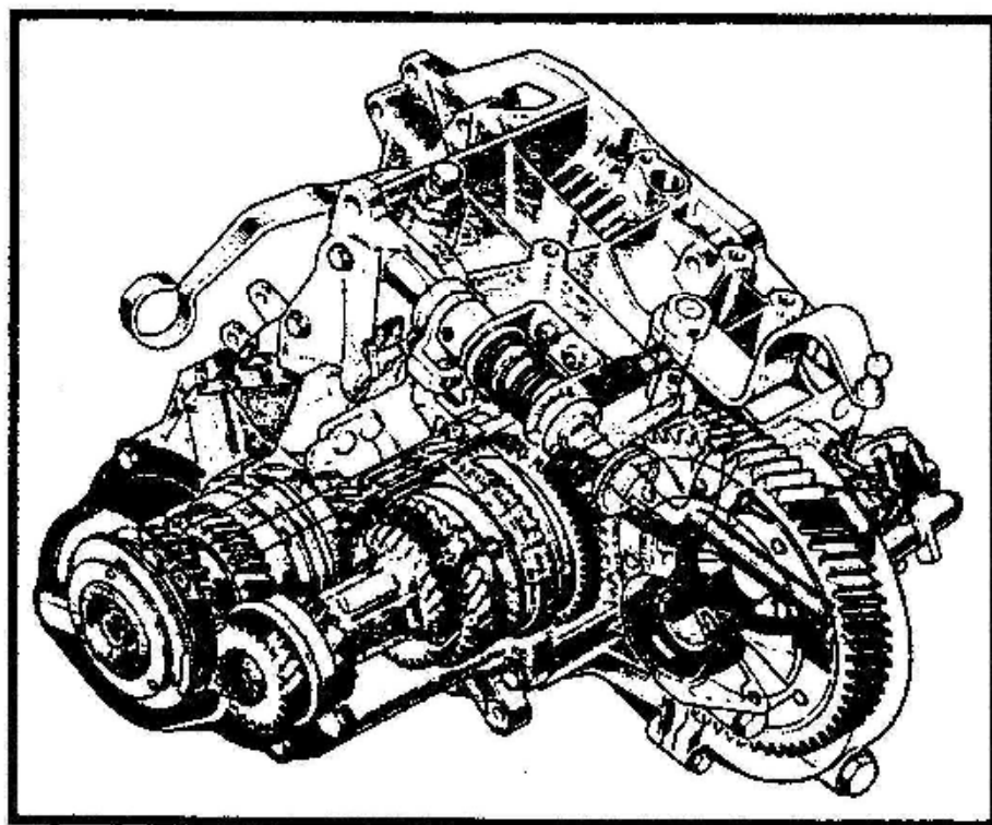
Fig. III.15 Caja de cambio BE3/5
