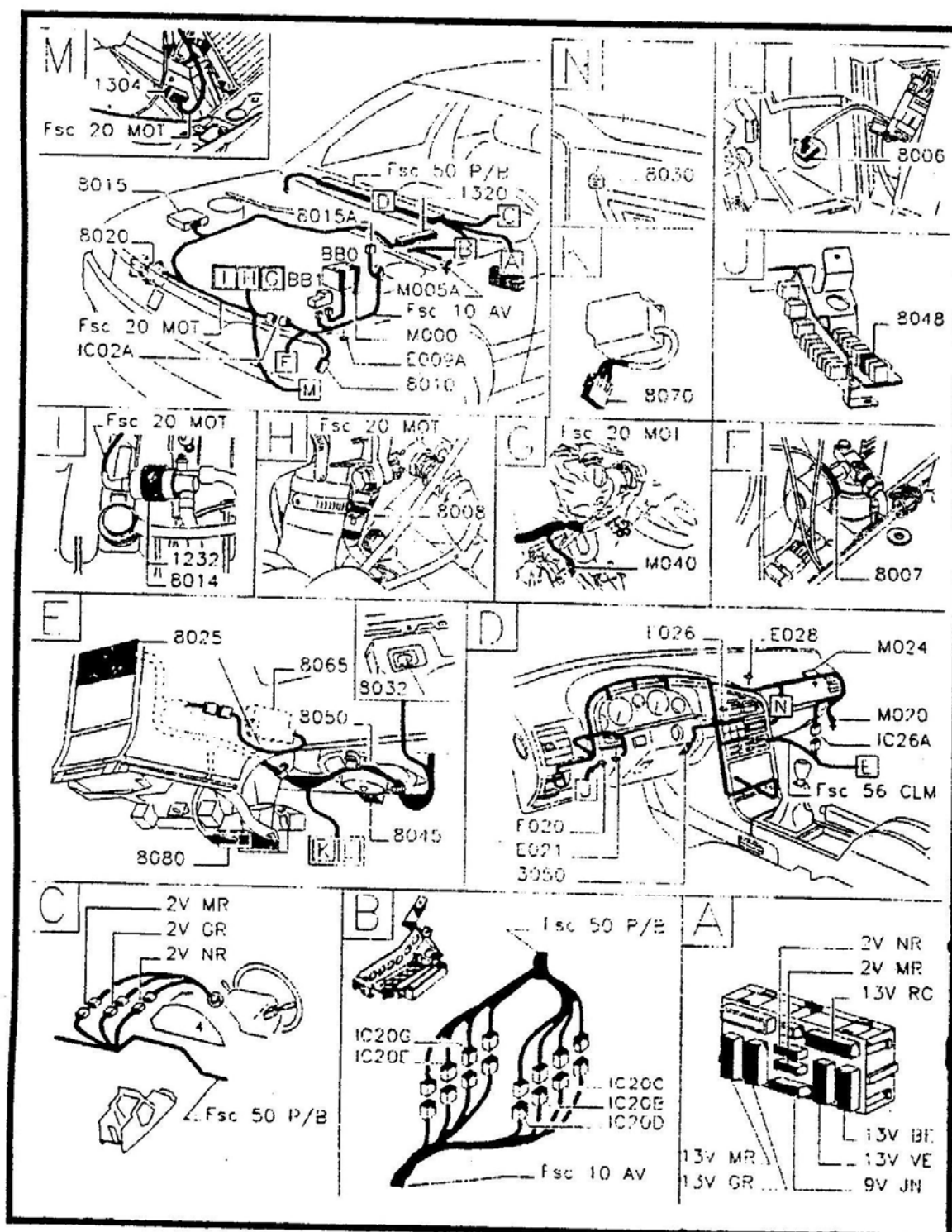
Fig. IX.2. Esquema de implantación
