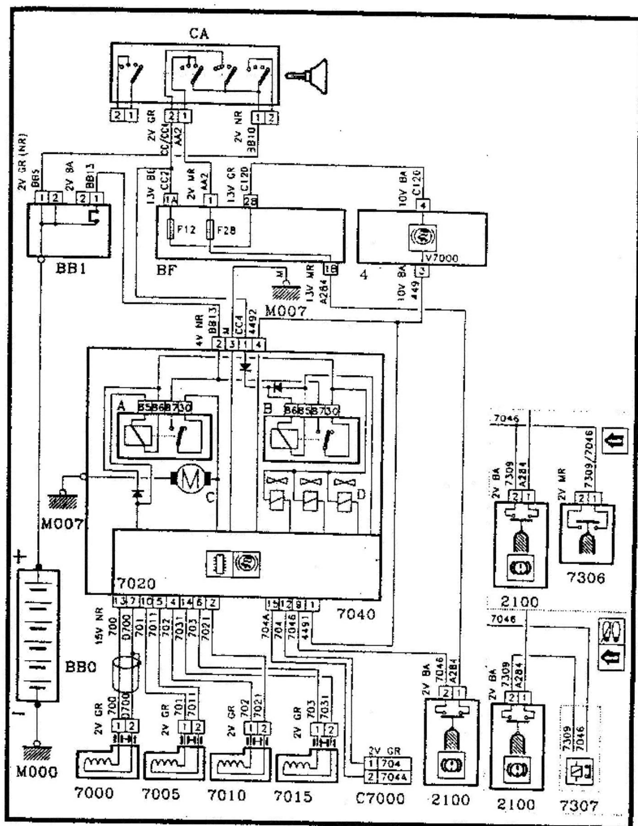
Fig. V.34 Esquema de principio
