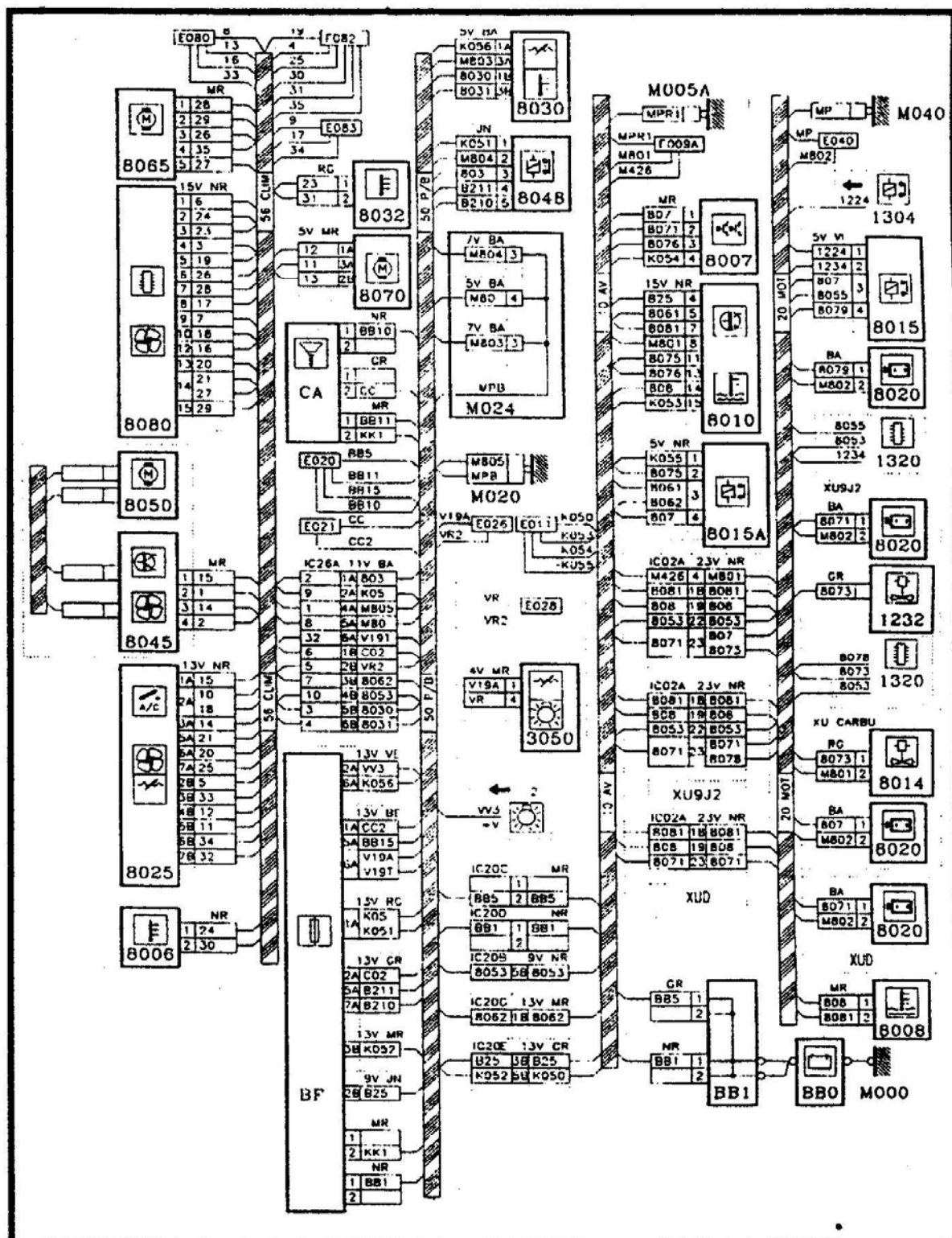
Fig. IX.3. Esquema de cableado
