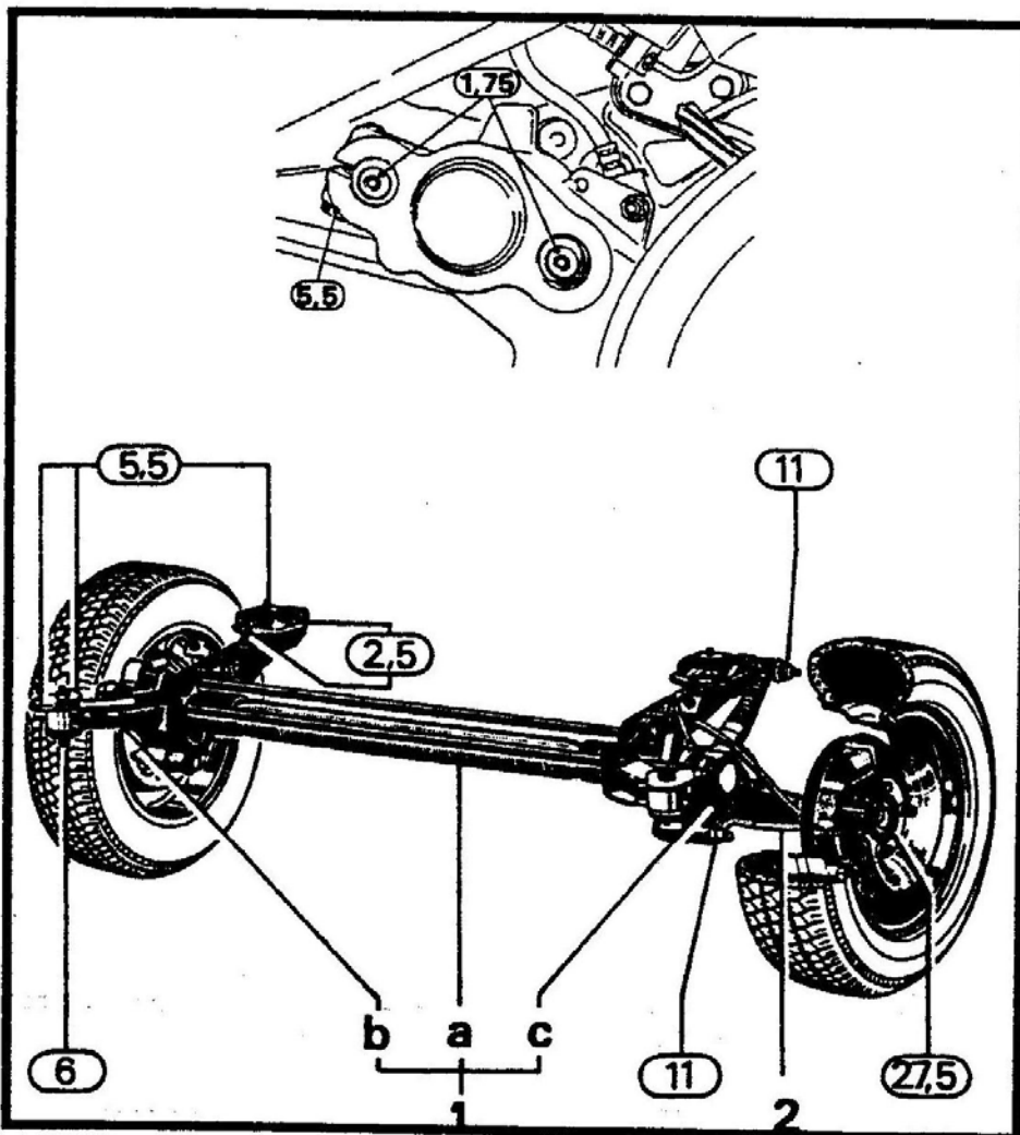
Fig. VI.17 Conjunto tren trasero con sus pares de aprietes en m.daN
