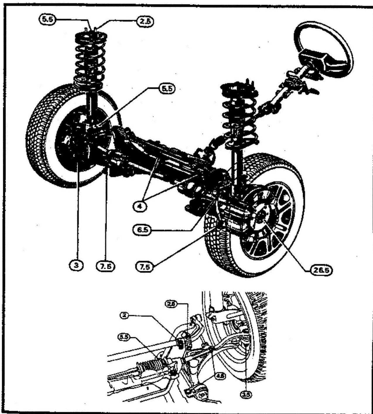
Fig. VI.1 Conjunto tren delantero con sus pares de aprietes en m.daN
