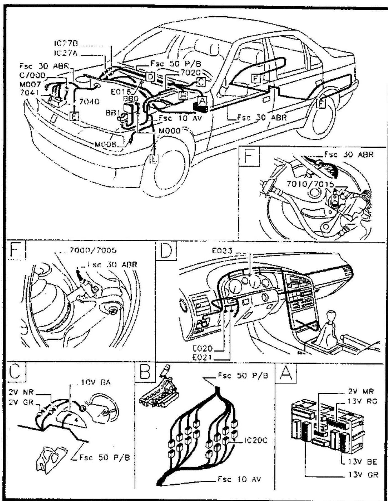
Fig. V.43 Esquema de implantación
