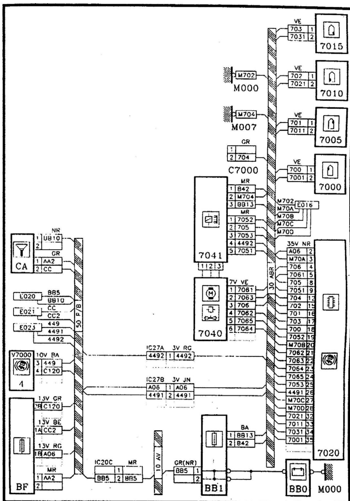
Fig. V.44 Esquema de cableado
