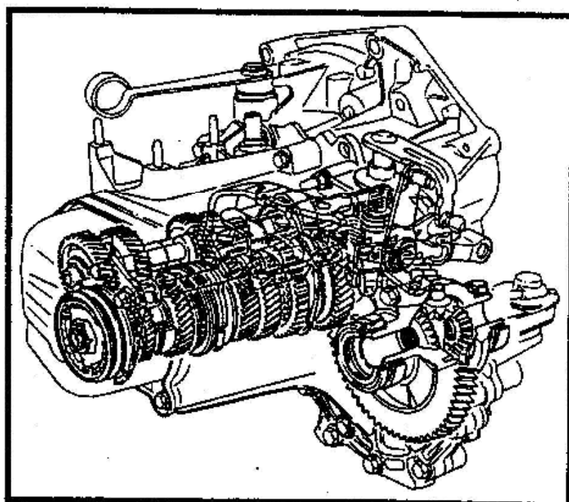
Fig. III.29 Caja de cambio MA-5
