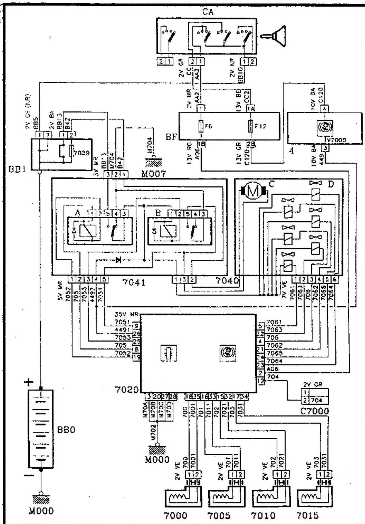
Fig. V.42 Esquema de principio
