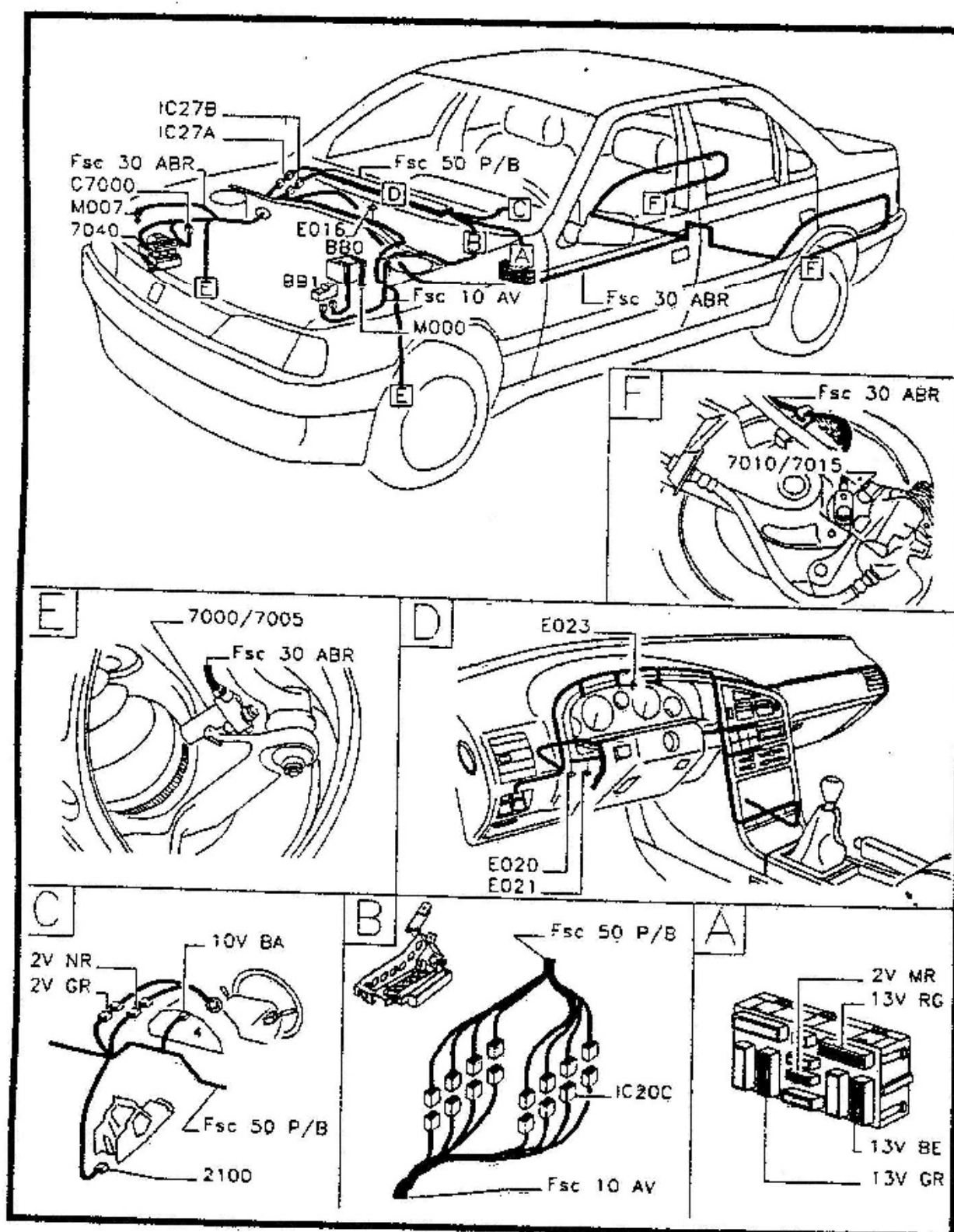
Fig. V.35 Esquema de implantación
