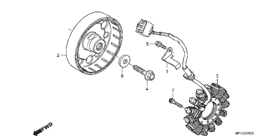
M-9 Gerador
