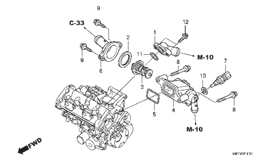
M-17 Termostato
