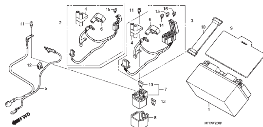
C-28 Bateria
