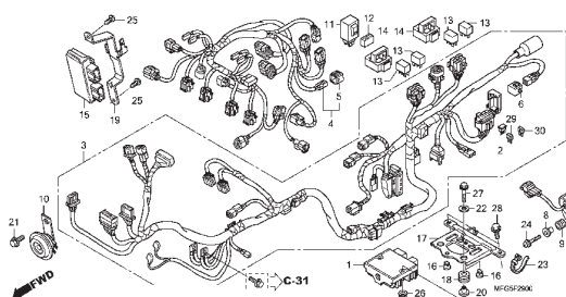
C-29 Fiação Principal
