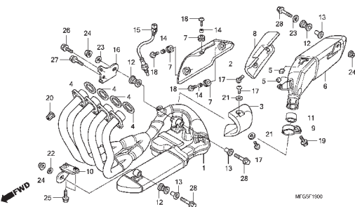
C-19 Escapamento
