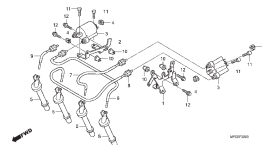
C-30 Bobina de Ignição
