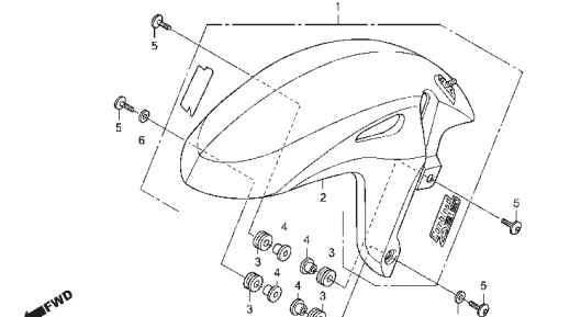
C-8 Pára-lama Dianteiro
