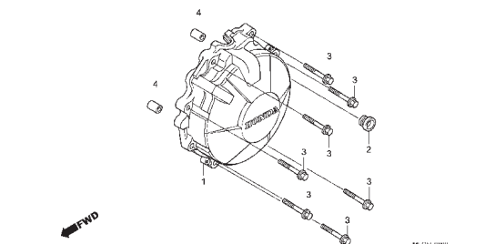
M-8 Tampa Lateral Esquerda
