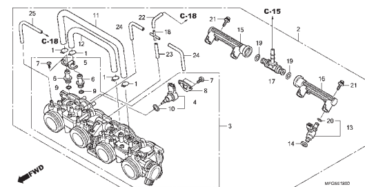
M-18 Carcaça do Acelerador
