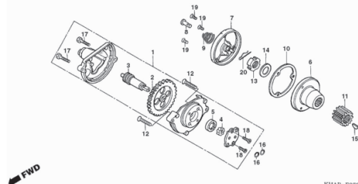
M-8.1 Cubierta Izquierda de la Carcasa del Motor (CTX200E)
