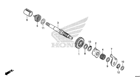
M-15 Arranque de Pie
