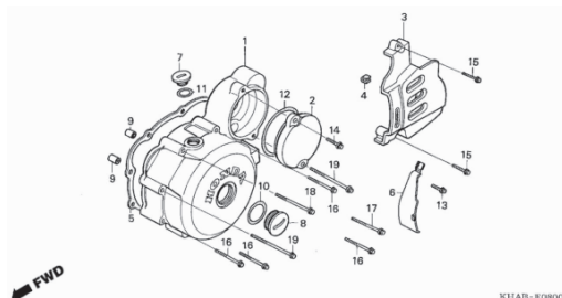
M-9.1 Generador (CTX200E)
