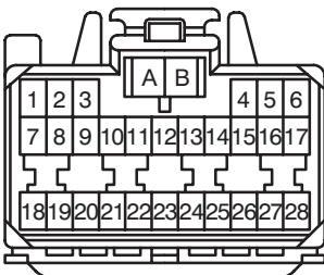
A36 Yellow
