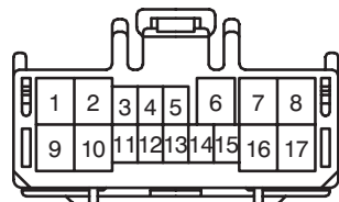
C14 (*7)
