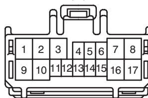
C14 (*6)
