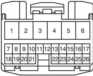
A28 Black
