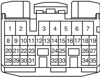
E12 (1GR-FE, 2TR-FE)
