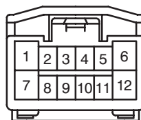
P11 (*9)
