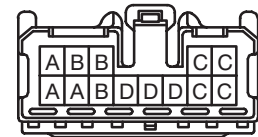
J10 (1KZ-TE)
