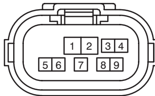
N 1 (*20) Gray
