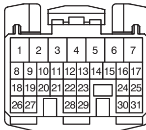
E10 (1GR-FE, 2TR-FE)
