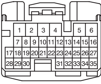
E18 Black
