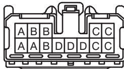
J10 (1GR-FE) Blue
