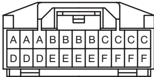
J20 (RHD General) Gray
