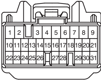
E12 (1KZ-TE)
