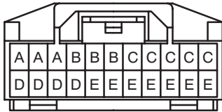
J19 (*15) Black
