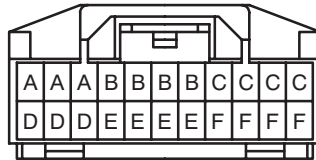
J21 (*18) Black
