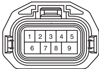
N 1 (1KZ-TE) Gray
