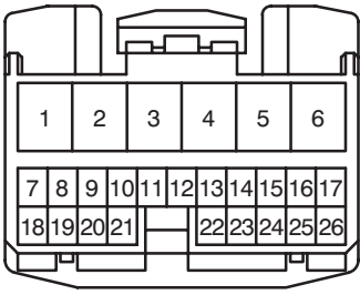
F 5 Gray
