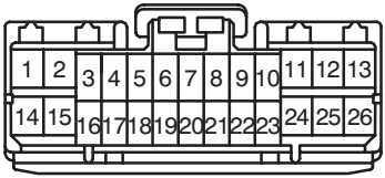
E12 (5L-E)
