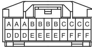
J19 (*16) Gray
