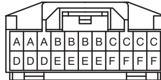
J11 (1KZ-TE)
