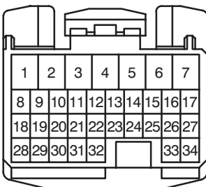
E11 (1GR-FE, 2TR-FE)
