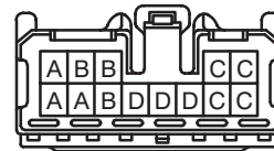
J23 (RHD) Blue
