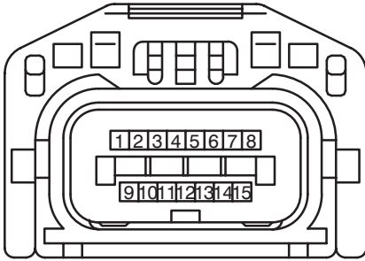
E 1 (*1) Gray
