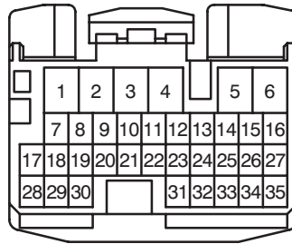
E 9 (1GR-FE, 2TR-FE)
