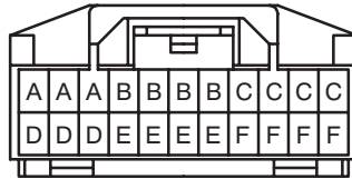
J18 (*15) Black
