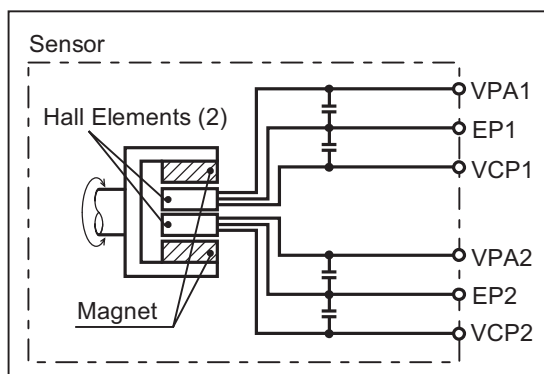
&lt; Wiring Diagram &gt;
