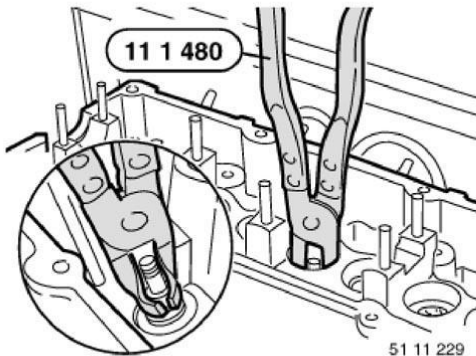
Fig. 258: Special Tool (11 1 480)
