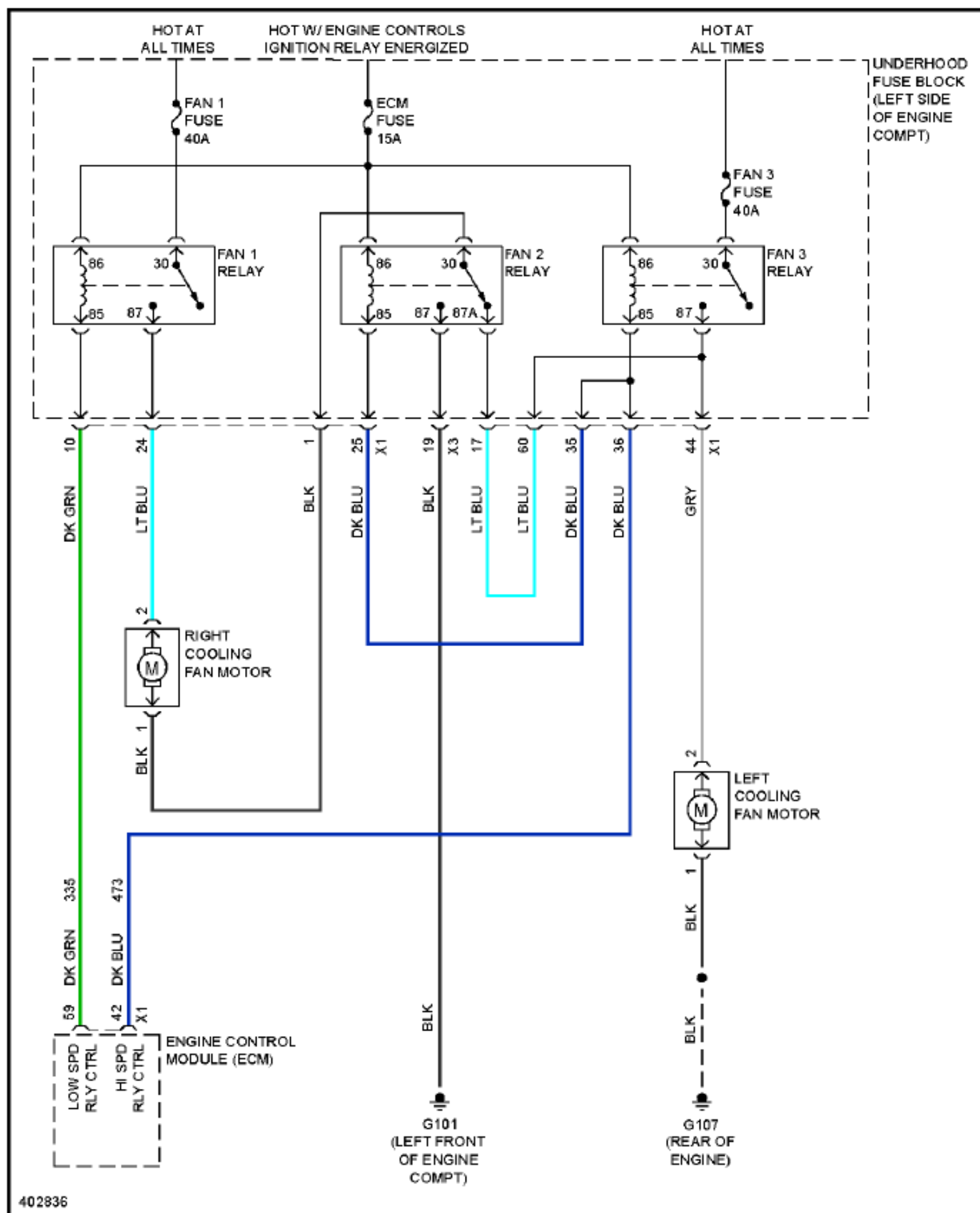
Fig. 15: 3.0L VIN 5, Cooling Fan Circuit
