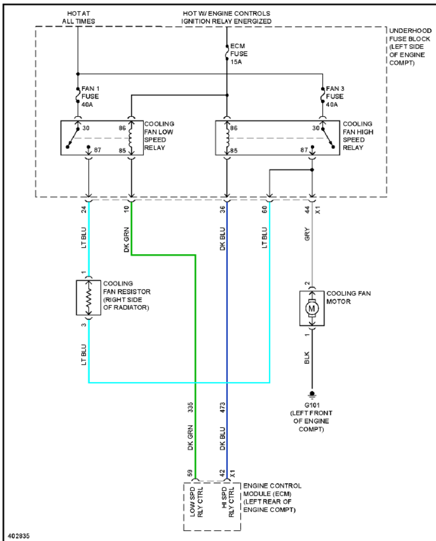
Fig. 14: 2.4L VIN K, Cooling Fan Circuit
