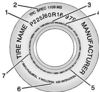
Ejemplo de llanta para vehículos de pasajeros (P-Métrico)
