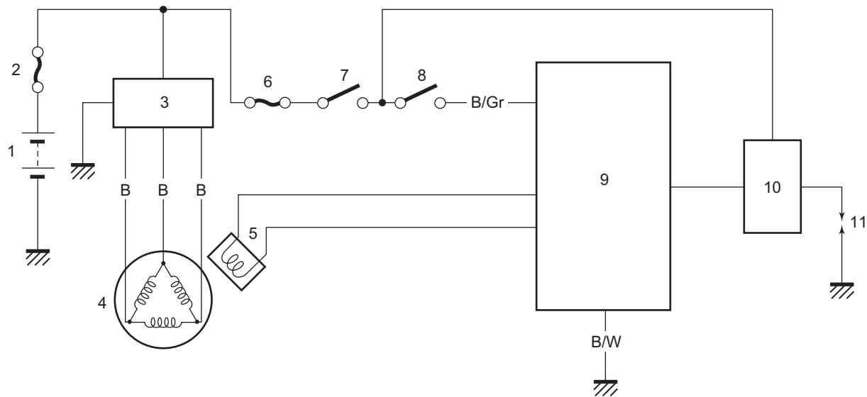
Diagrama del sistema de encendido
