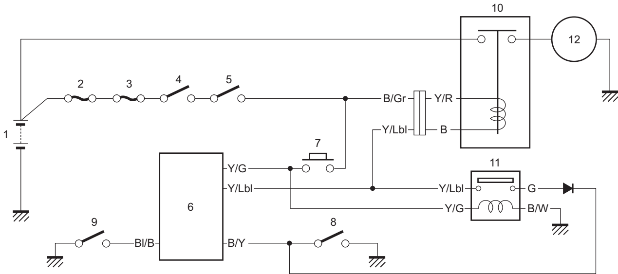
Diagrama del Sistema de Arranque
