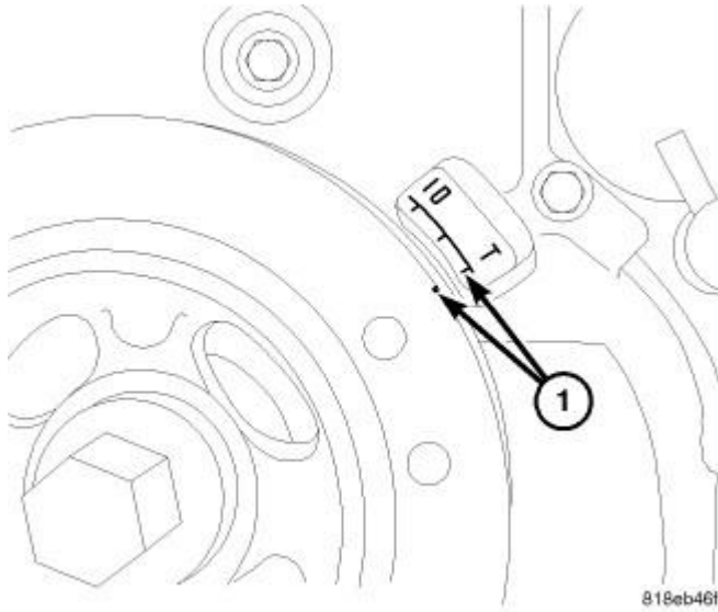
Fig. 418: TDC
