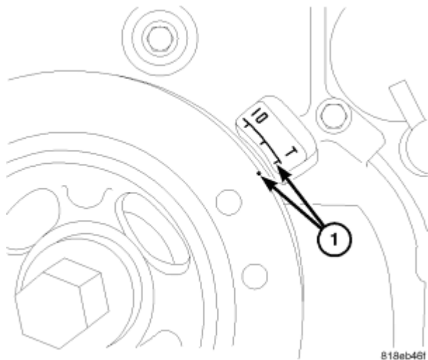
Fig. 127: TDC
