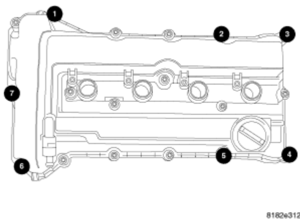
Fig. 155: Stud Location
