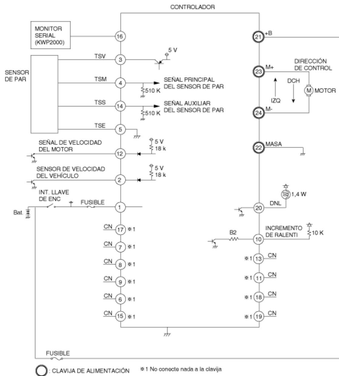
DIAGRAMA DE CONEXIONES
