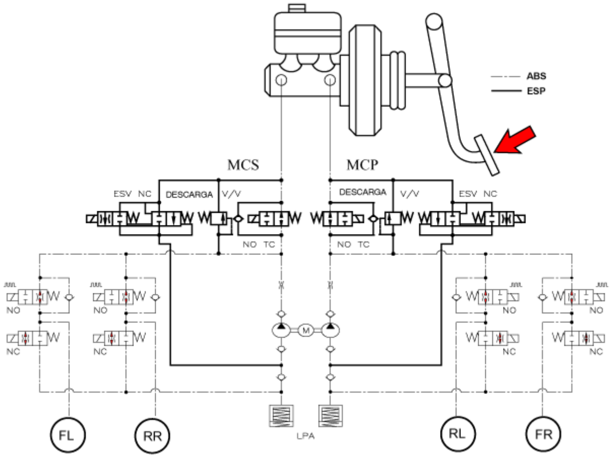
DIAGRAMA DEL SISTEMA HIDRÁULICO ESP
