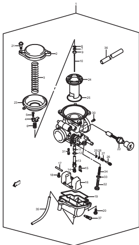
FIG.9 (B-10) CARBURETOR
