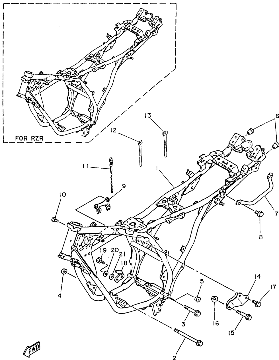
FIG. 15 FRAME
