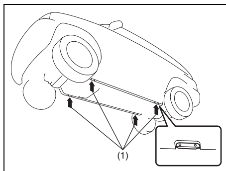
(1) Punto de elevación con el gato
