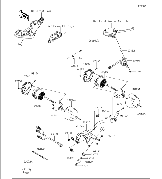
70 Accessory(Sub Lamp)
