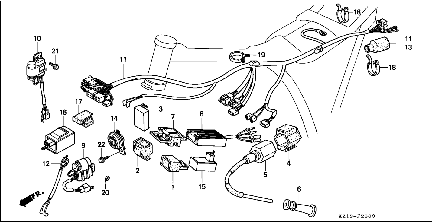
Bloque F-26 CONJUNTO DE ALAMBRES/ BOBINA DE ENCENDIDO/UNIDAD DE C.D.I.
