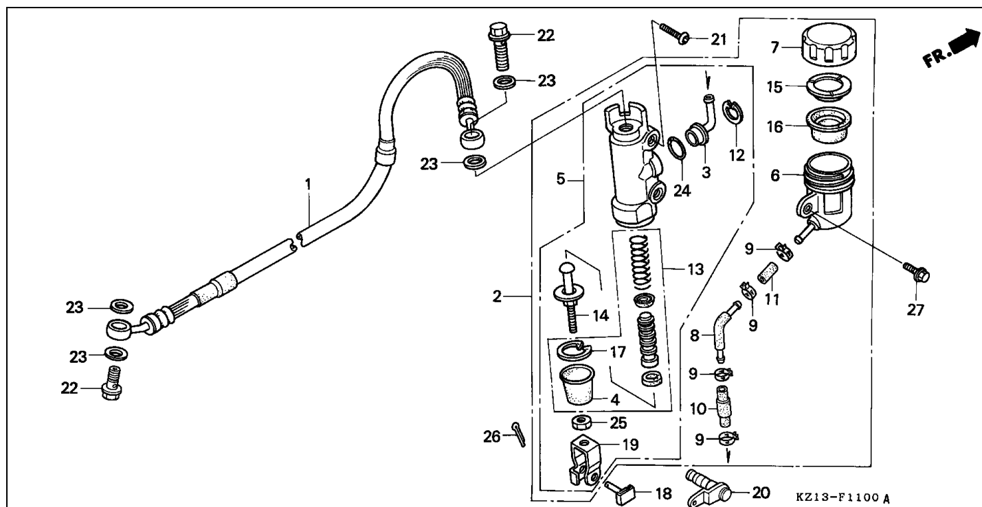
Bloque F-11 MAESTRO DE FRENO TRASERO CILINDRO
