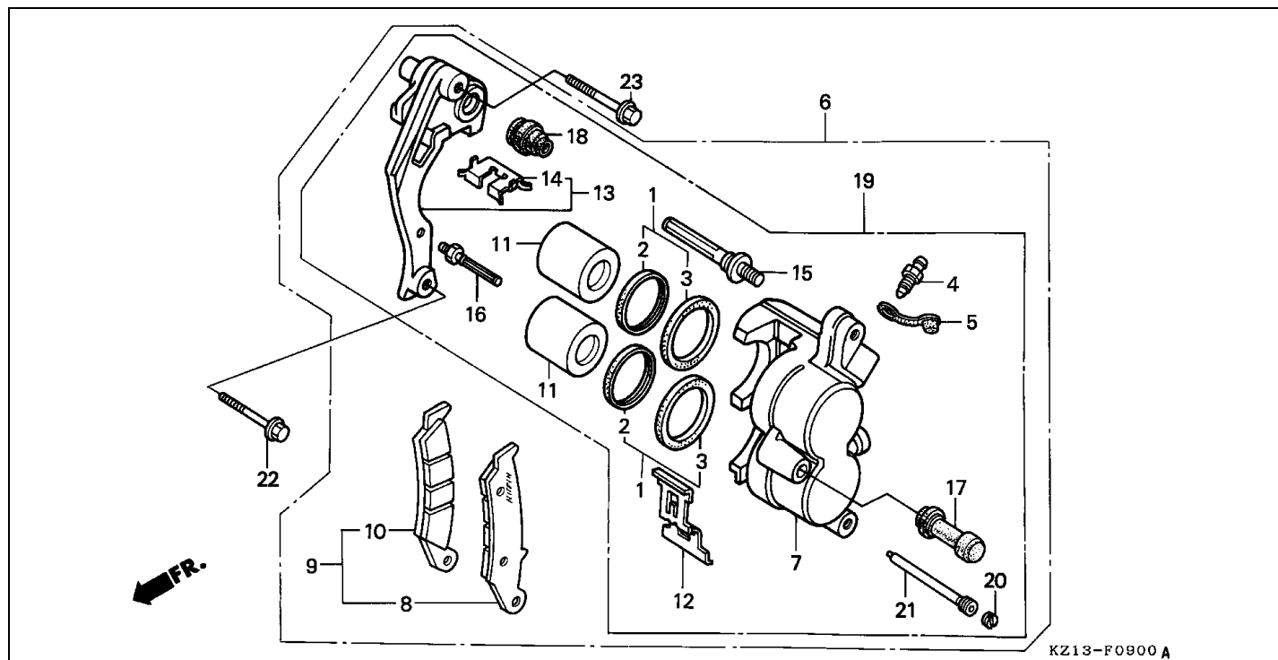
Bloque F-9 CALIBRE DE FRENO
