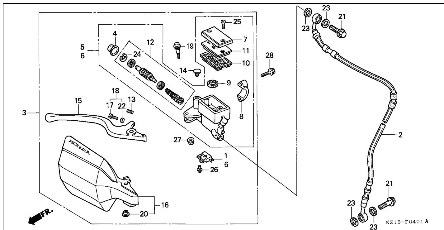
Bloque F-4-1 CILINDRO MAESTRO DE FRENO(RP/RR)
