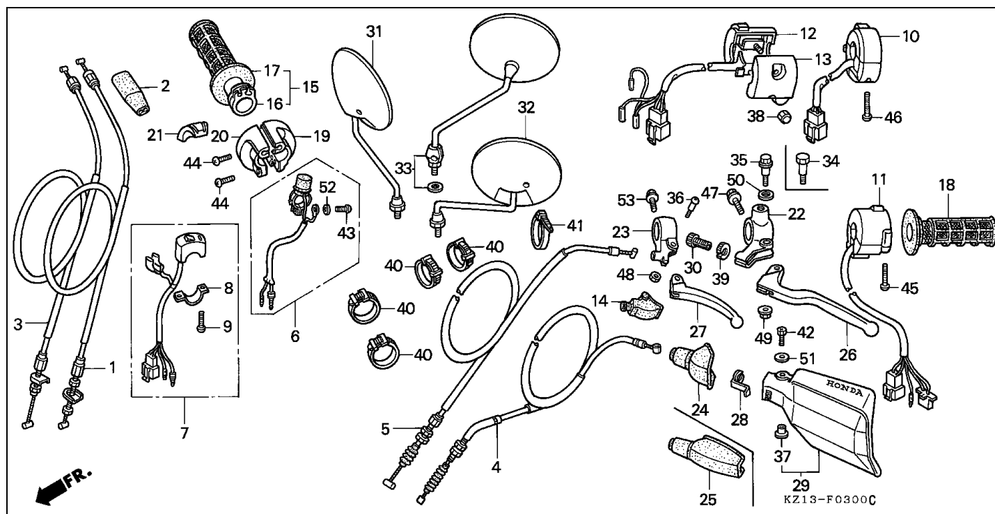
Bloque F-3 PALANCA DE MANIJA/INTERRUPTOR/ CABLE(B/DK/ED/U)
