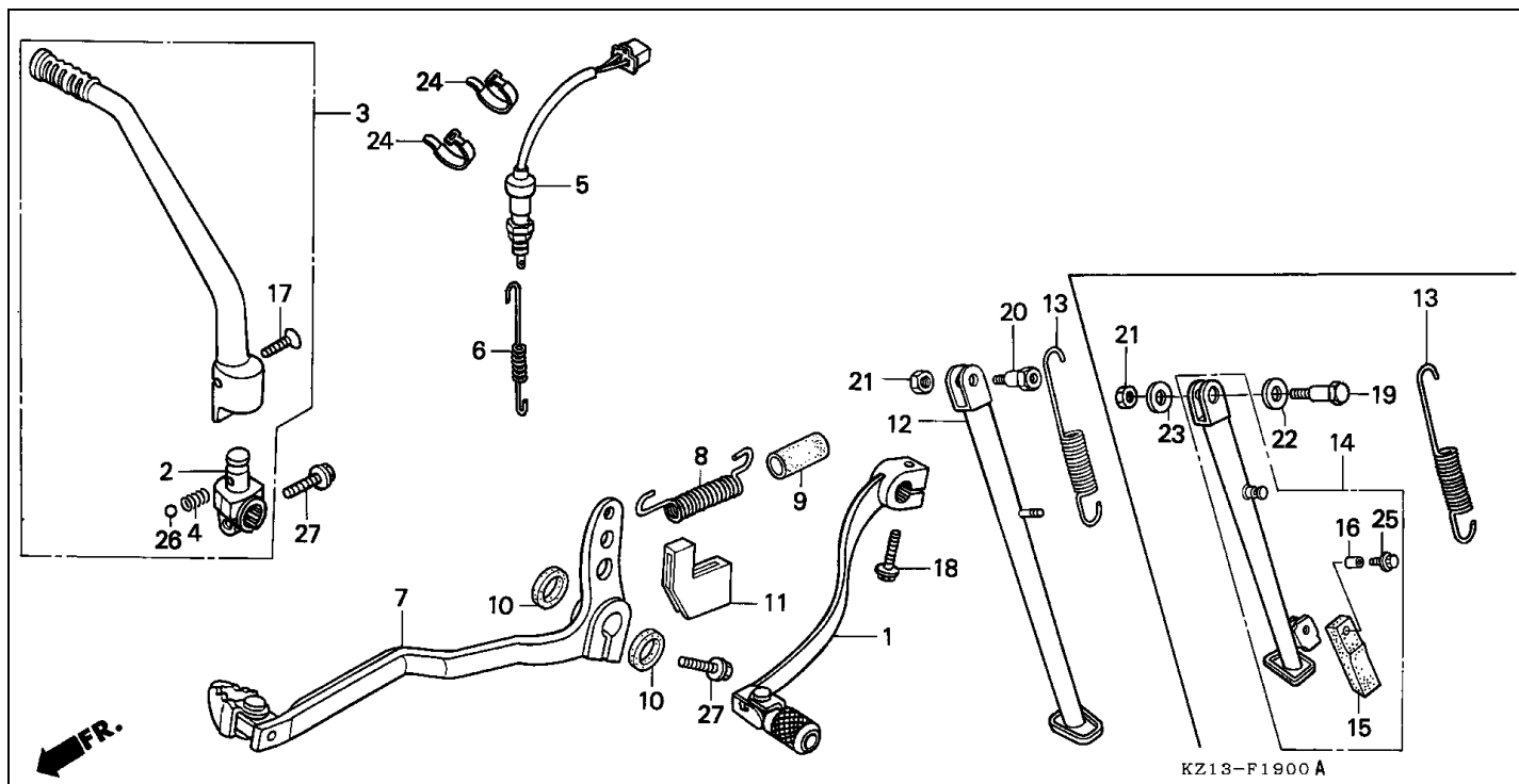
Bloque F-19 PEDAL/BRAZO ARRANCADOR PEDAL
