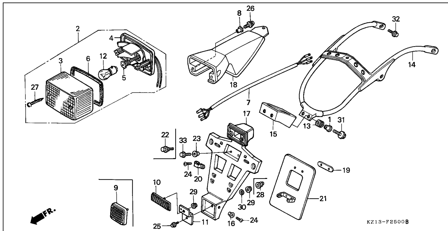
Bloque F-25 LUZ TRASERA (B/DK/ED/U)
