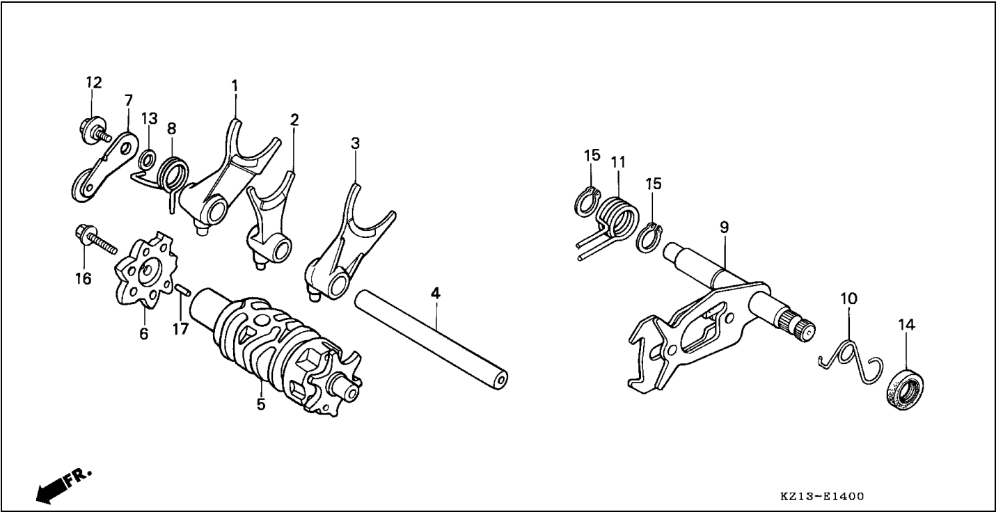
Bloque E-14 TAMBOR CAMBIO ENGRANAJES
