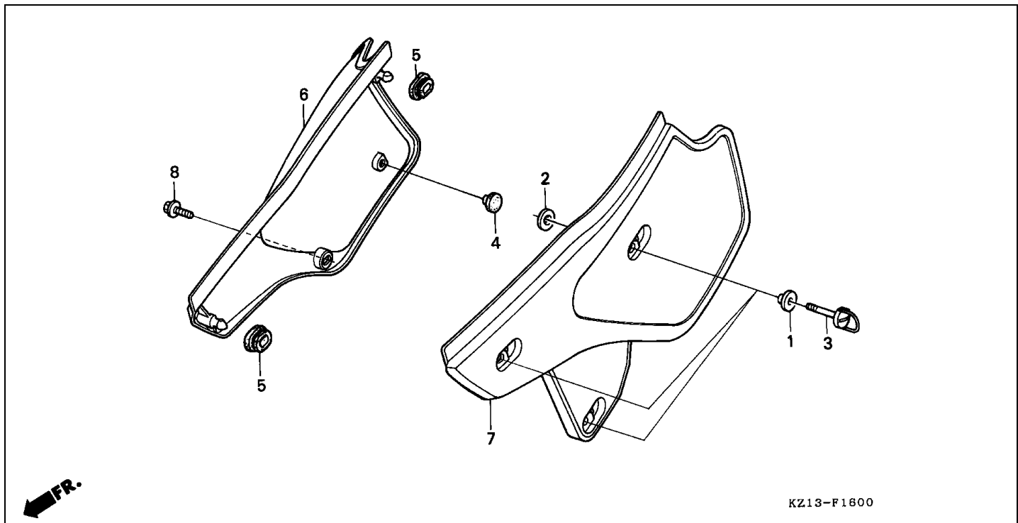
Bloque F-16 CUBIERTA LATERAL
