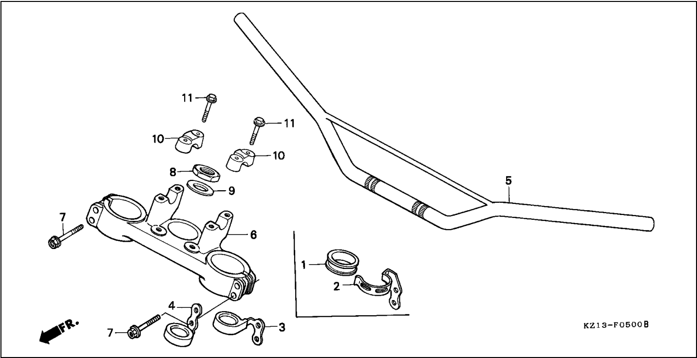
Bloque F-5 TUBERIA DE MANIJA/PUENTE SUPERIOR
