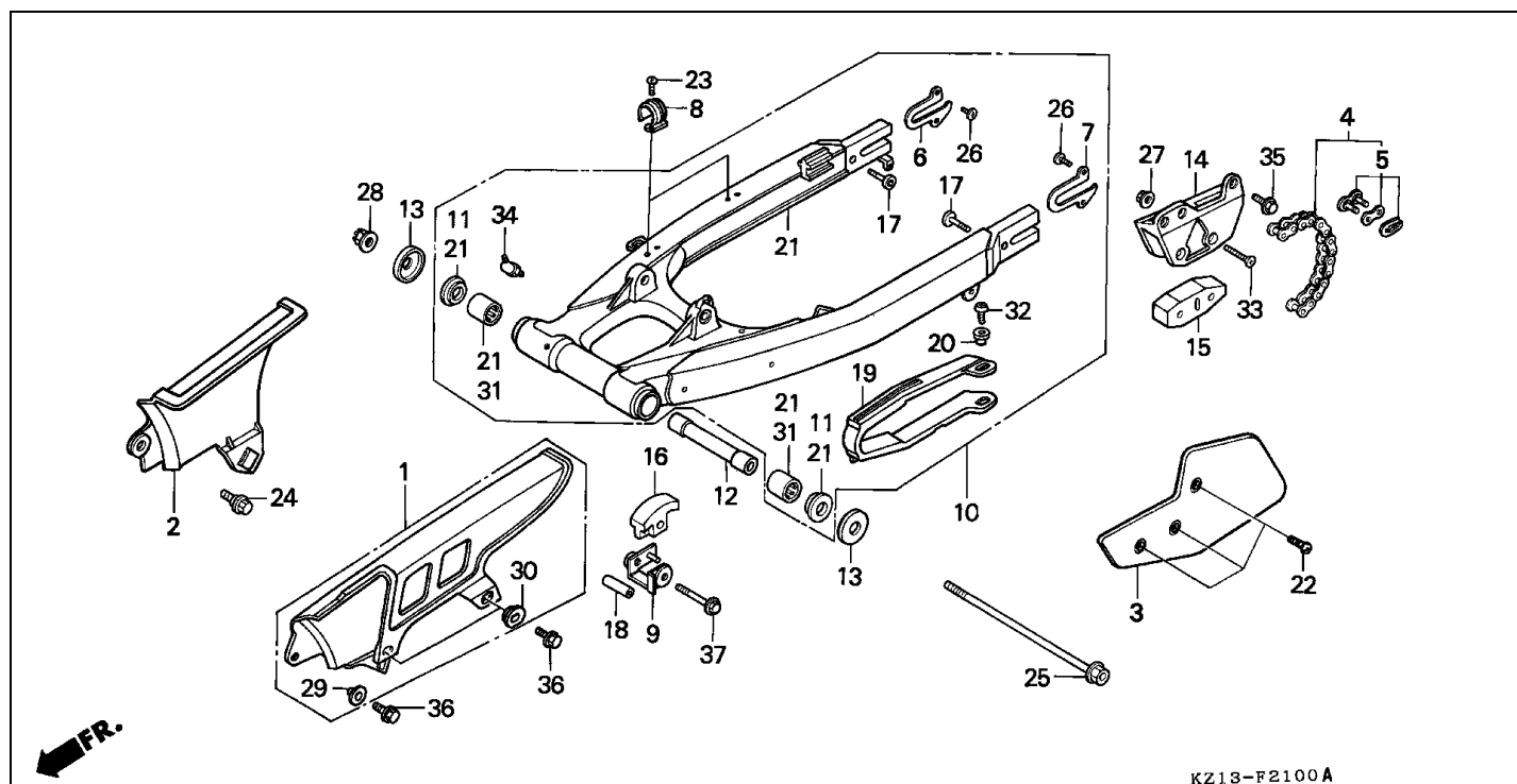
Bloque F-21 BRAZO DE OSCILACION/CAJA DE CADENA
