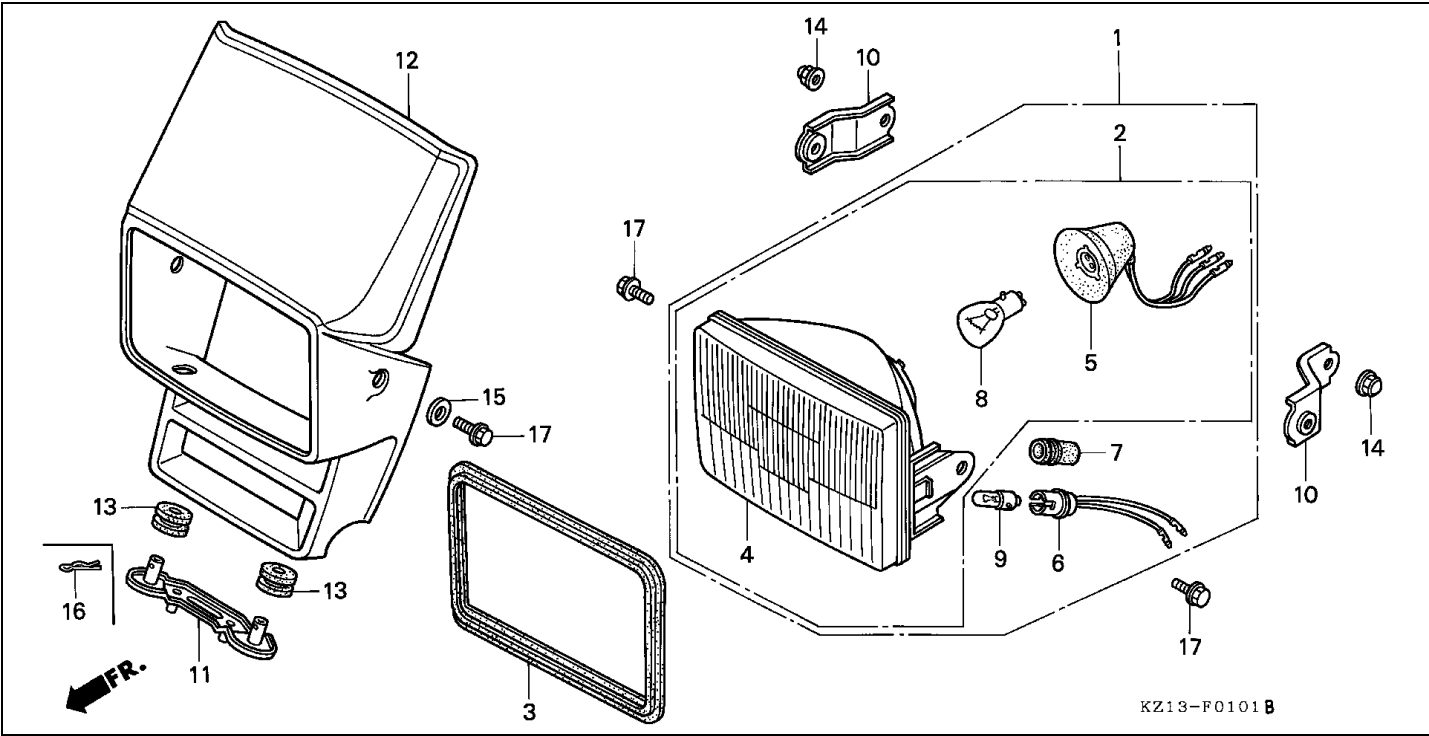
Bloque F-1-1 FARO DELANTERO (B/ED/U)
