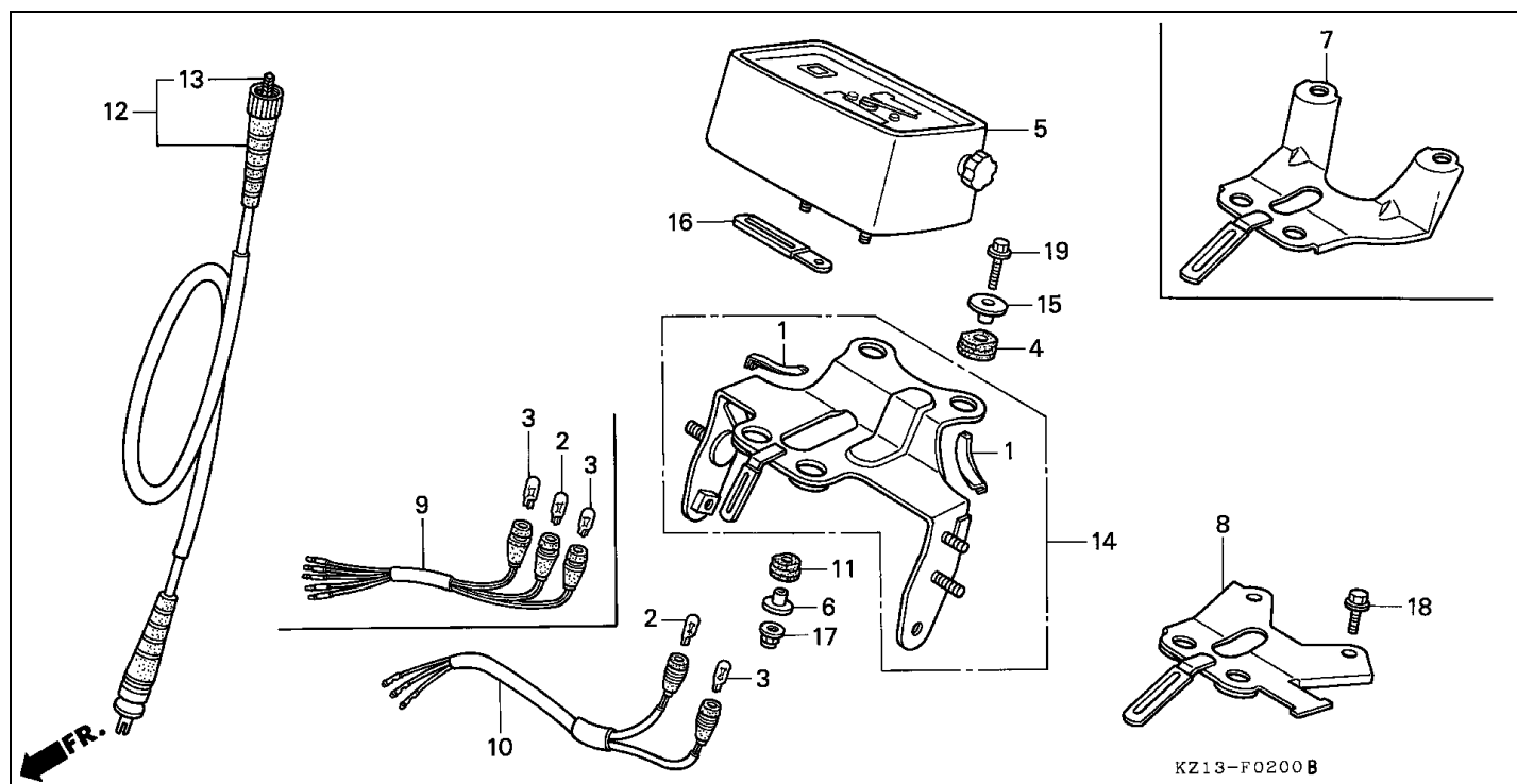
Bloque F-2 VELOCIMETRO (B/DK/ED/U)
