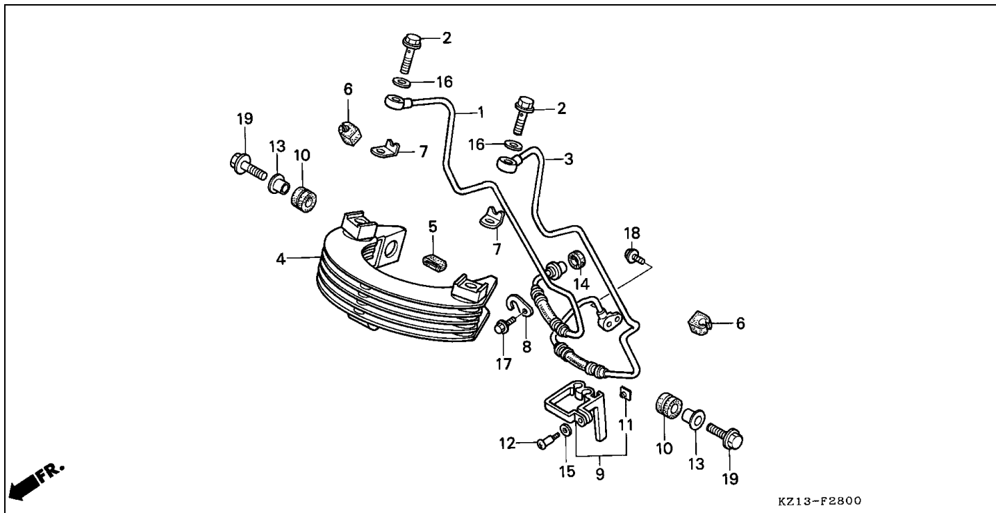
Bloque F-28 ENFRIADOR DE ACEITE
