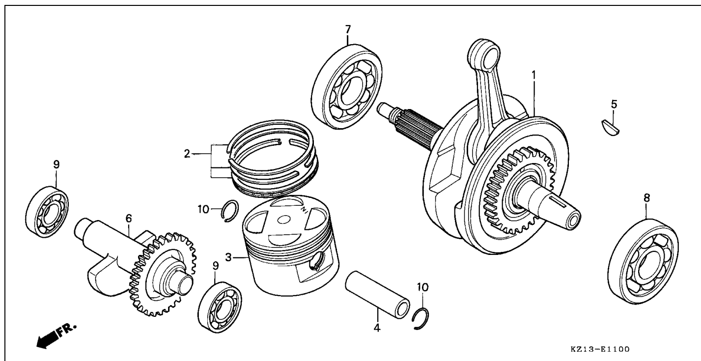
Bloque E-11 CIGUENAL/PISTON
