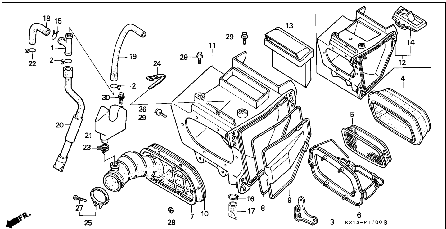
Bloque F-17 LIMPIADOR DE AIRE
