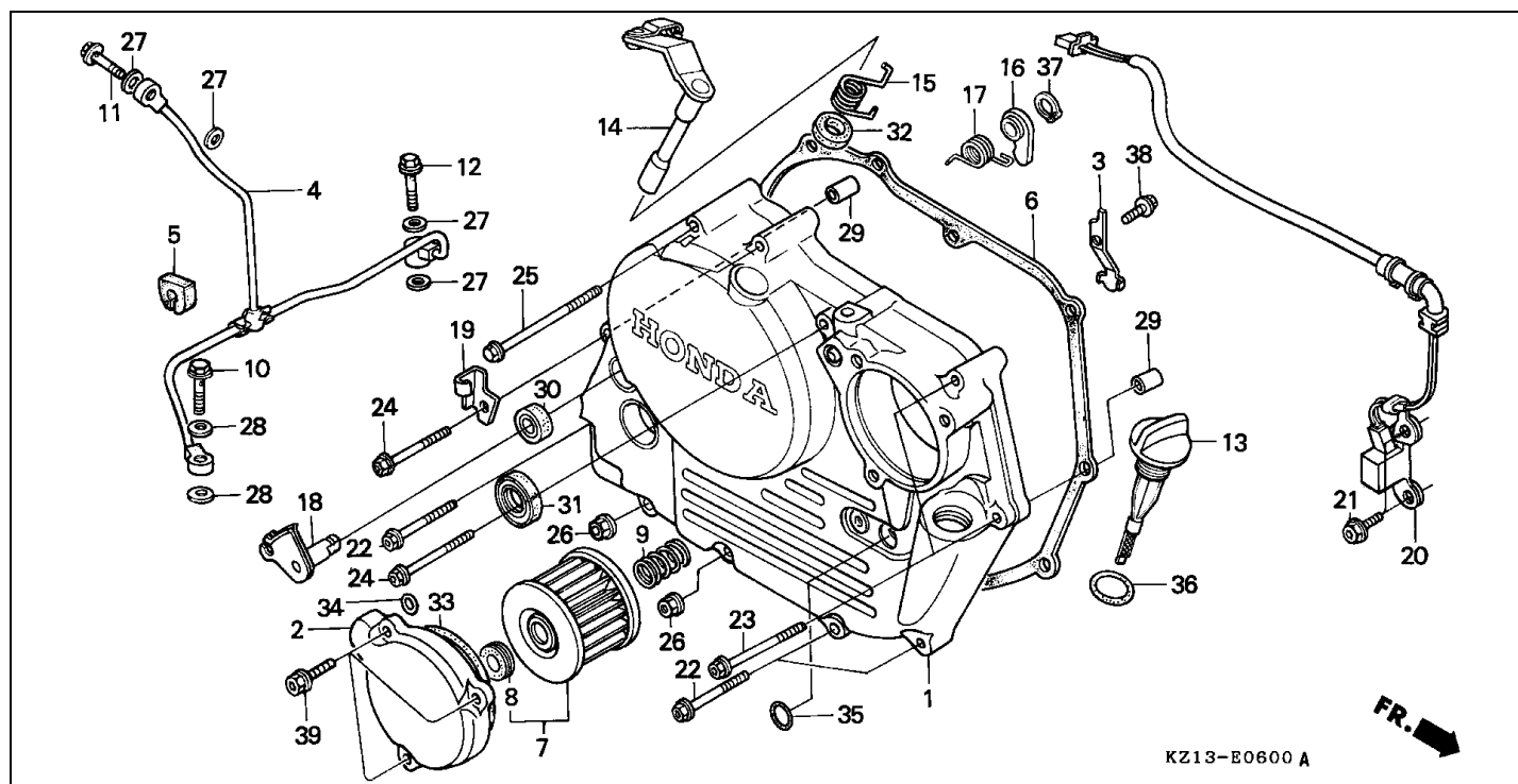
Bloque E-6 CUBIERTA DE CARTER DER.
