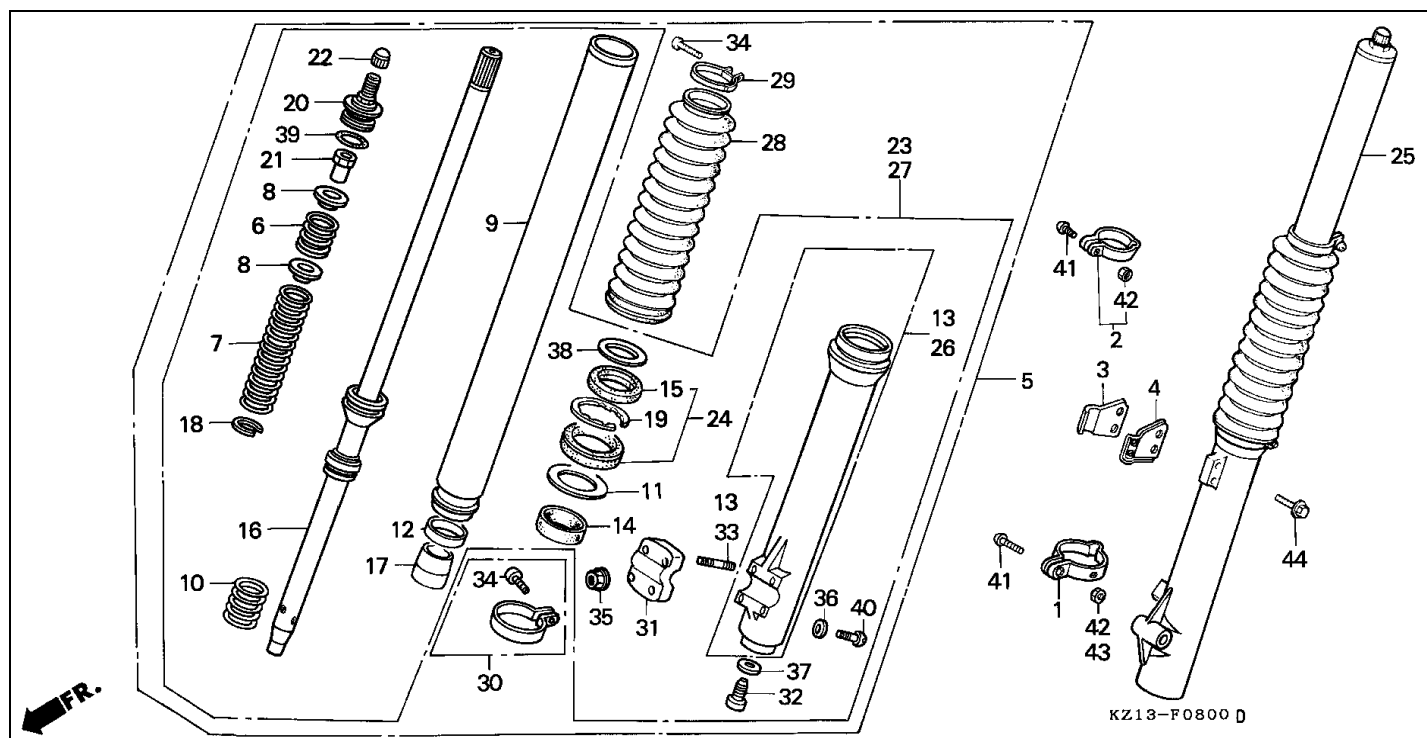
Bloque F-8 HORQUILLA DELANTERA
