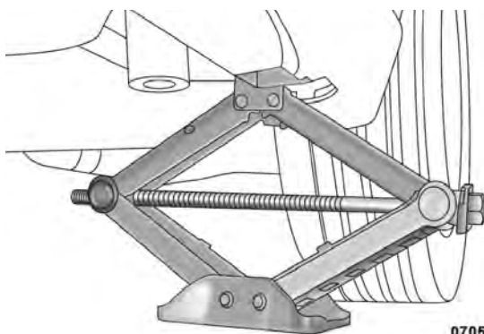
Colocación del gato en la parte trasera
