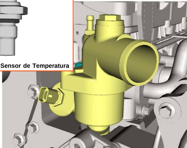
Carcaça termostática
