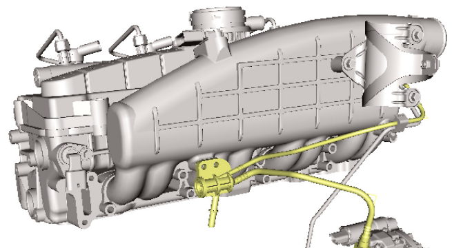
Carcaça do sensor de temperatura de combustível
