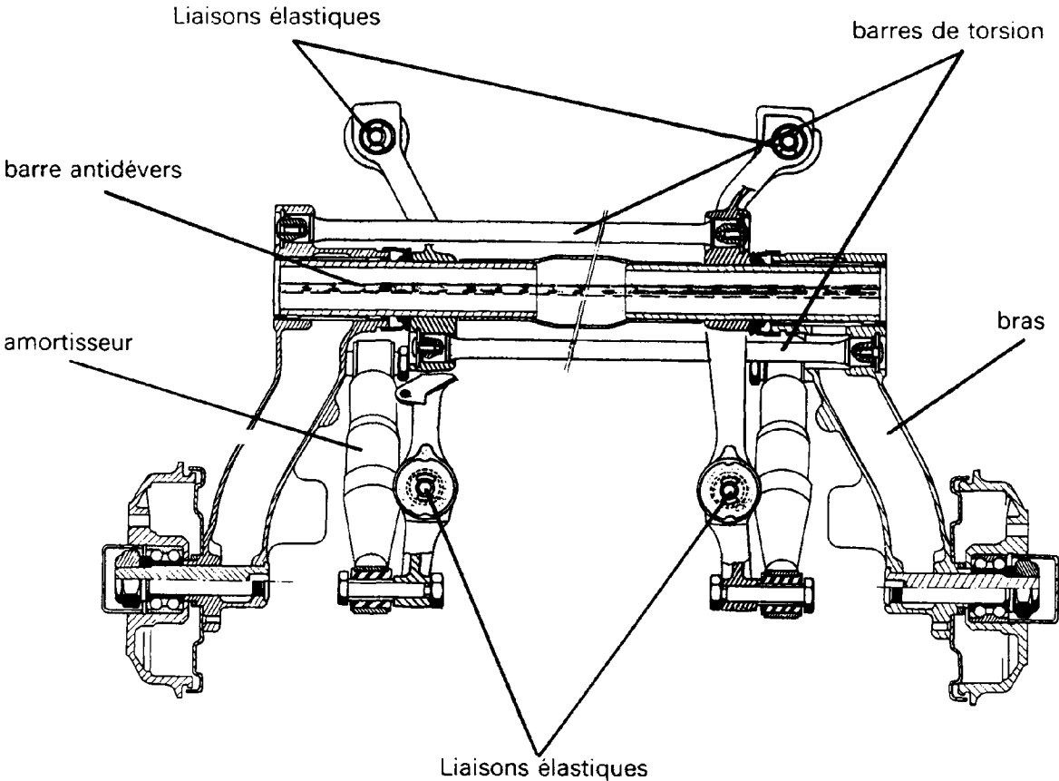
SUSPENSION - TRAIN ARRIÈRE
