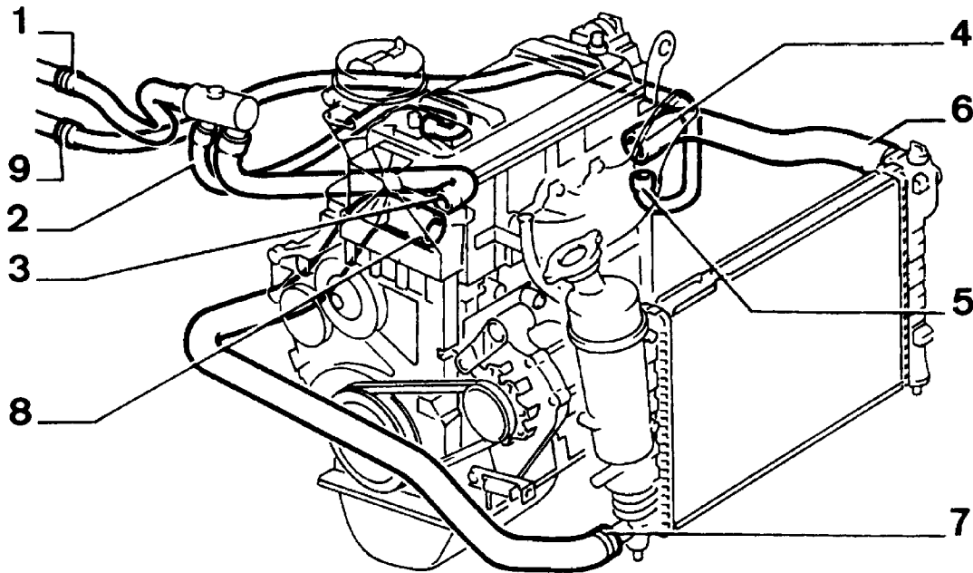
- 1 : Sortie aérotherme - 2 : Retour réchauffage carburateur - 3 : Retour aérotherme sur moteur - 4 : Sortie moteur - 5 : Sortie moteur vers aérotherme - 6 : Entrée radiateur - 7 : Sortie radiateur - 8 : Entrée moteur - 9 : Retour aérotherme.
