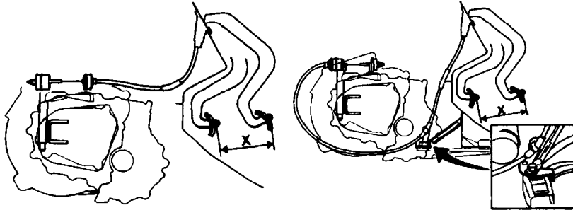
Câble d'embrayage
