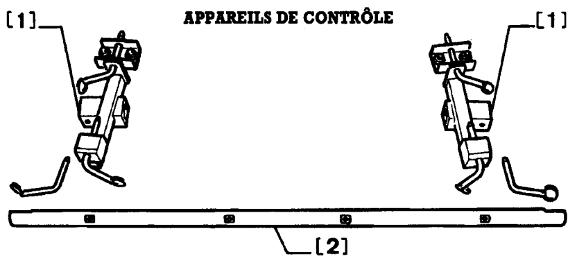
(1) Gabarits de contrôle ancrage bras de suspension AV (-).1108B (2) Tube de contrôle (-).1108C
