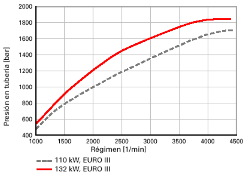
Comparación de la presión de inyección entre 110 kW y 132 kW, EURO III: presión máxima en la tubería ante el inyector
