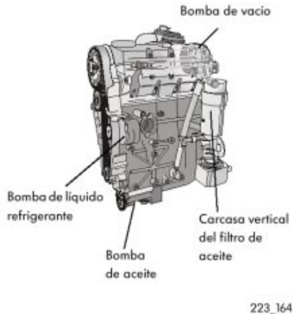
Serie de motores EA 188
