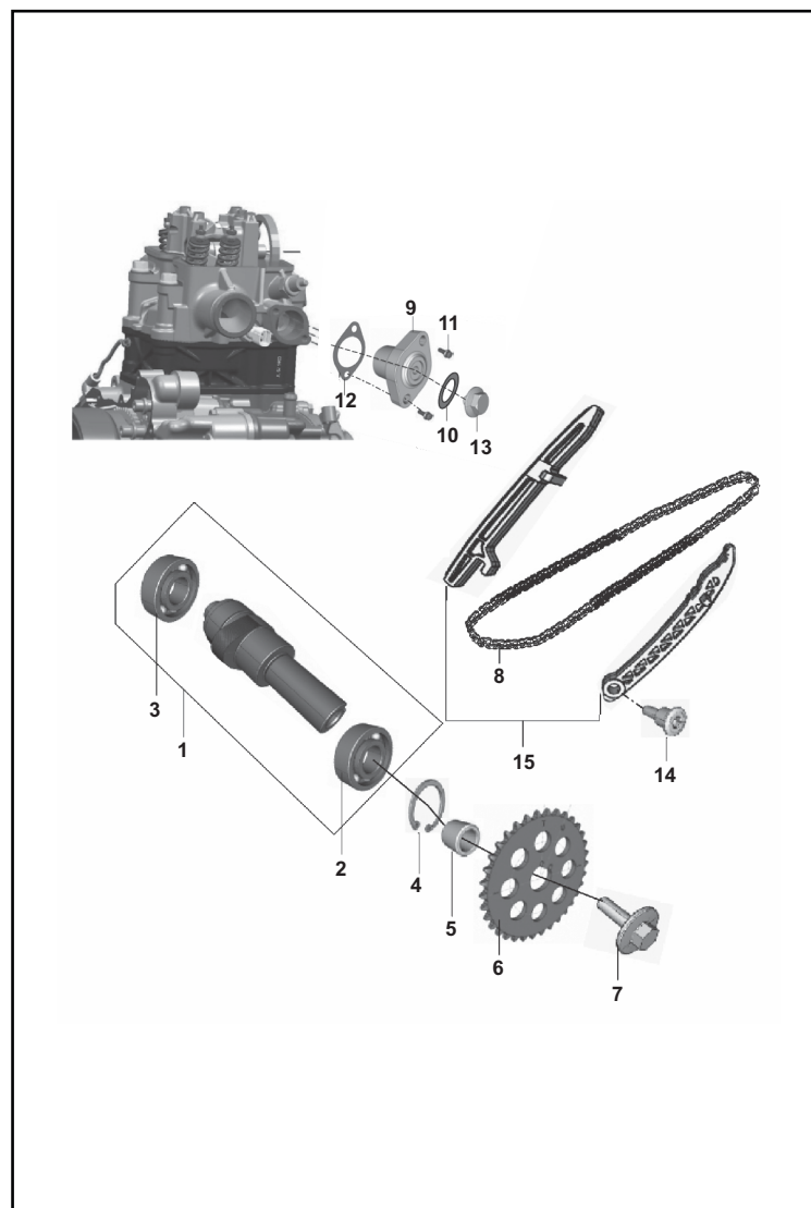
FIGURA N° 5: EJE DE LEVAS / TENSOR CADENILLA
