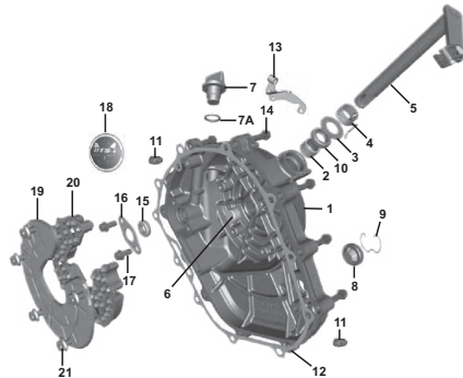
FIGURA N° 16: CUBIERTA CLUTCH
