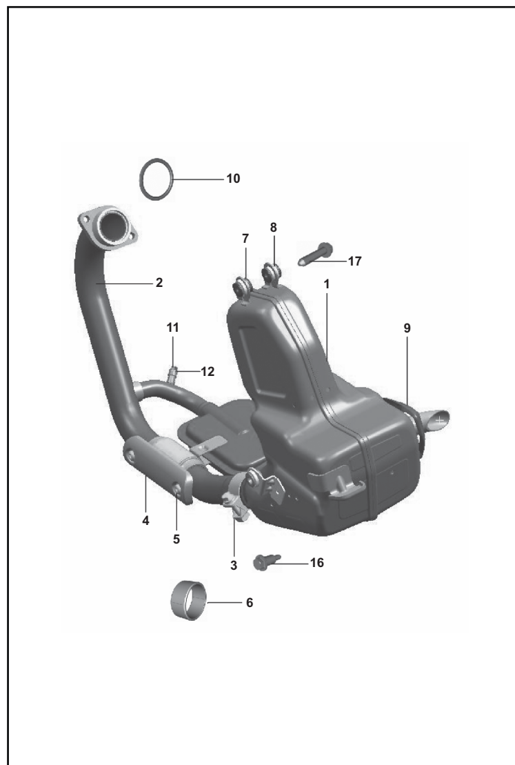
FIGURA N° 21: SILENCIADOR
