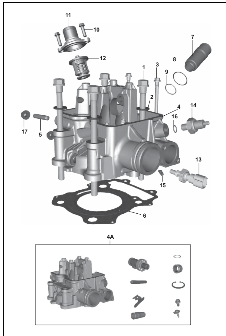
FIGURA N° 3: CULATA
