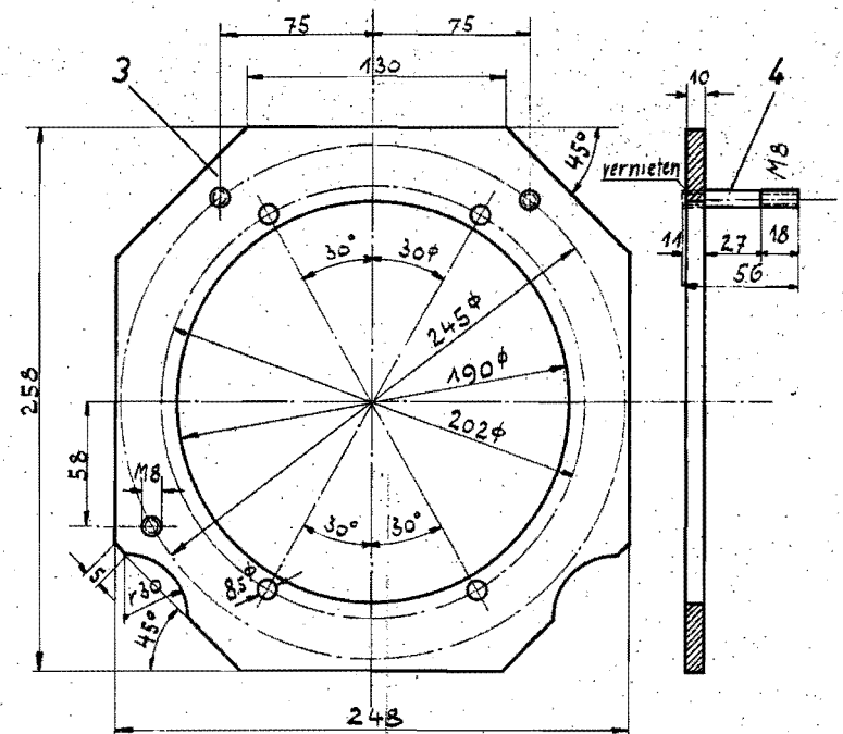
Zwischenplatte zum Aufspannen von Motor und Getriebe R24 R25
