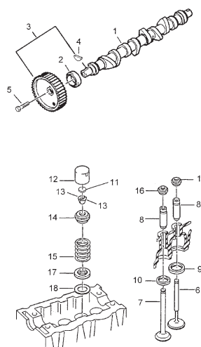
FIG.16 CAM SHAFT (TURBO DIESEL)
