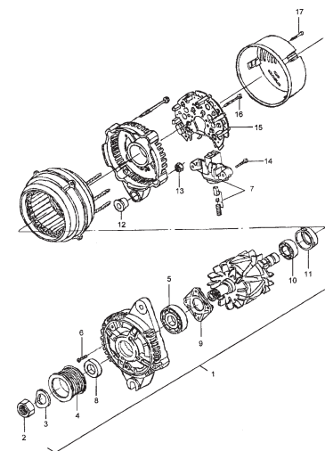
FIG.61 GENERATOR (TURBO DIESEL)
