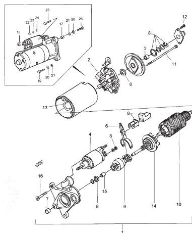
FIG.59 STARTING MOTOR (TURBO DIESEL)
