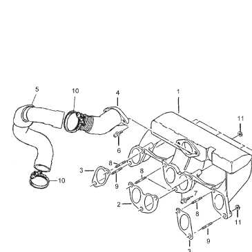
FIG.21 INTAKE MANIFOLD (TURBO DIESEL)
