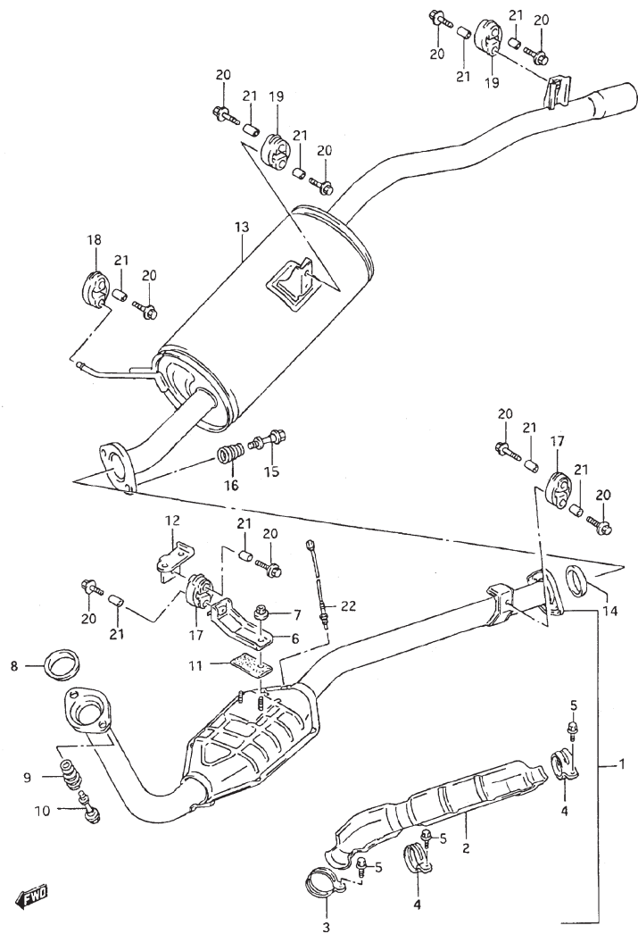
FIG.32
