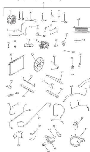
FIG.137 AIR CONDITIONER (TURBO DIESEL)
