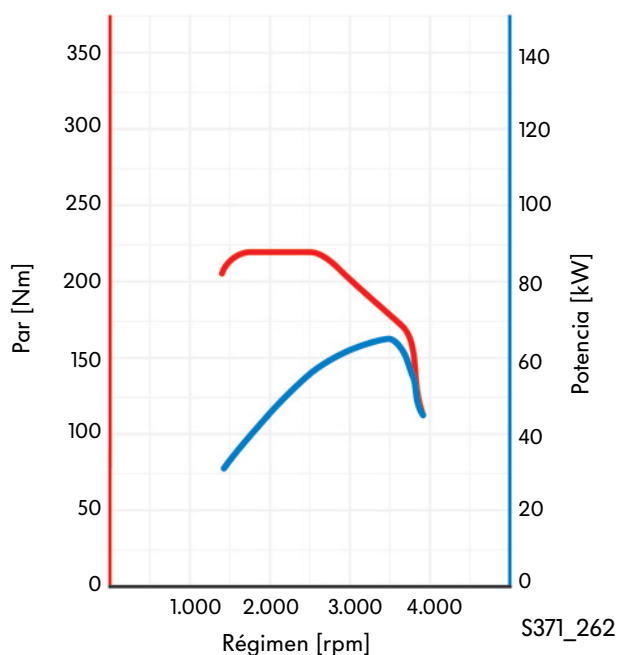
Curva de potencia y par
