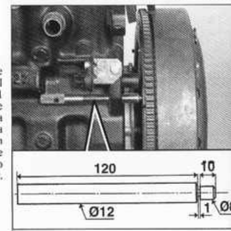
Colocación del pasador de calado del cigüeñal en el volante motor (útil BMW 11 2 300), con cotas de fabricación (en mm). La ranura de 1 mm sirve para la rotura del pasador, en caso de olvidarse de desmontarlo, evitando daños al motor.
