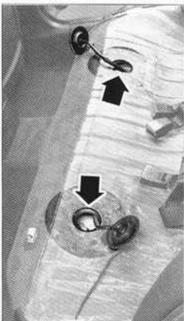
Situación de las trampillas de acceso a los conjuntos aforador / bomba y bomba de alimentación, debajo de la banqueta trasera. Para acceder a las fijaciones de las trampillas, levantar el insonorizante y el revestimiento de suelo.
