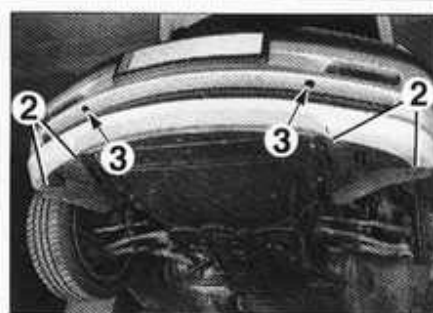
Desmontaje del parachoques delantero.
