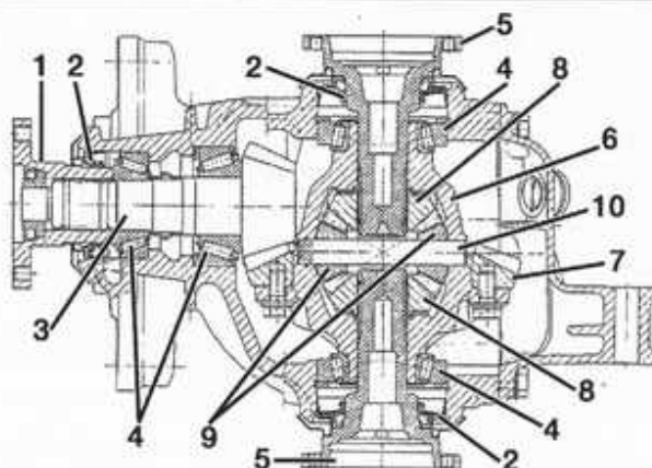
CORTE LONGITUDINAL DEL PUENTE TRASERO.
