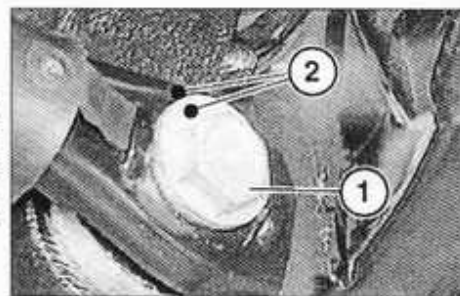
Reglaje de la caída de rueda.
