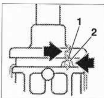
Alineamiento del capuchón (1) con la caja (2). En esta posición, la dirección está en línea recta.
