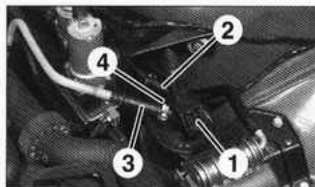
ALIMENTACION DE COMBUSTIBLE. 1. Tornillo de fijación del captador de presión de alimentación - 2. Tubería de alimentación que viene del depósito - 3. Tubería de alimentación hacia la bomba de alta presión - 4. Tornillo de sujeción del filtro.
