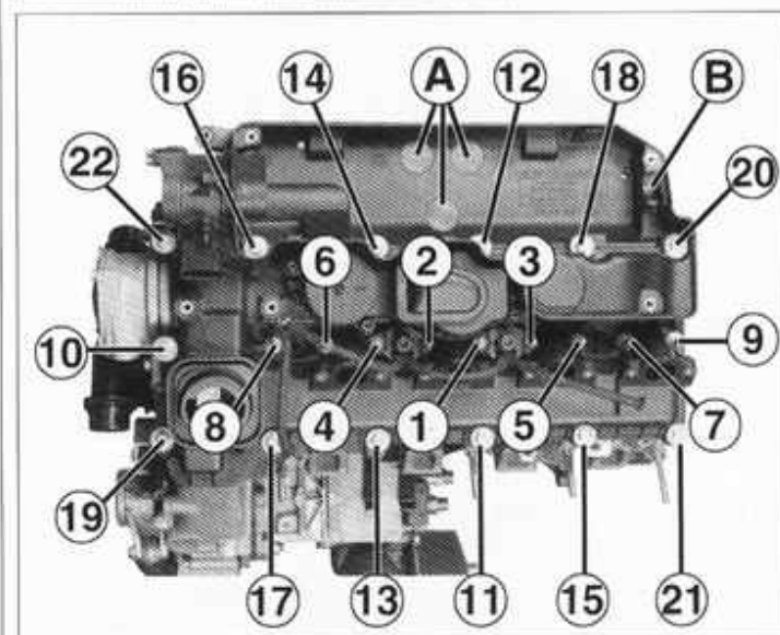
Tapa de culata.
