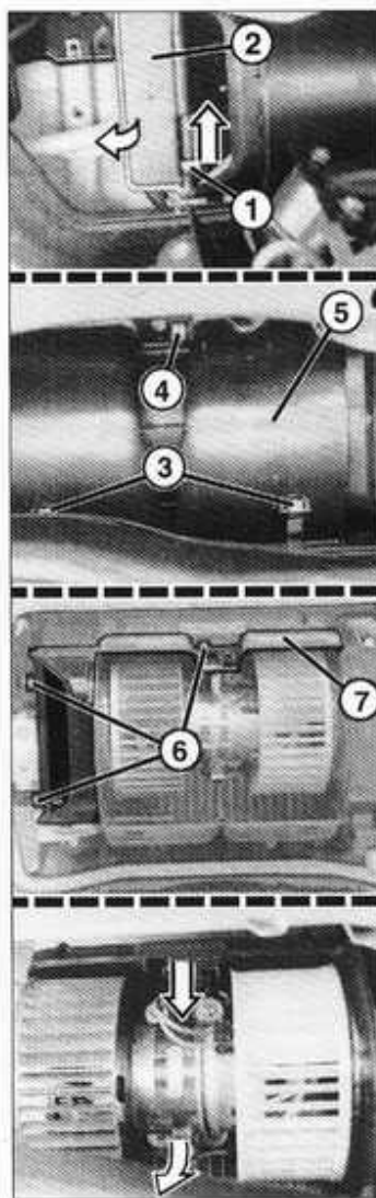
Desmontaje del ventilador de calefacción
