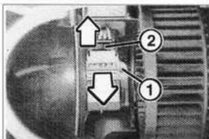
Desmontaje de la resistencia de motoventilador.
