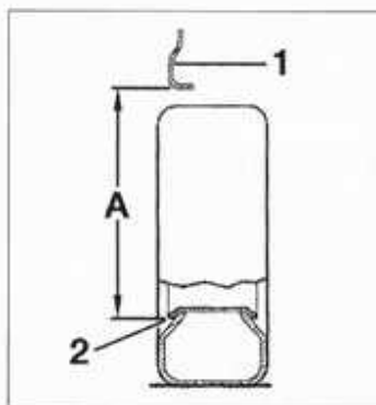
Altura de carrocería "A" - 1. Borde inferior del paso de rueda - 2. Borde de la llanta.
