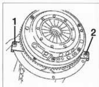
Comprobar el buen posicionado de los casquillos de centrado 1 y 2.
