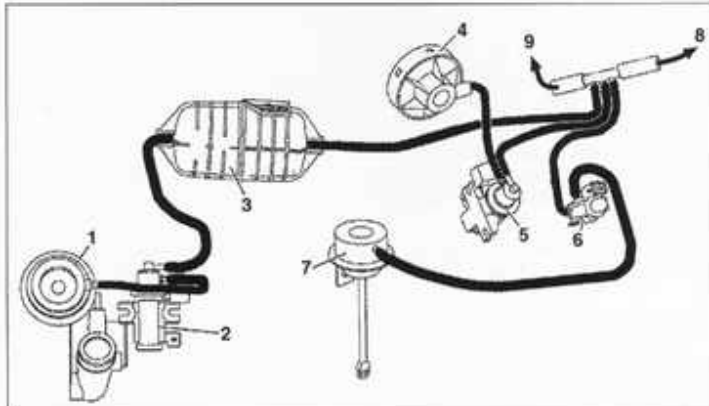
Disposición y conexión de los manguitos de vacío.
