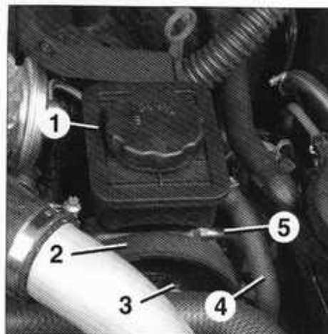
Grupo de la bomba de asistencia de dirección. 1. Depósito de compensación de la bomba - 2. Correa de accesorios - 3. Tornillo de la polea - 4. Conducción de retorno - 5. Conducción de alimentación.
