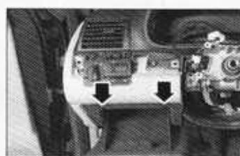
Tornillo de fijación de la guantera izquierda.
