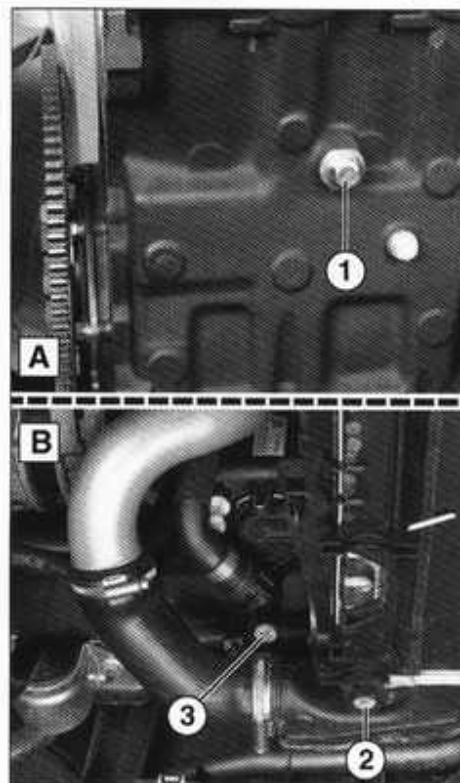
Vaciado del circuito de refrigeración.
