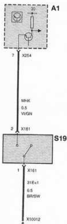
CONTACTO DE COMPARTIMENTO MOTOR
