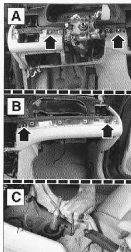
Situación de las tuercas de salpicadero.
