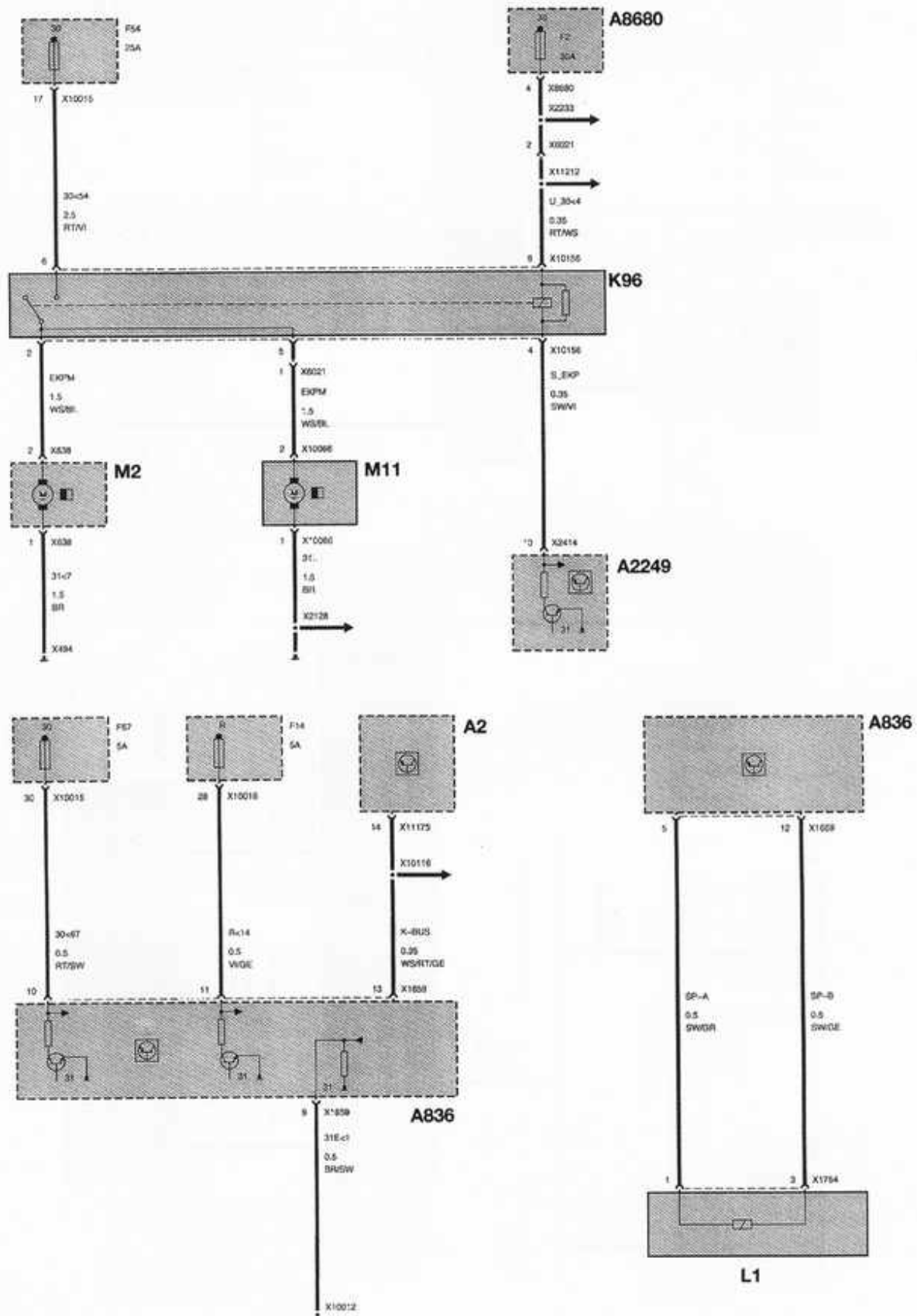
BOMBAS DE ALIMENTACION DE COMBUSTIBLE - SISTEMA ANTIARRANQUE
