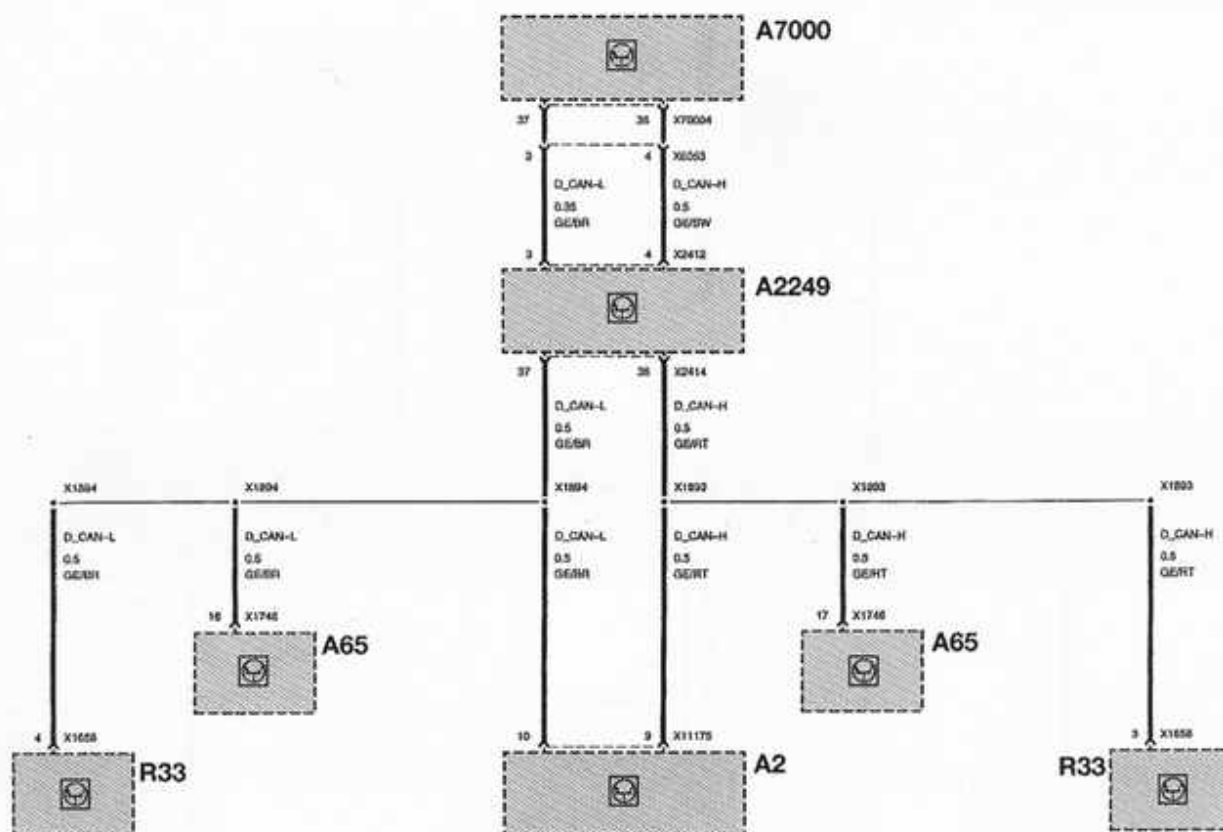
CUADRO DE INSTRUMENTOS. CONECTOR BUS CAN.
