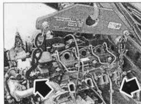
Colocación de los ganchos de izado del motor.
