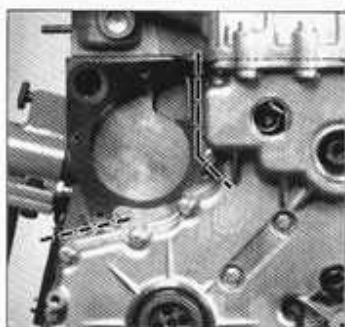
Puntos de corte de la junta de la bomba de agua.
