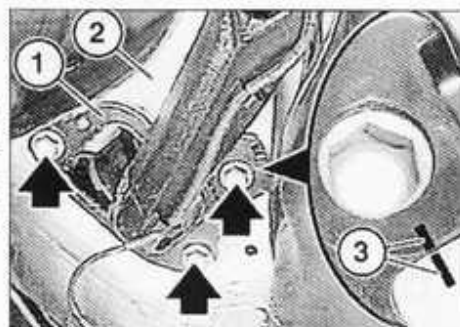
Reglaje del paralelismo.
