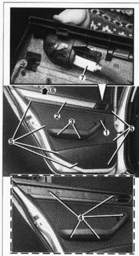
Desmontaje de la guarnición de puerta trasera.
