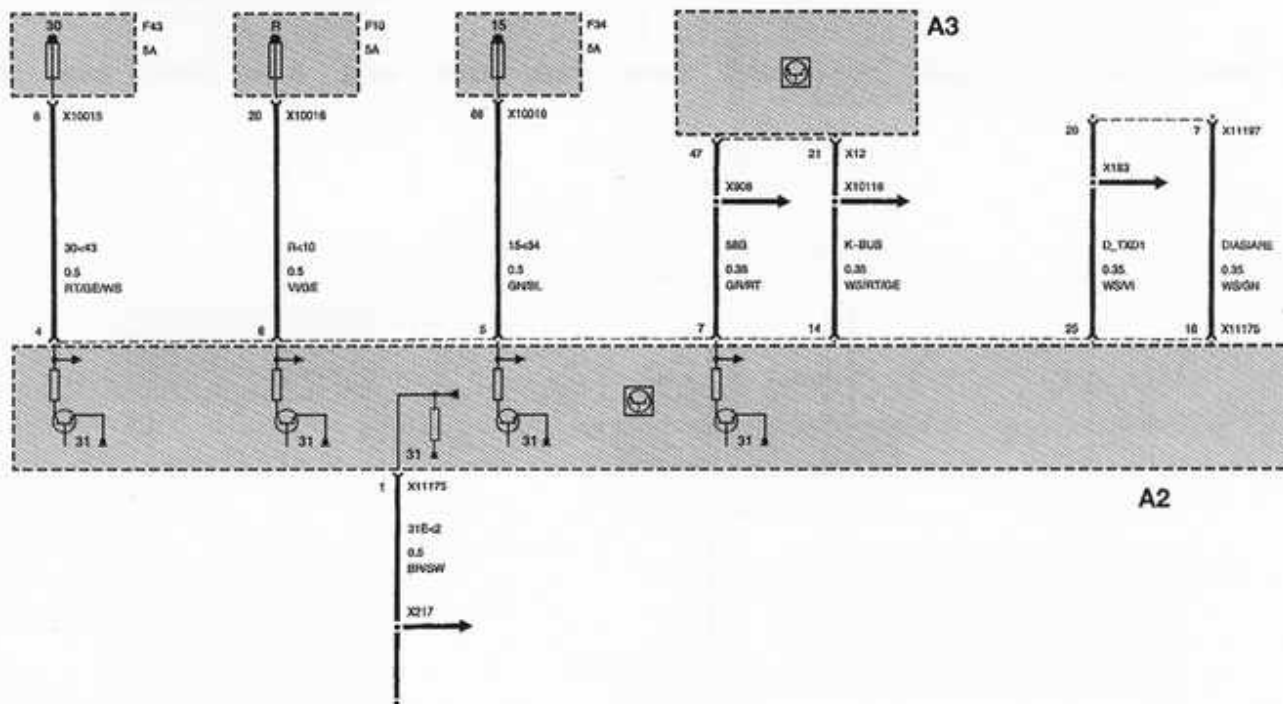
CUADRO DE INSTRUMENTOS. ALIMENTACION.
