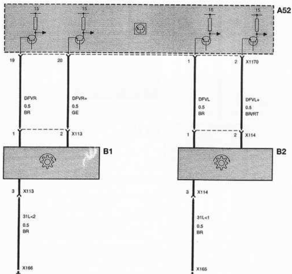
CAPTADORES DE VELOCIDAD DE RUEDAS
