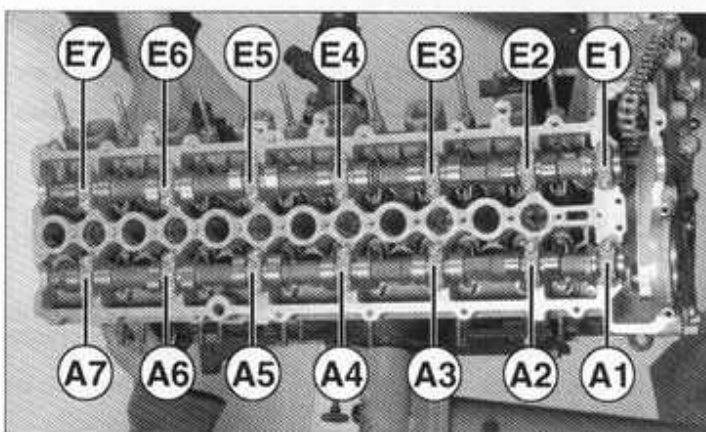
Identificación y sentido de montaje de las tapas de ejes de levas. A1 a A7. Eje de levas de escape. E1 a E7. Eje de levas de admisión.
