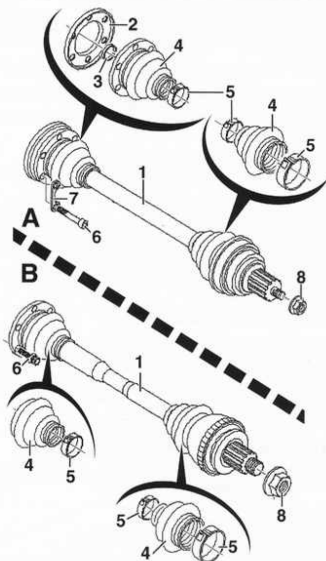
SEMIEJES DE RUEDA.
