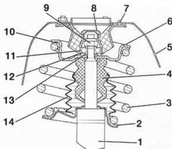
PIEZAS DE UN ELEMENTO DE SUSPENSIÓN
