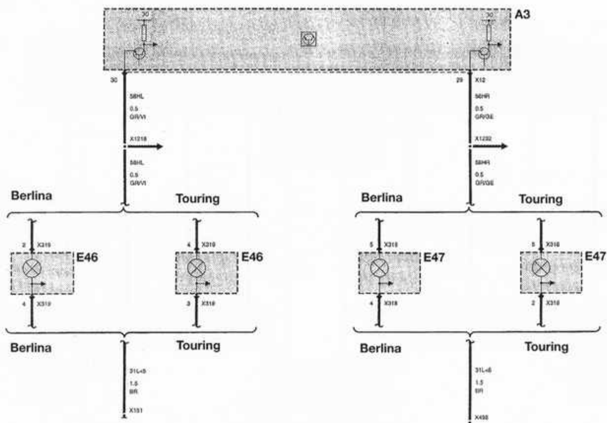
LUZ POSICION TRASERA
