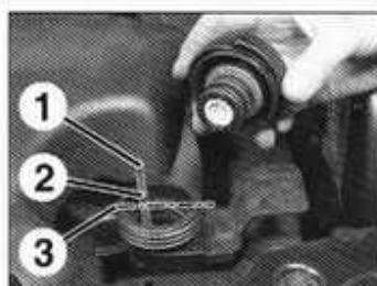
Control del nivel del circuito de refrigeración. El nivel es correcto cuando las marcas (1) en frío ("KALT") ó (2) en caliente ("WARM") del flotador se sitúan a la altura del borde superior del vaso de expansión.
