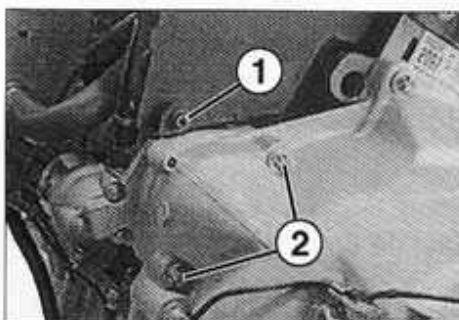
Desmontaje del motor de arranque. 1. Tornillo del aislamiento fónico - 2. Tornillo de fijación.
