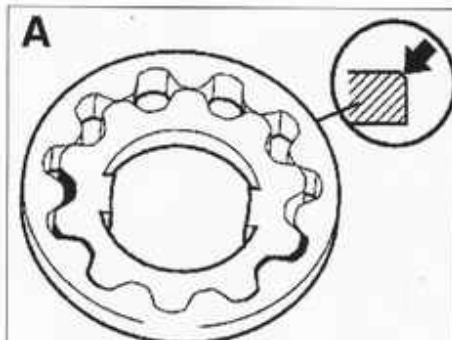
Ensamblado de la bomba de aceite. A. Orientar el chafán del rotor exterior hacia el cuerpo de la bomba -
