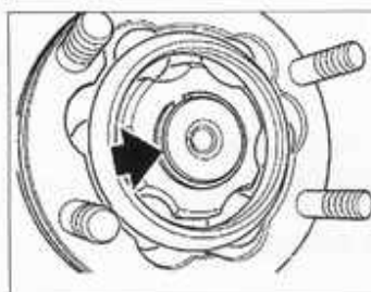
Anillo de freno del acoplamiento trasero sobre el eje transmisión.
