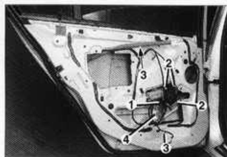
Desmontaje del mecanismo elevavinas trasero.
