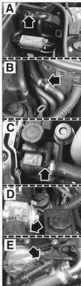
Situación de los tornillos de purga del circuito de refrigeración.
