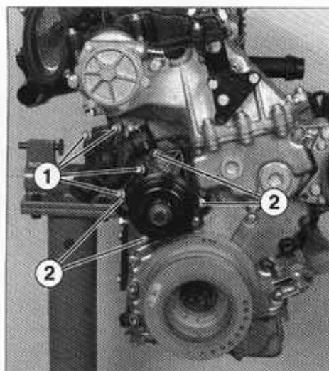
1. Tornillo de fijación del termostato - 2. Tornillo de fijación de la bomba de agua.
