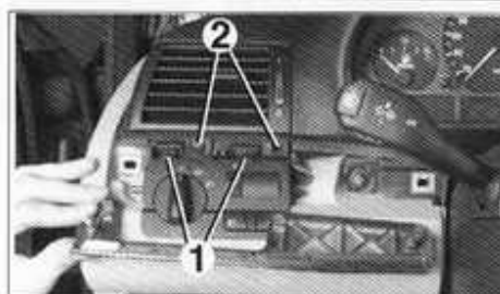
1. Tornillo de fijación de mando de iluminación - 2. Tornillo de fijación de la salida de ventilación izquierda.
