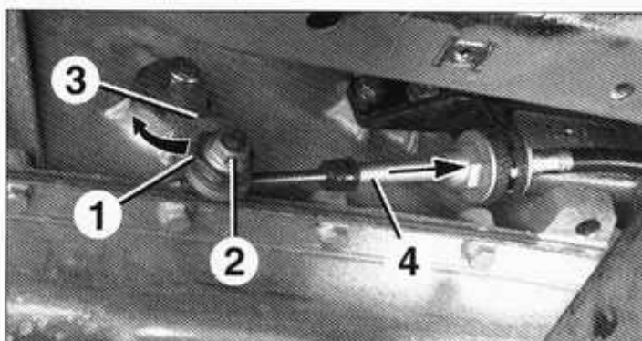
Método de reglaje del cable de selección.
