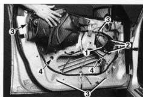
Desmontaje del mecanismo elevavinas delantero.
