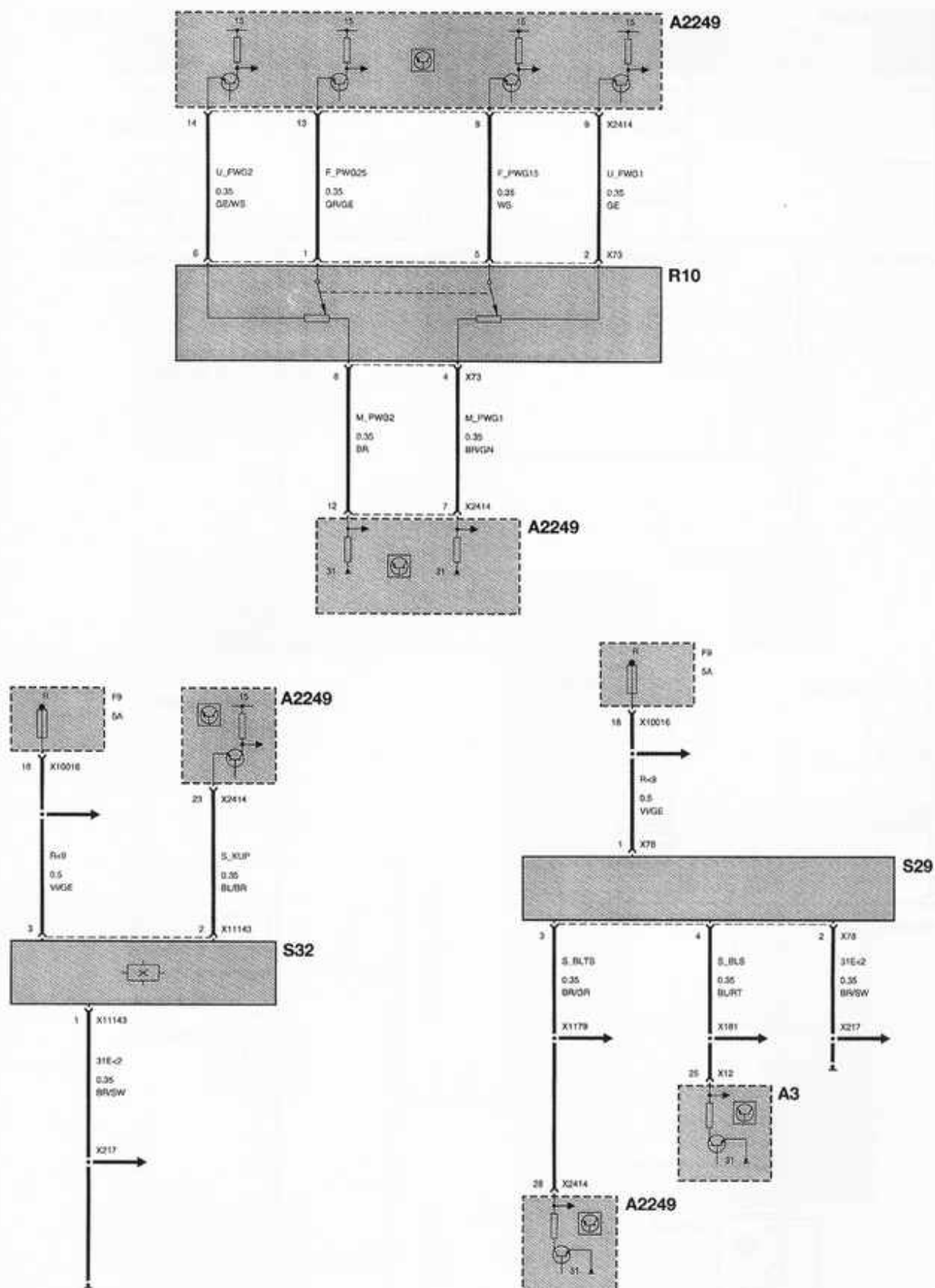
CAPTADOR DE POSICION DE ACELERADOR - CONTACTOR DE EMBRAGUE - CONTACTOR DE LUCES DE STOP
