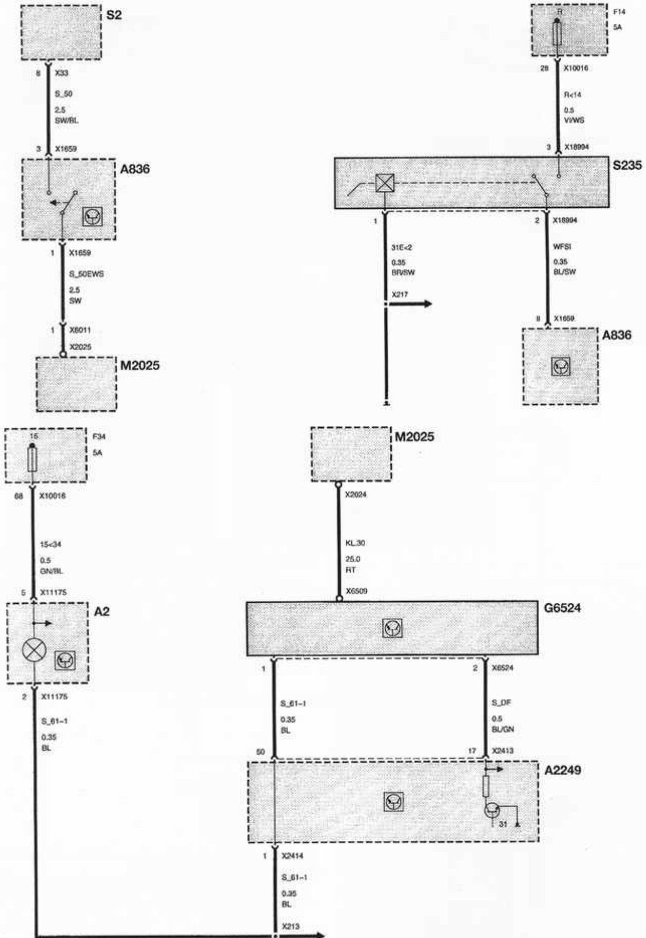
SISTEMA ANTIARRANQUE - CIRCUITO DE CARGA
