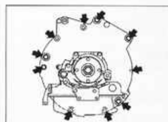
Situación de los tornillos de fijación de la transmisión automática sobre el bloque motor.
