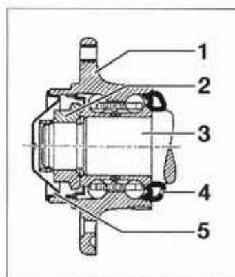
Corte de un cubo delantero. 1. Cubo de rueda - 2. Tuerca con collarín - 3. Mangueta - 4. Chapa guardapolvo - 5. Capuchón.
