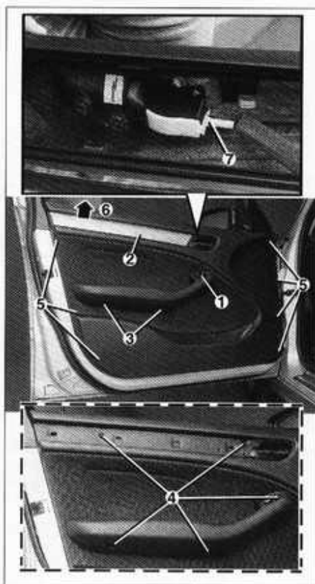
Desmontaje de la guarnición de puerta delantera.
