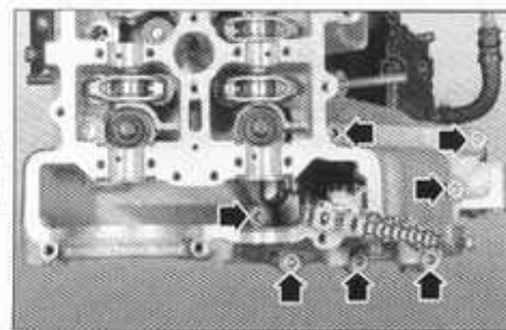
Situación de los tornillos de fijación de la culata sobre el cárter de distribución.
