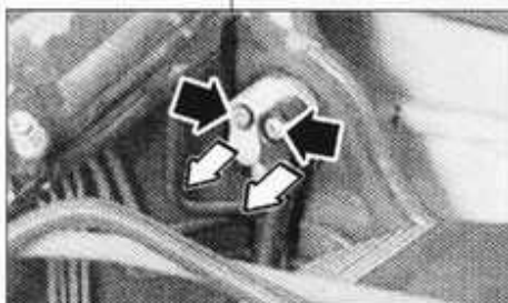
Desmontaje del tubo de aspiración de climatización.
