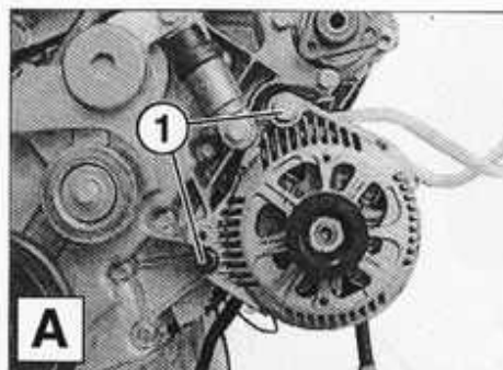
Desmontaje del alternador. A. 320d - B. 330d -
