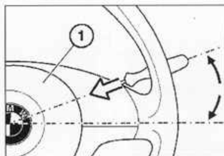
Desmontaje del airbag conductor (1).
