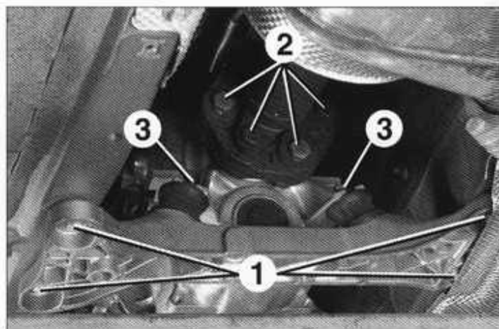
Desmontaje de la caja de velocidades.
