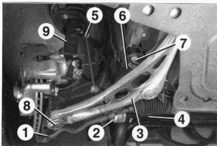
SITUACIÓN DE LAS DIFERENTES PIEZAS DE UN SEMITREN DELANTERO
