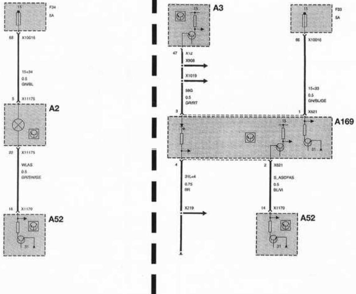
ALIMENTACION ABS, TESTIGO ABS EN CUADRO INSTRUMENTOS, TECLA ASC.
