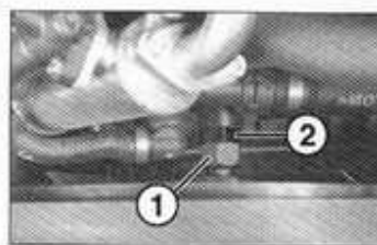
Desmontaje del viscoacoplador del ventilador de refrigeración (con transmisión automática).
