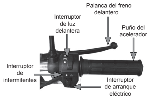
Imagen 6. Mando derecho
