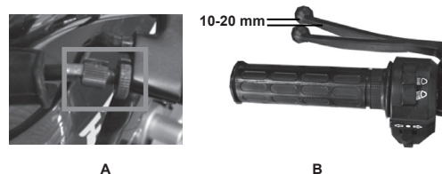
Imagen 30. Ajuste de la palanca del embrague
