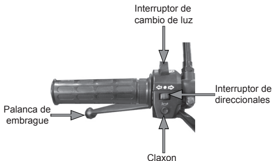
Imagen 9. Mando izquierdo
