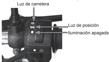
Imagen 7. Interruptor de luz delantera
