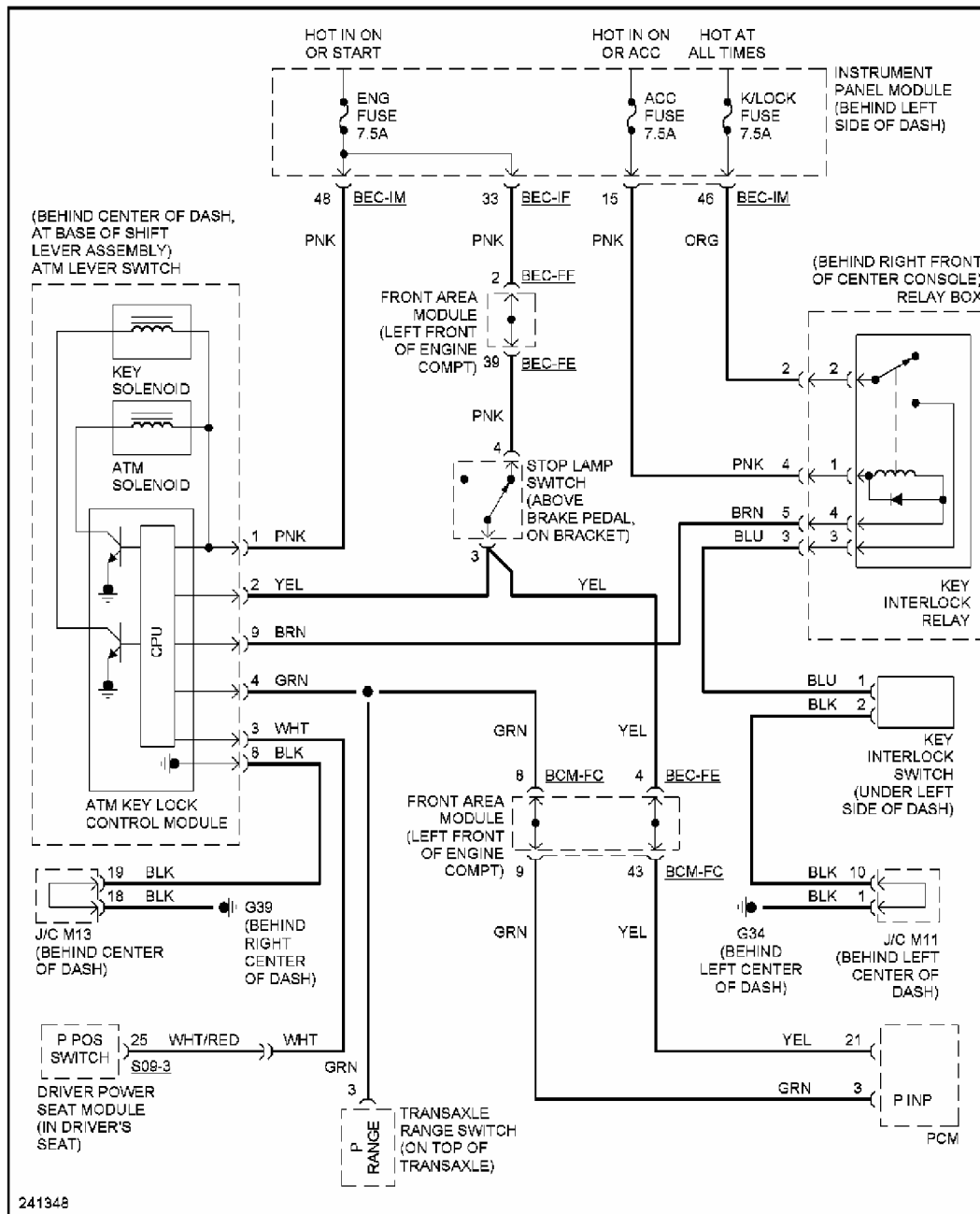
Fig. 68: Shift Interlock Circuit
