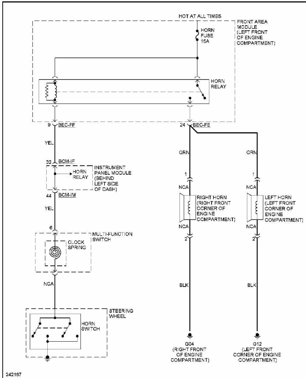
Fig. 37: Horn Circuit
