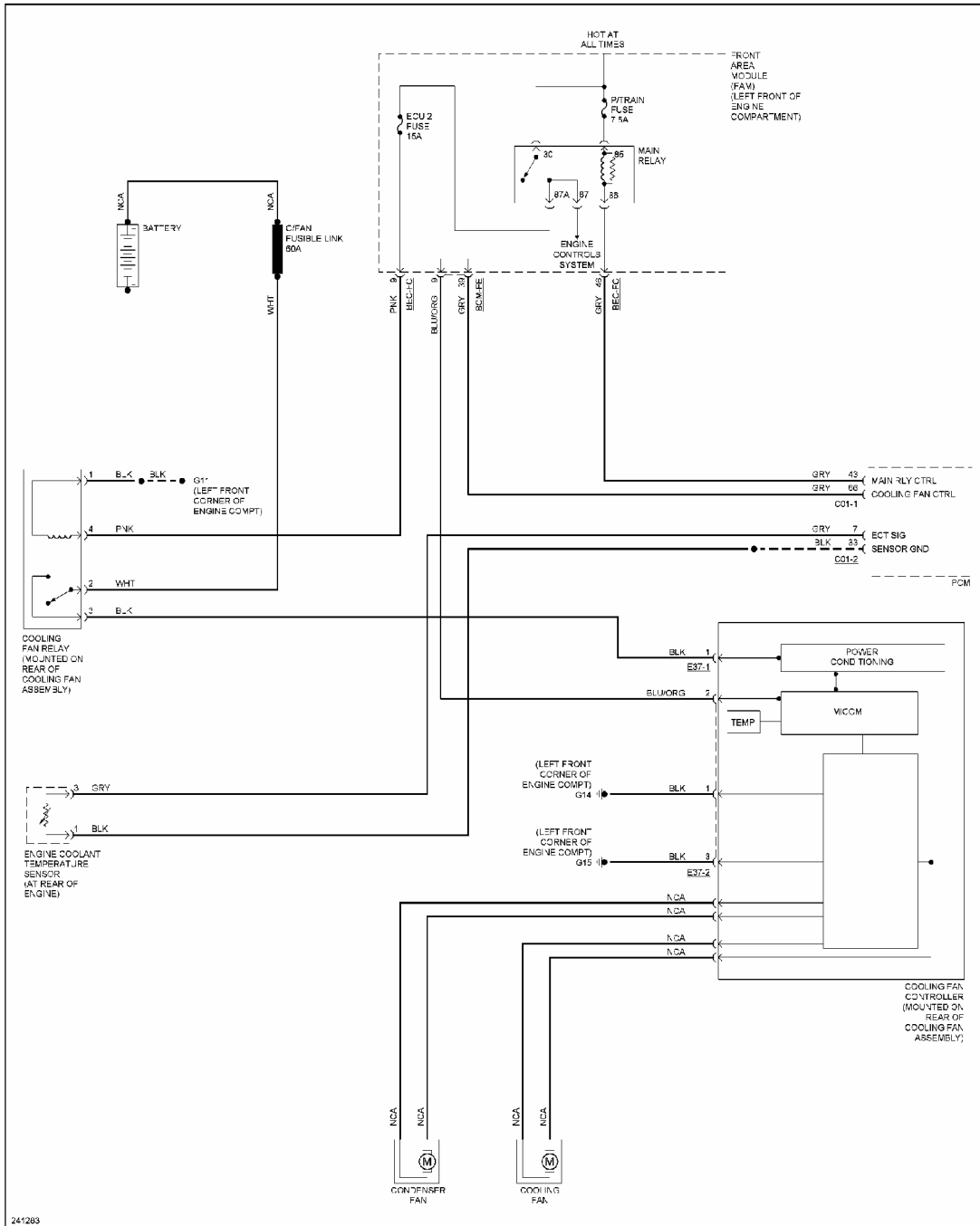
Fig. 19: Cooling Fan Circuit
