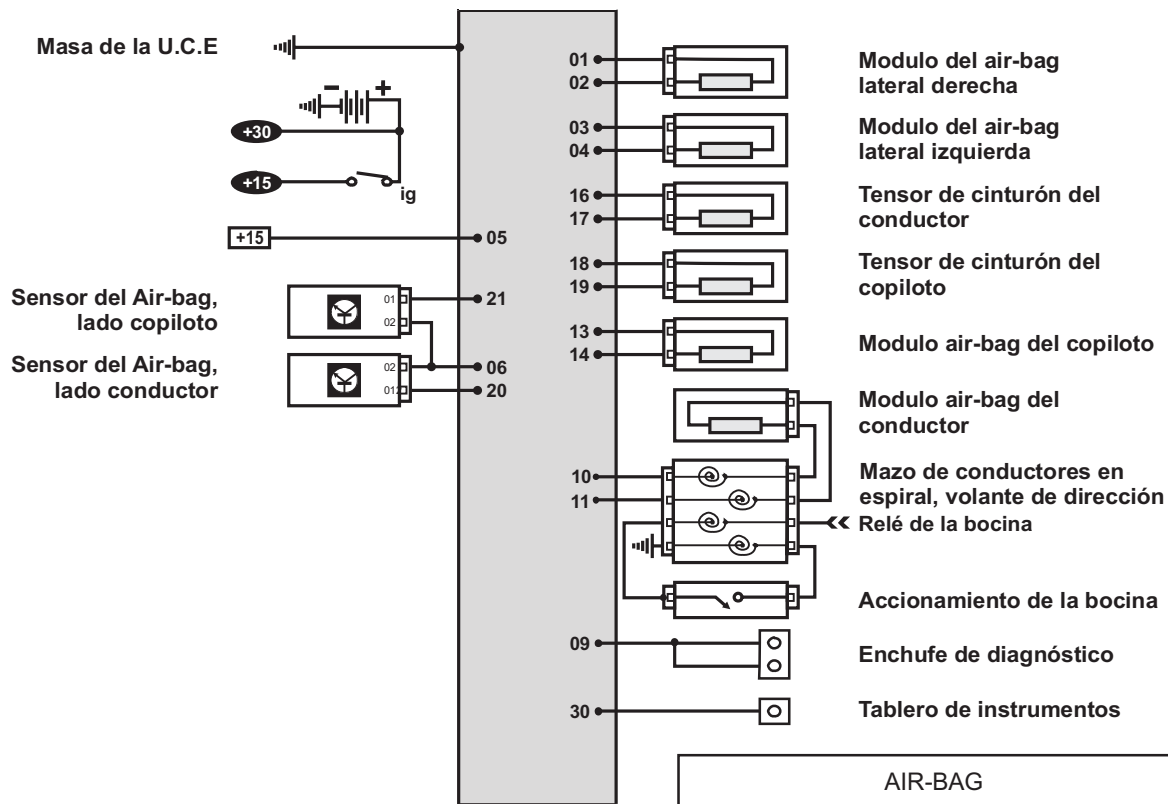
Fig. VW Airbag 03
