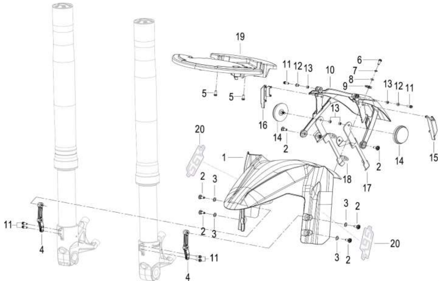
FIG 13 LODERA DELANTERA
