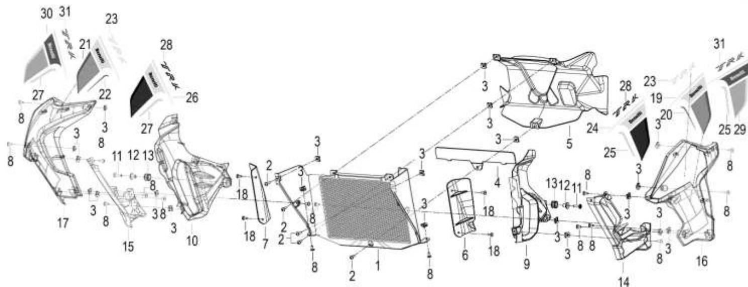
FIG 17 COBERTORES
