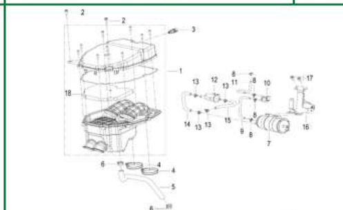
FIGURA N°6: FILTRO DE AIRE
