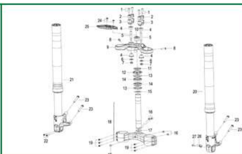
FIGURA N°2: T DE BARRAS
