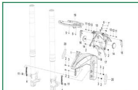
FIGURA N°13: LODERA DELANTERA
