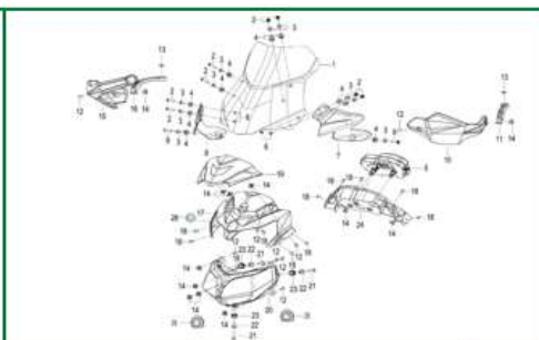
FIGURA N°14: SILVIN, ASPIROMETRO Y COBERTORES
