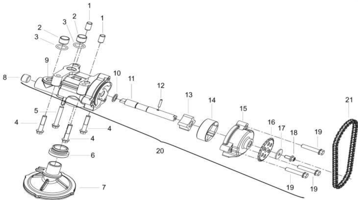
FIG 35 BOMBA DE ACEITE
