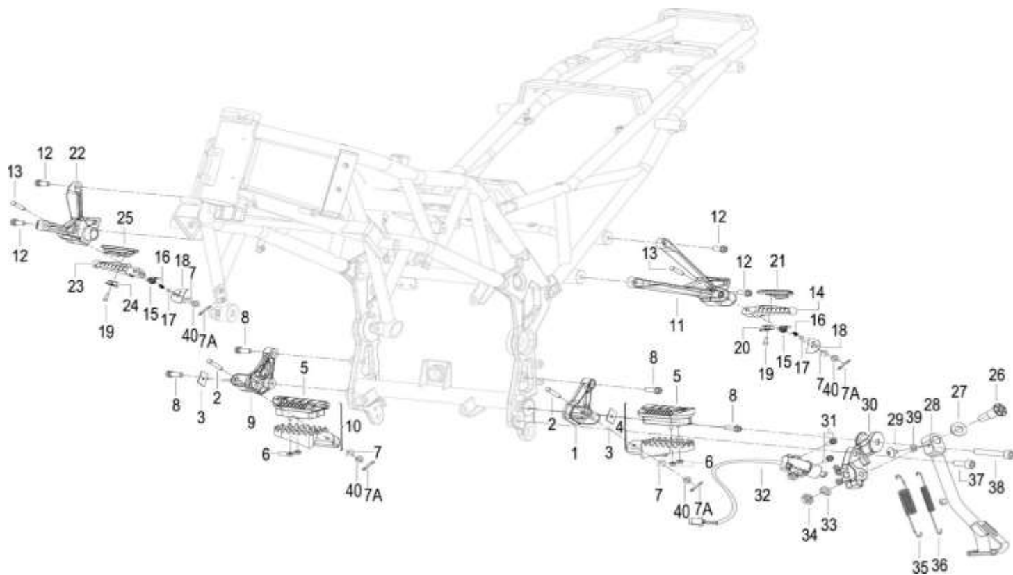
FIG 12 REPOSAPIES
