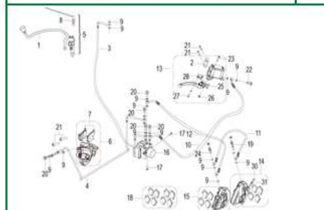
FIGURA N°4: SISTEMA DE FRENO DELANTERO Y TRASE
