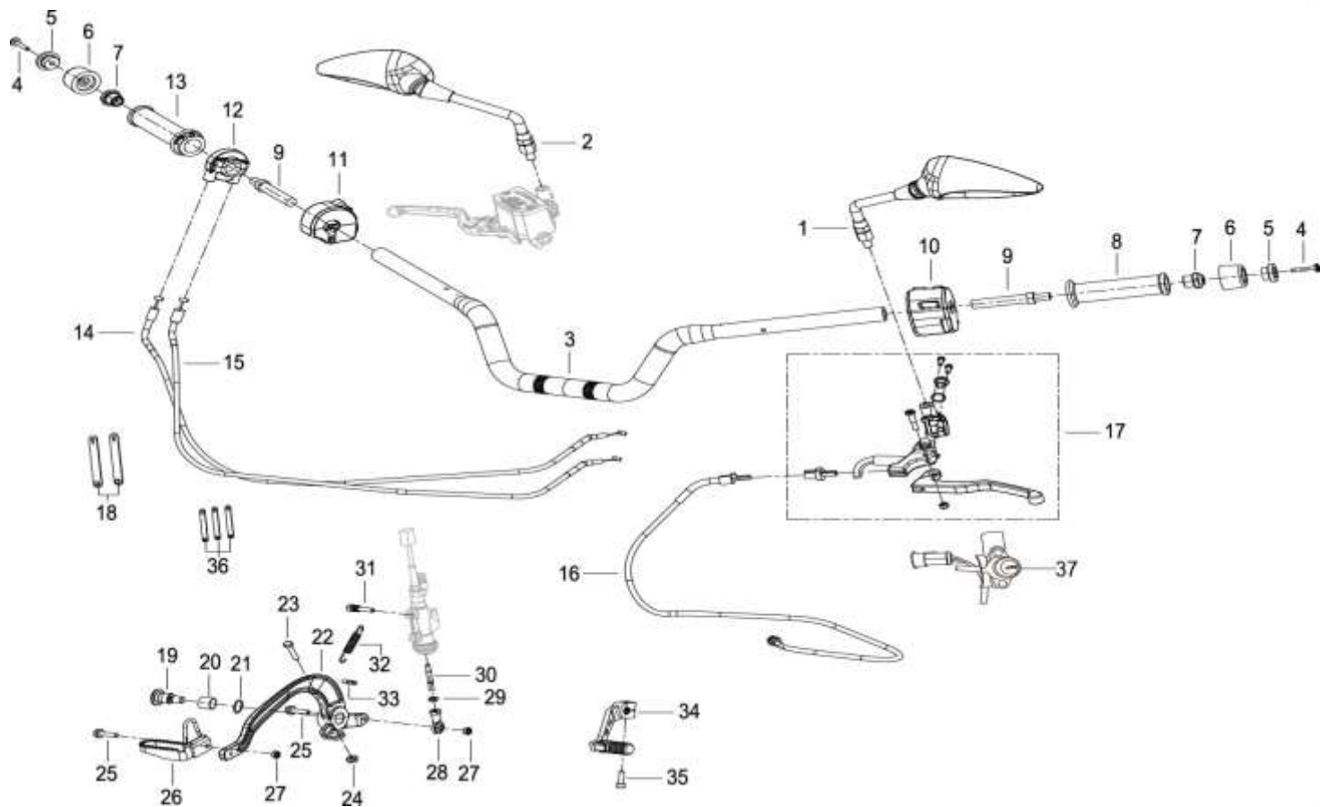
FIG 1 TIMÓN Y CABLES
