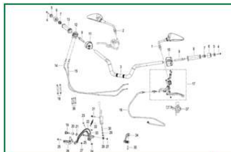
FIGURA N°1: TIMÓN Y CABLES
