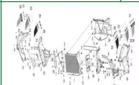
FIGURA N°17: COBERTORES
