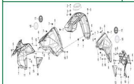
FIGURA N°16: COBERTORES DE TANQUE
