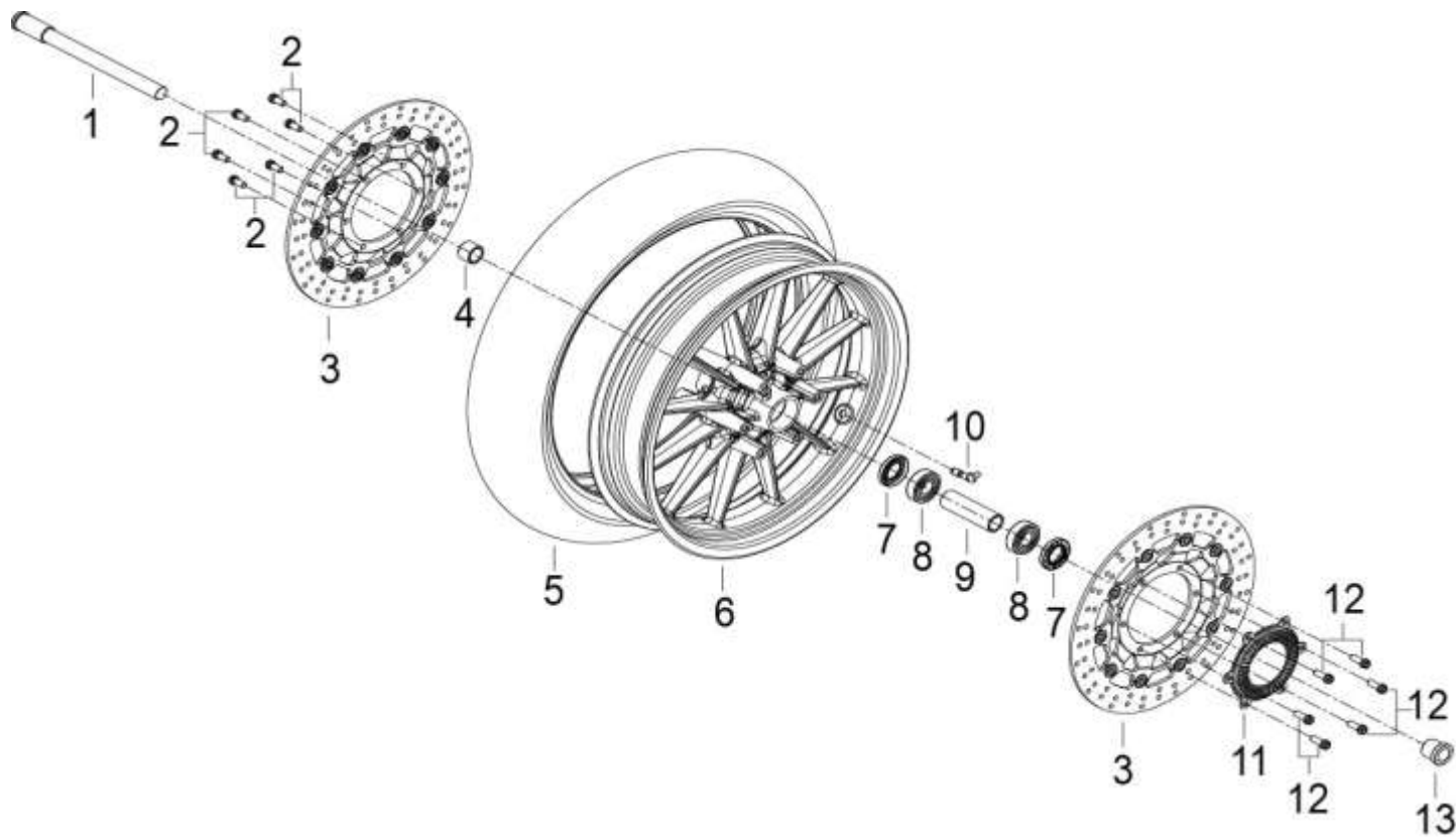
FIG 3 RUEDA DELANTERA
