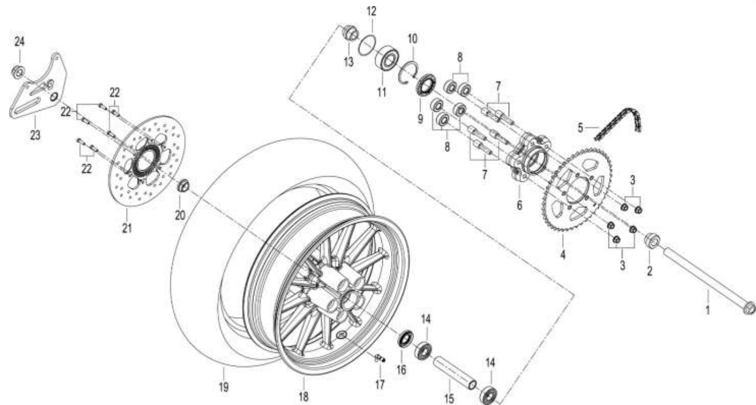
FIG 9 LLANTA TRASERA
