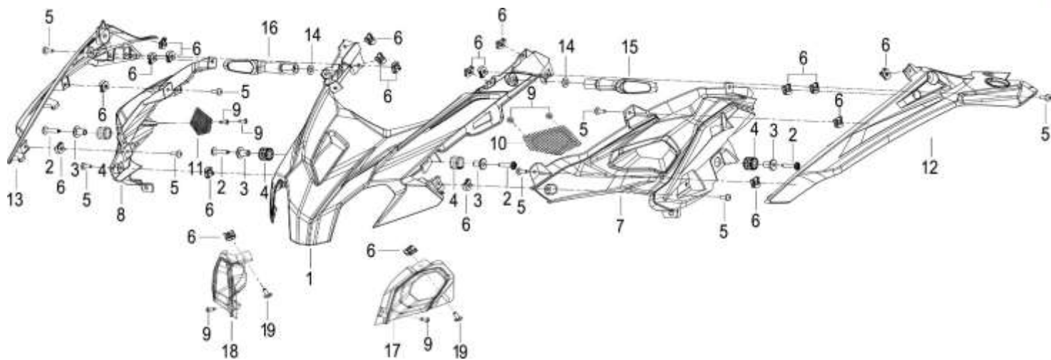
FIG 15 COBERTORES Y PIDEVIAS
