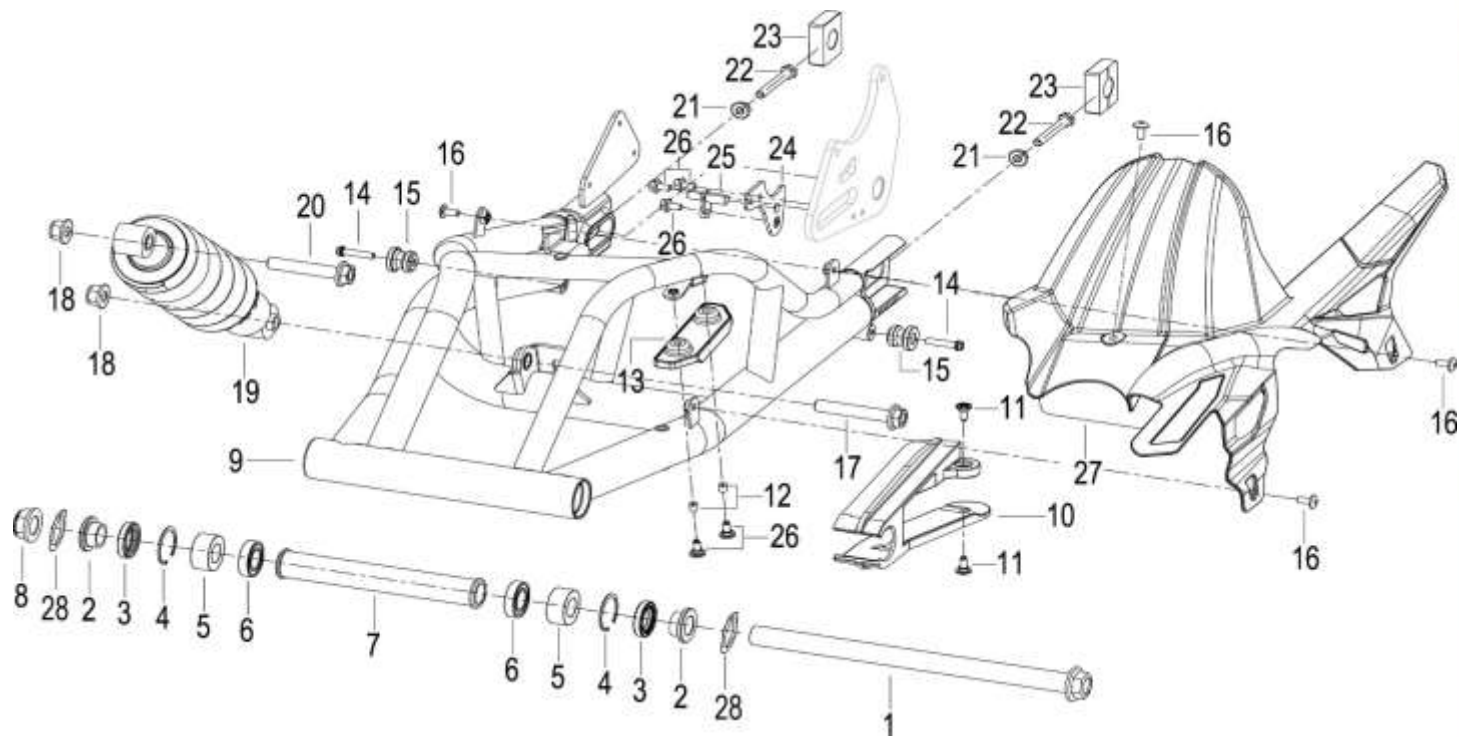
FIG 8 MULETA, LODERA TRASERA Y MONOSHOCK
