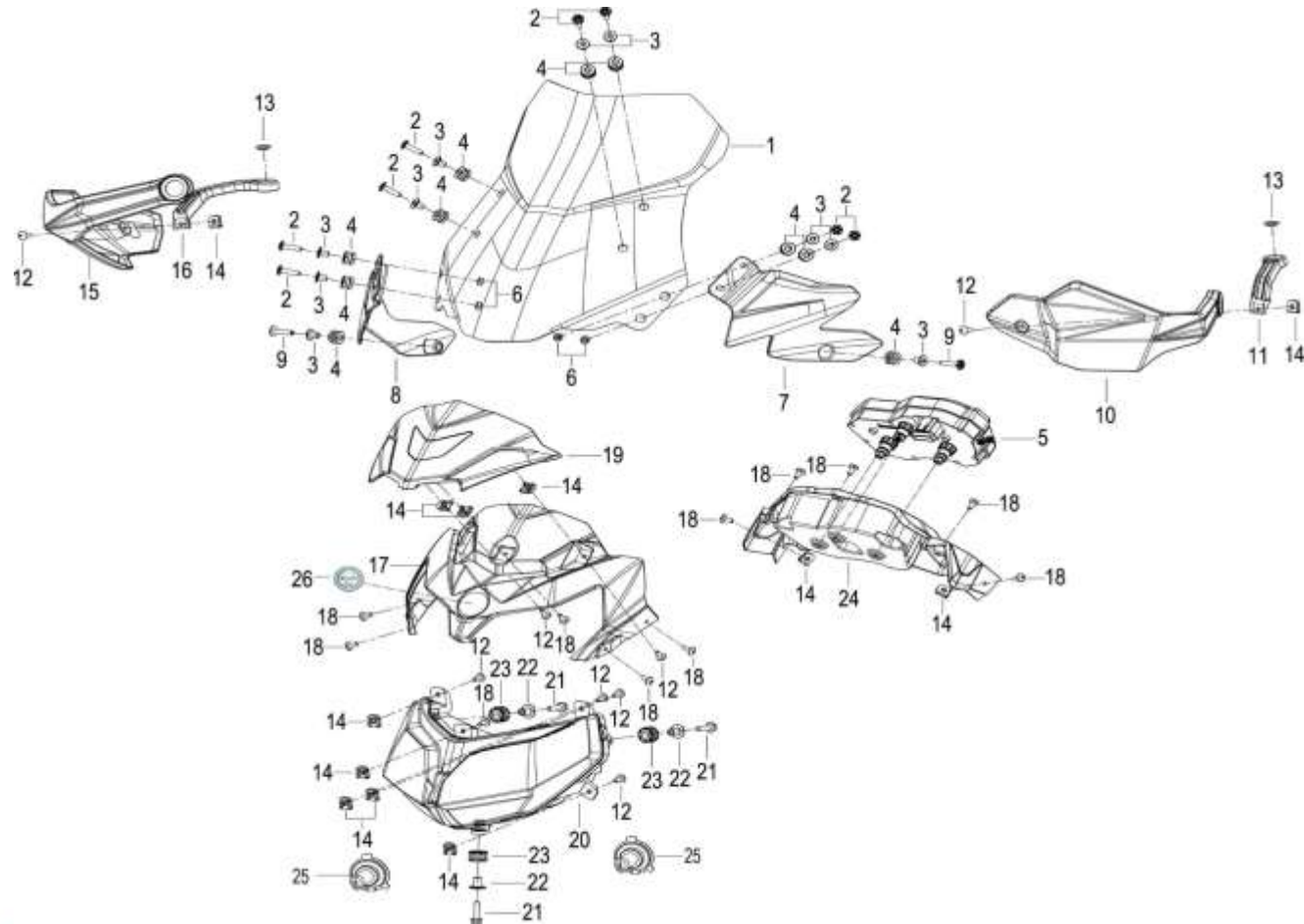
FIG 14 SILVIN, ASPIROMETRO Y COBERTORES
