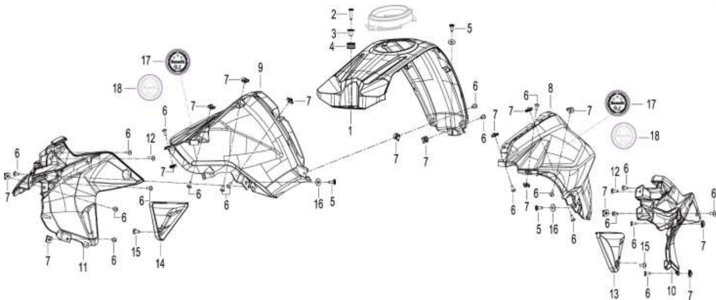
FIG 16 COBERTORES DE TANQUE
