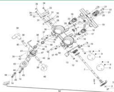
FIGURA Nº37: CUERPO DE ACCELERACIÓN
