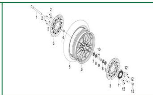
FIGURA N°3: RUEDA DELANTERA
