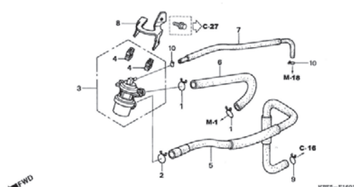
C-17 Inyección de Aire • Válvula Controladora
