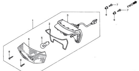
F-26 Taillight
