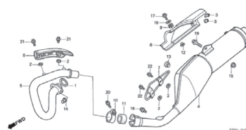
C-18 Silenciador
