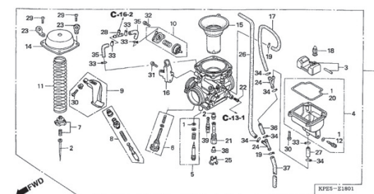
M-18 Carburador
