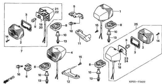
F-25 Winker
