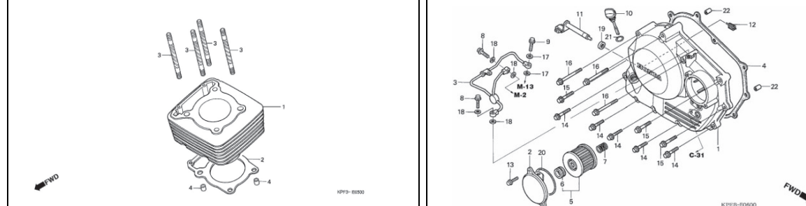
M-9 Cubierta de la Carcasa Izquierda del Motor
