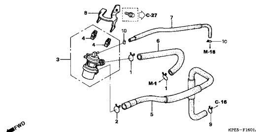
C-17 Válvula Controle / Air Injection Cont. Valve / Valvula Controladora • Inyeccion Aire
