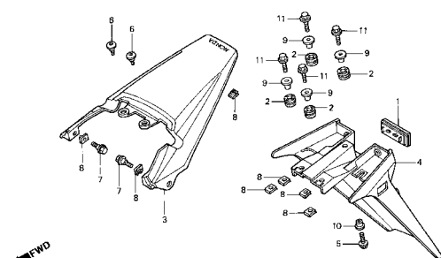
C-24 Para-Lama Traseiro / Rear Fender / Parafango Trasero
