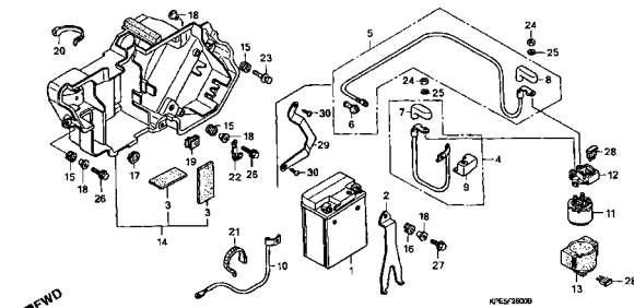
C-27 Bateria / Battery / Batería
