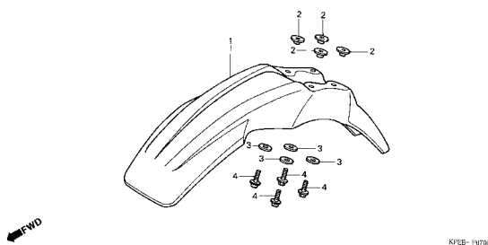
C-7 Para-Lama Dianteiro / Front Fender / Parafango Delantero
