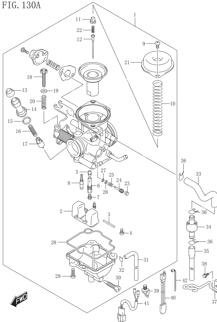
FIG.130A (1-B-10) CARBURETOR
