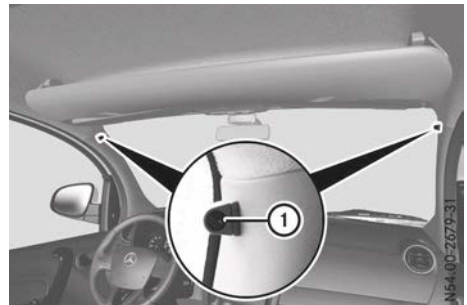
① Sensores situados en el montante A
