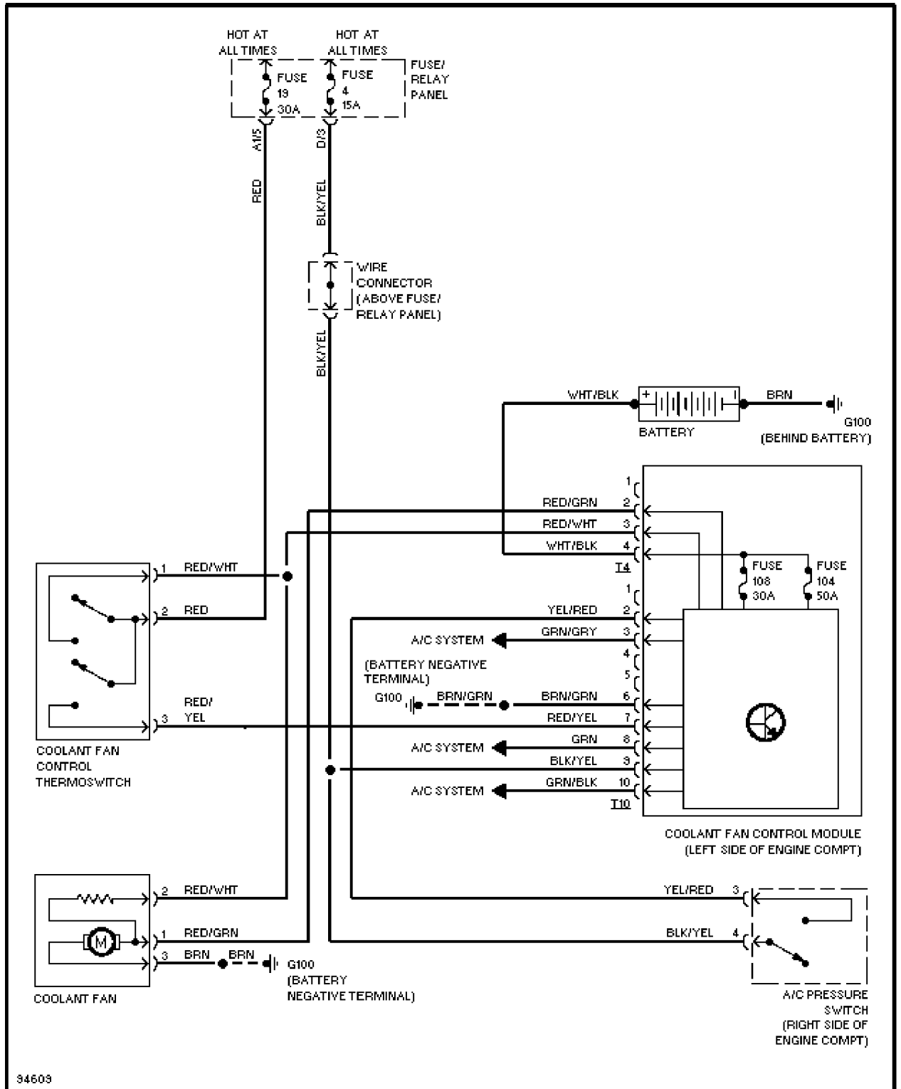
2.0L, Cooling Fan Circuit
