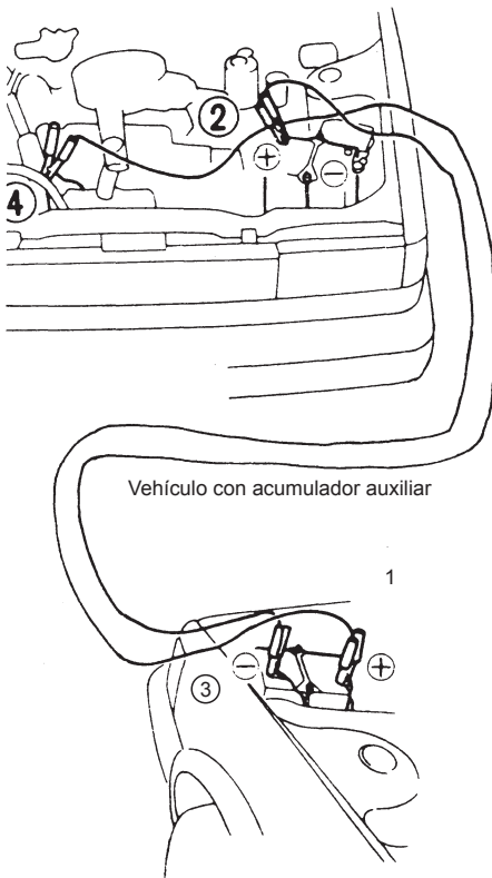
Vehículo arrancado con acumulador auxiliar
