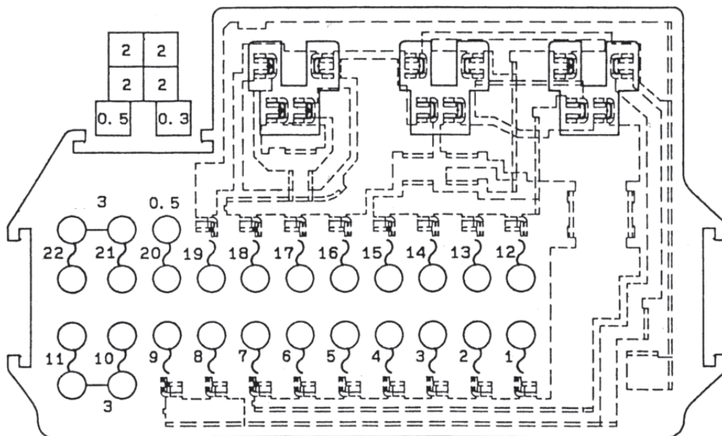
Esquema de conexiones (Continuación)
