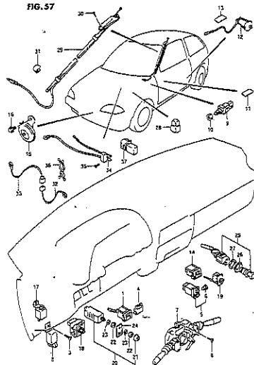
02-70 PARTES ELECTRICAS
