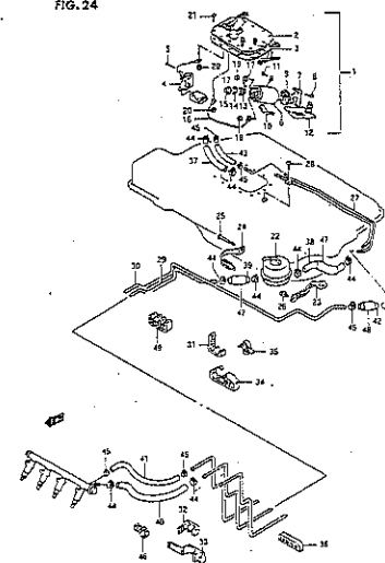
03-30 LINEAS COMBUSTIBLE
