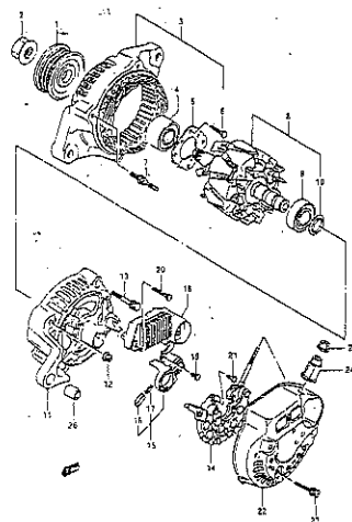
02-15 ALTERNADOR
