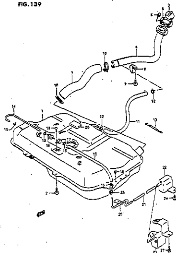
03-35 TANQUE COMBUSTIBLE
