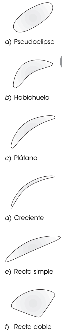
FIGURA 3-16 Parte 1 “Catálogo resumido” de formas de curva del acoplador
