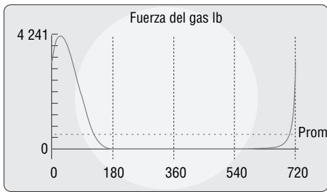
a) Ciclo Otto de cuatro tiempos
