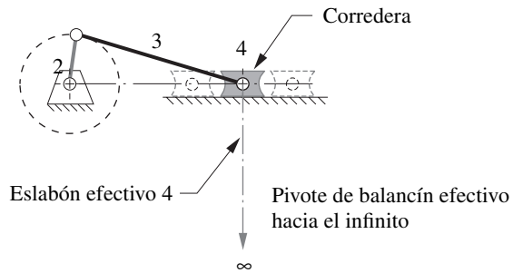
Manivela-corredera de Grashof
