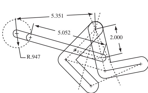
a) Una solución posible al problema 3-3
