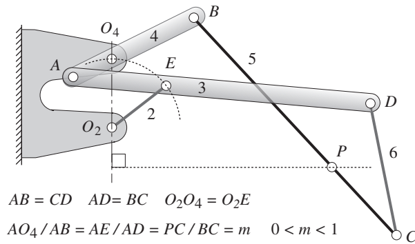
i) Mecanismo de línea recta exacta de Hart
