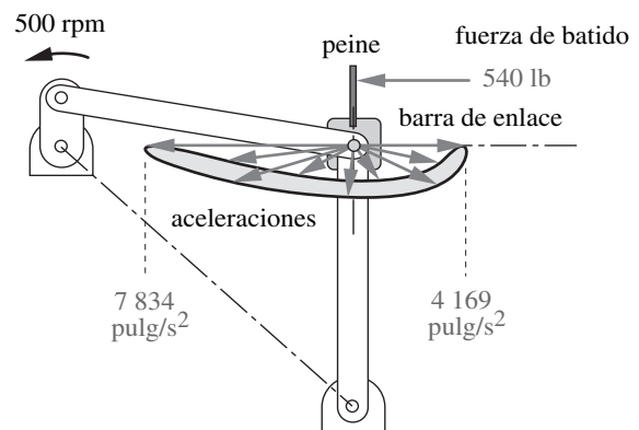
c) Aceleración en la barra de enlace y fuerza en el peine
