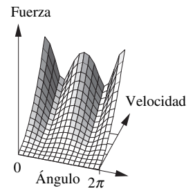
a) Fuerza de inercia del muñón de manivela
