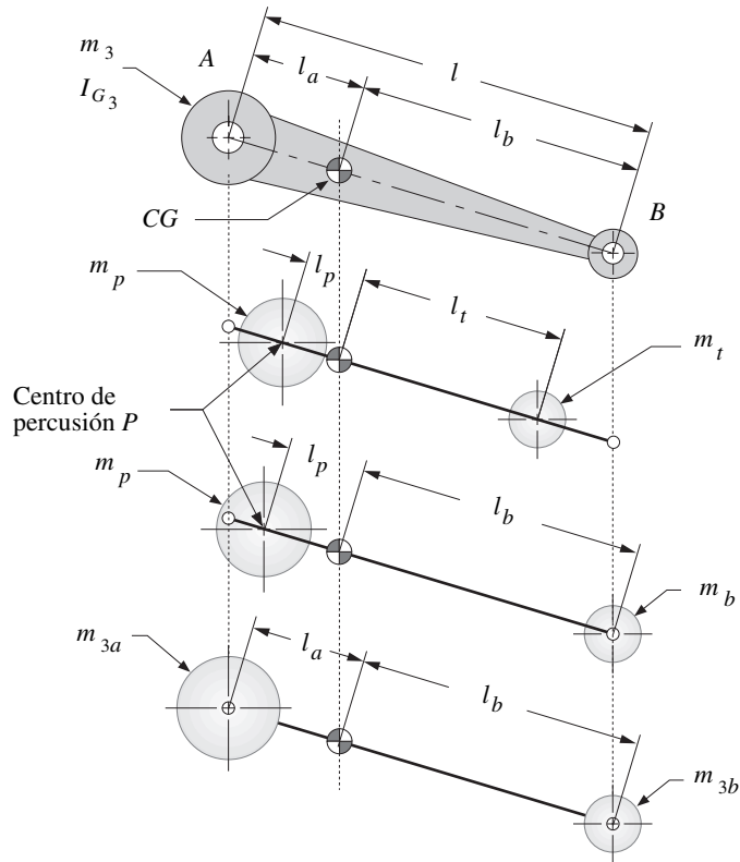
b) Modelo de dos masas genérico
