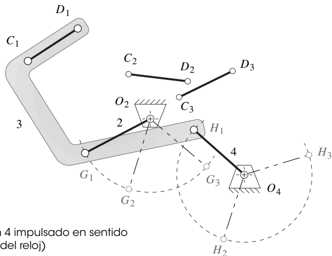
c) Reinversión para obtener el resultado d) Recolocación de la línea CD en el eslabón 3
