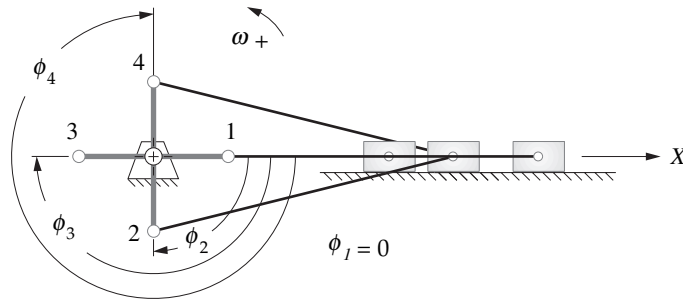
a) Ángulos de fase del cigüeñal
