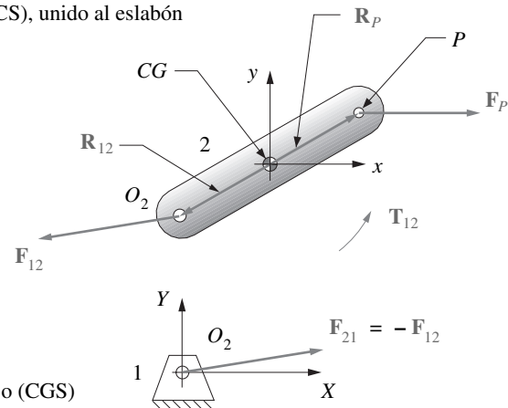
b) Diagramas de fuerzas (cuerpo libre)
