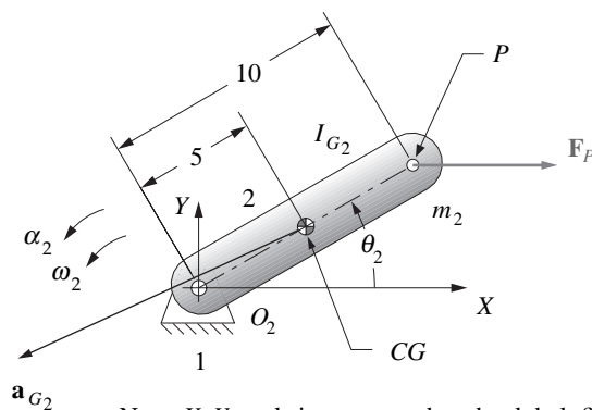
a) Diagrama cinemático
