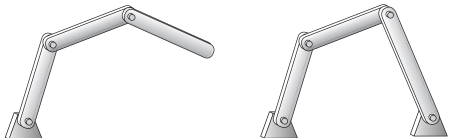
a) Mecanismo de cadena abierta
