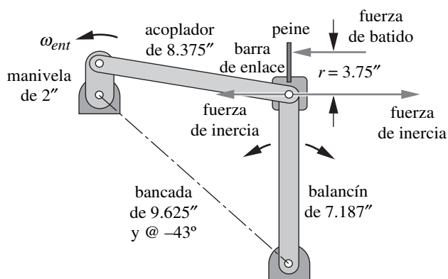
b) Mecanismo, barra de enlace, peine y dimensiones
