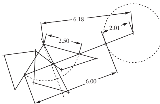
b) Una solución posible al problema 3-5
