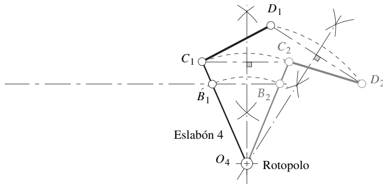
a) Localización del rotapolo en el ejemplo 3-2
