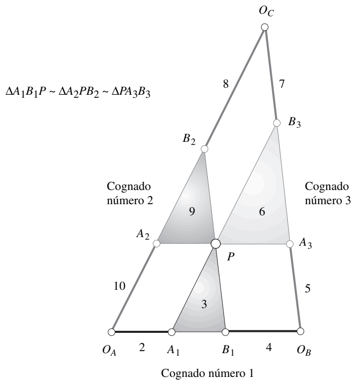
c) Trace líneas paralelas a todos los lados del mecanismo de cuatro barras original para crear cognados
