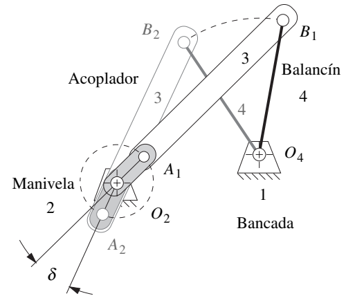
b) Mecanismo articulado terminado en sus dos posiciones de agarrotamiento
