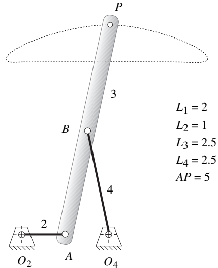
e) Mecanismo de línea recta de Hoeken
