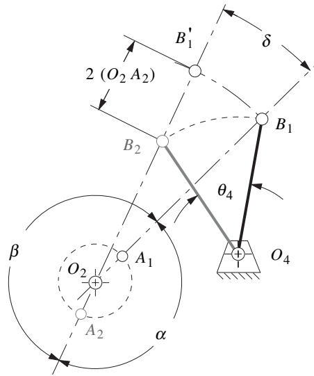
a) Construcción de un mecanismo balancín-manivela de Grashof de retorno rápido
