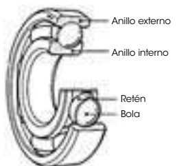
a) Cojinete de bolas
