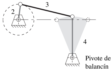
Manivela-balancín de Grashof
