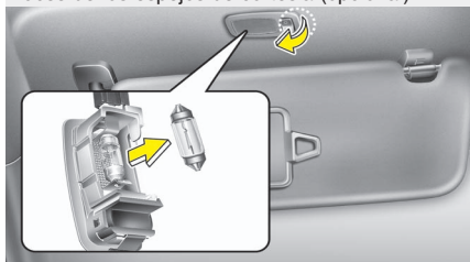
Luces de los espejos de cortesía (opcional)
