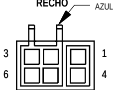
CONMUTADOR DE ELEVACIONAS ELECTRICAS DELANTERO DERECHO
