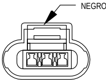
3 2 1 SENSOR DE POSICION DE LA MARIPOSA DEL ACELERADOR (2.0L)
