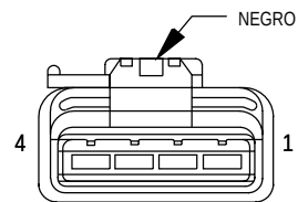
CONJUNTO DE MOTOR DE VENTILADOR DE RADIADOR
