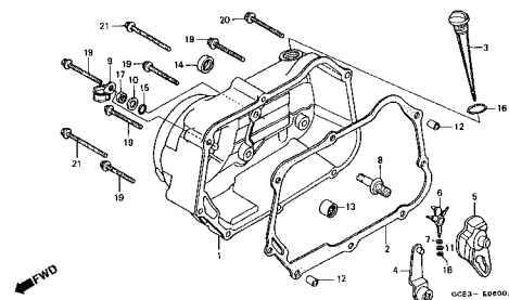
M-6 Tampa Direita da Carcaça / Right Crankcase Cover / Cubierta da Cáster Derecha de Motor
