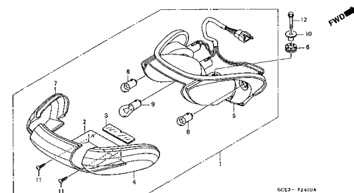
C-24 Lanterna Traseira • Sinalizador Traseiro / Rear Combination Light / Luz Intermitente Trasera
