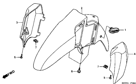
C-6.4 Pára-lama Dianteiro • Tampa do Pára-lama (+) / Front Fender • Front Cover (+) / Parafango Delantero • Tapa Parafango Delantero (+)
