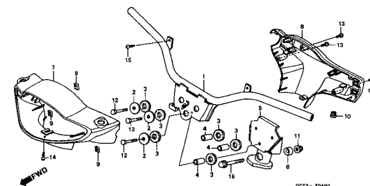
C-4.4 Guidão • Tampa do Guidão (+) / Steering Handle Cover (+) / Tubo de Manubrio • Tapa Tubo de Manubrio (+)
