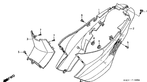
C-14.5 Carenagem Lateral / Body Cover / Cubretablero (ARGENTINA)
