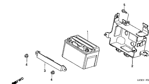
C-25.1 Bateria / Battery / Bateria (ARGENTINA)
