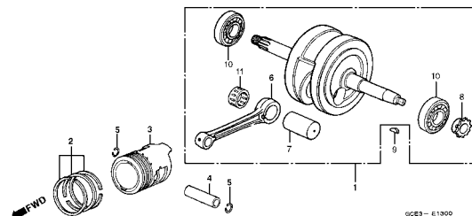
M-13 Árvore de Manivelas • Pistão / Crankshaft • Piston / Cigüenal • Pistón
