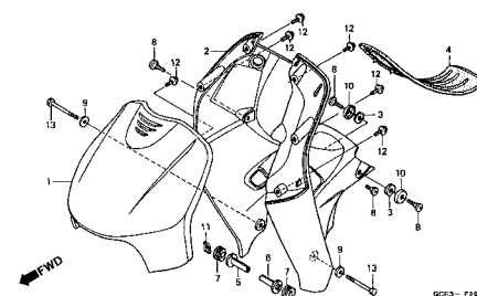
C-29.5 Tampa Dianteira • Protetor de Pernas (+) / Front Cover • Leg Shield (+) / Cubierta Delantera • Protector de Pernas (+)
