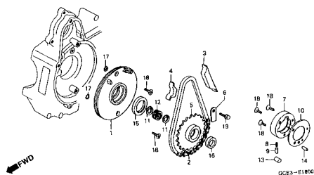
M-18 Embreagem de Partida / Starting Clutch / Embrague Arranque
