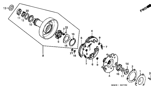
M-7 Embreagem Unidirecional / One Way Clutch / Sistema Embreague
