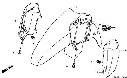
C-6.3 Pára-lama Dianteiro • Tampa do Pára-lama (+) / Front Fender • Front Cover (+) / Parafango Delantero • Tapa Parafango Delantero (+)
