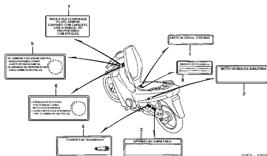
C-31.2 Emblemas (04) / Mark (04) / Franjas (04)
