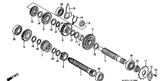
M-14 Transmissão / Transmission / Transmisión
