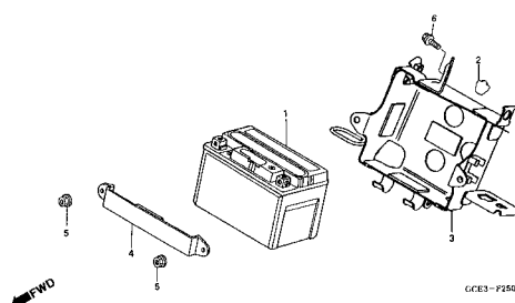
C-25 Bateria / Battery / Bateria
