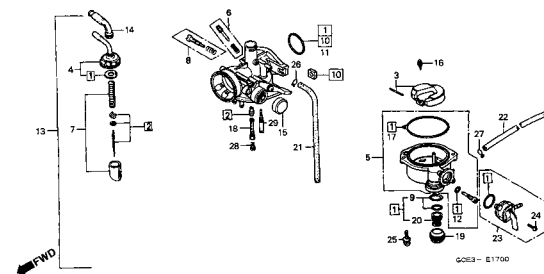
M-17 Carburador / Carburetor / Carburador
