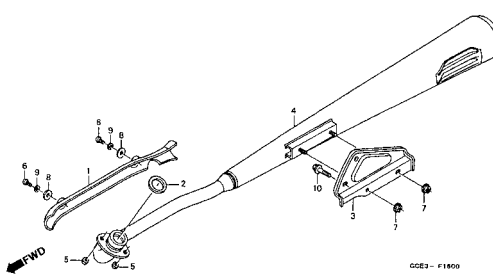
C-16 Escapamento / Exhaust Muffler / Silenciador de Escape
