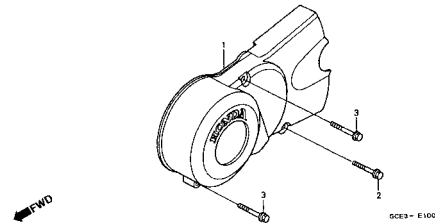
M-10 Tampa Lateral Esquerda do Motor / Left Crankcase Cover / Cubierta de Cáter Izquierda de Motor
