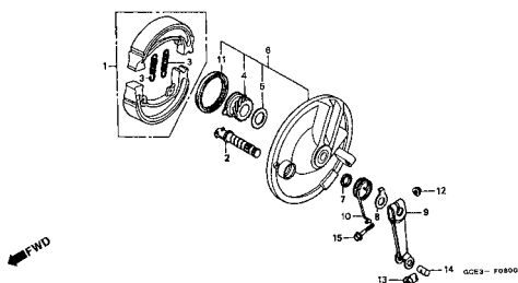
C-10 Espelho Freio Traseiro / Rear Brake Panel / Panel de Freno Trasero
