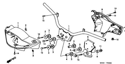
C-4.4 Guidão • Tampa do Guidão (+) / Steering Handle Cover (+) / Tubo de Manubrio • Tapa Tubo de Manubrio (+)
