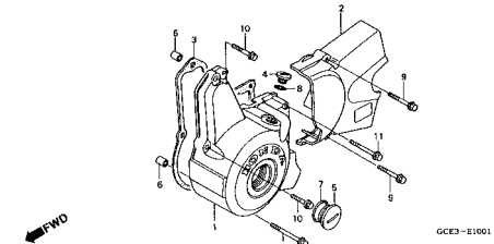
M-10.1 Tampa Lateral Esquerda do Motor / Left Crankcase Cover / Cubierta de Cáter Izquierda de Motor
