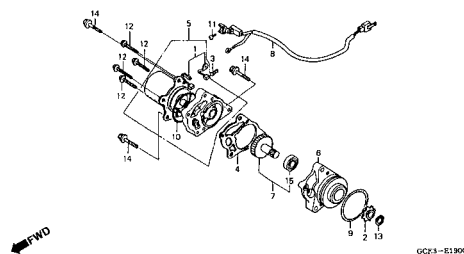
M-19 Motor de Partida / Starting Motor / Motor de Arranque
