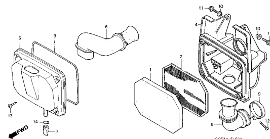
C-15 Filtro de Ar / Air Cleaner / Limpiador de Aire
