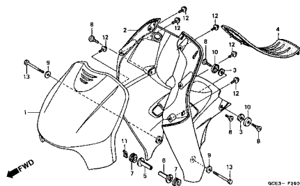
C-29.3 Tampa Dianteira • Protetor de Pernas (+) / Front Cover • Leg Shield (+) / Cubierta Delantera • Protector de Pernas (+)
