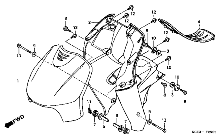
C-31.1 Emblemas (03) / Mark (03) / Franjas (03)
