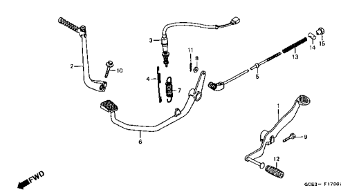
C-17 Pedal de Partida • Pedal de Freio / Kick Starter Arm • Pedal / Brazo Arranque de Pie • Pedal
