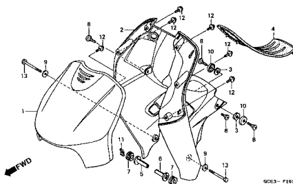
C-29.4 Tampa Dianteira • Protetor de Pernas (+) / Front Cover • Leg Shield (+) / Cubierta Delantera • Protector de Pernas (+)
