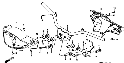
C-4.3 Guidão • Tampa do Guidão / Steering Handle Cover / Tubo de Manubrio • Tapa Tubo de Manubrio (ARGENTINA)
