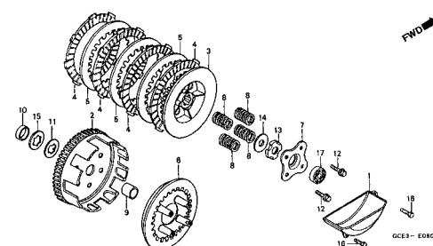
M-8 Embreagem / Clutch / Embrague
