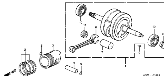
M-13.1 Árvore de Manivelas • Pistão / Crankshaft • Piston / Cigüenal • Pistón (ARGENTINA)
