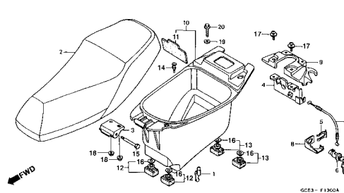
C-13 Assento • Caixa Interna / Seat • Luggage Box / Asiento • Guarda Documentos
