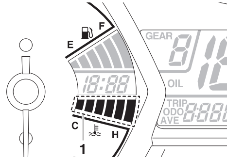
1. Indicador de temperatura del refrigerante
