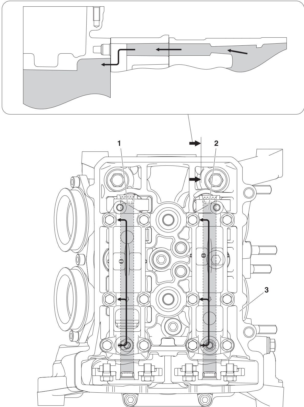
Eje de levas (vista superior)
