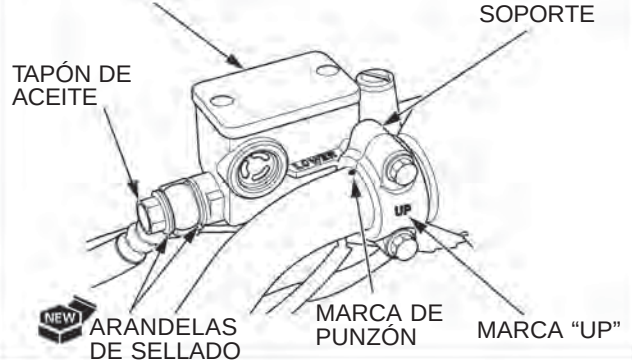
CILINDRO MAESTRO
