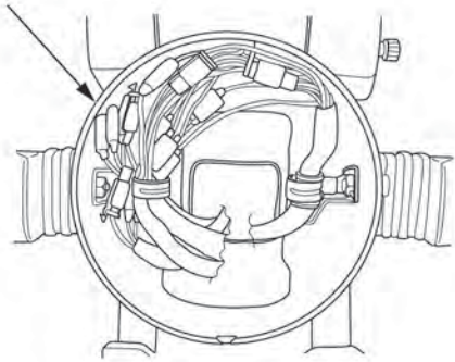
ALOJAMIENTO DEL FARO
