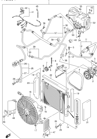
SN413V-5 E22_204 AIR CON SET (1)
