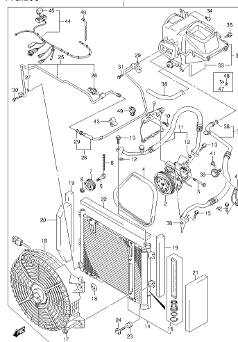
SN413V-5 E22_205 AIR CON SET (2)
