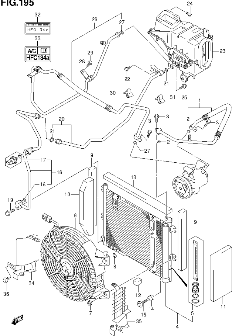
SN413V-5 E22_195 AIR CON PIPING (1)
