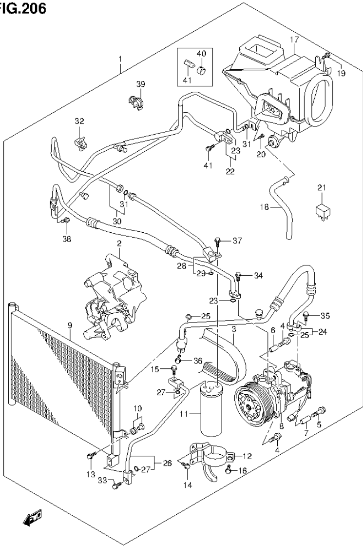
FIG.206 (4-K-2) AIR CON SET (SN415VD:OPT)
