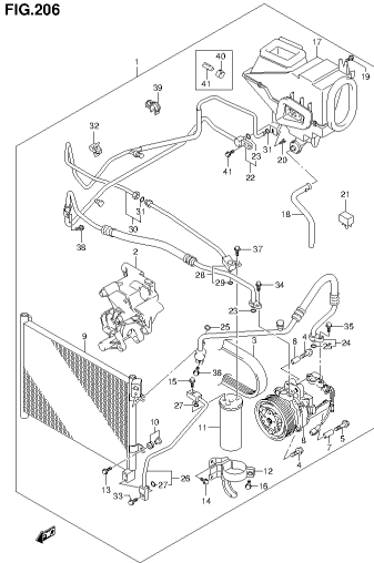
SN413V-5 E22_206 AIR CON SET (3)
